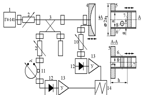
Рисунок 2 - Блок-схема экспериментальной установки
