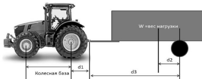
Рис. 2 – Розрахункова схема для визначення параметрів баластування
