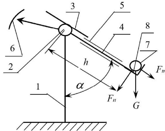
Рис. 1 – Калібрувальна схема вимірювача маси потоку дисперсних матеріалів: 1 – опора; 2 – поздовжня балка; 3 – компенсатор динамічних зусиль; 4 – тензовимірювальна площина; 5 – тензодатчик; 6 – механізм зміни кута нахилу тензовимірювальної площини; 7 – гирі; 8 – фіксована пластина для гир
