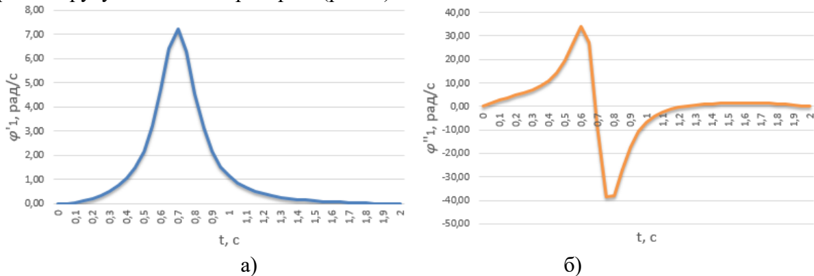
Рис.8. Графіки кутової швидкості (а) та пришвидшення (б) повороту руки робота при оптимальному ривковому режимі руху захвату
