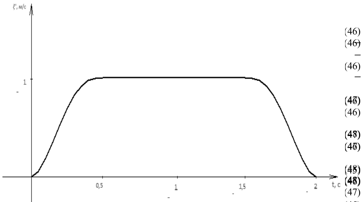
Рис. 9. Графік швидкості комплексного оптимального режиму руху захвату
