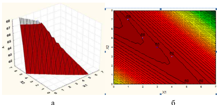
Рисунок 2 – Поверхня і лінії рівня параболічної залежності (а), лінії рівнів (б) для індексу деформації клейковини пшениці: x_1 – термін зберігання; x_2 – середня температура зерна в зернохвищі; Y – ІДК пшениці
