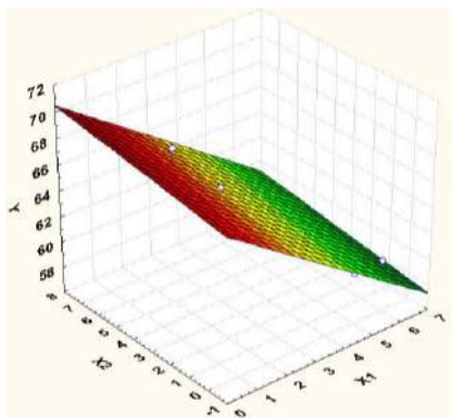
Рисунок 1 – Поверхня лінійної залежності для індексу деформації клейковини пшениці: x_1 – термін зберігання; x_2 – середня температура зерна в зернохвищі; Y – ІДК пшениці
