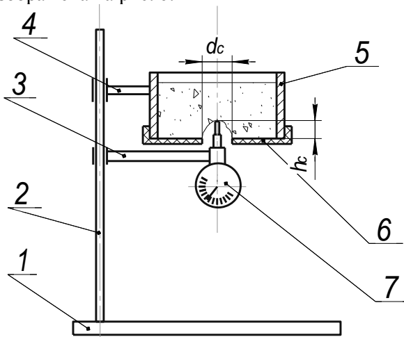
Рис. 6. Схема експериментальної установки для визначення висоти склепінень: 1 - платформа; 2 - стойка; 3, 4 - кронштейни; 5 - циліндрична ємність; 6 - еластична насадка; 7 - індикатор переміщення
