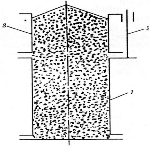
Рис. 1. Мірна посудина для визначення об'ємної щільності сипучих матеріалів: 1 – мірна посудина; 2 – вісь; 3 – обертова рамка
