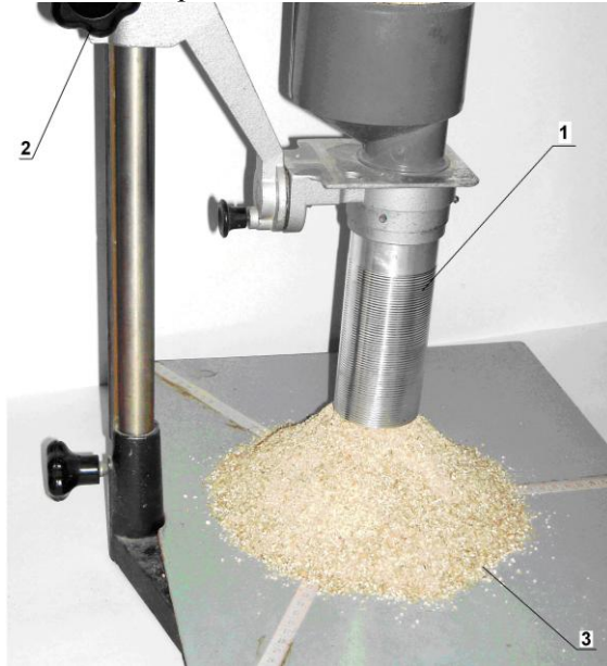
Рис. 3. Прилад для визначення кутів природного укосу сипучих матеріалів: 1 – порожнистий циліндр; 2 – механізм підймання циліндра; 3 – площина з розміткою
