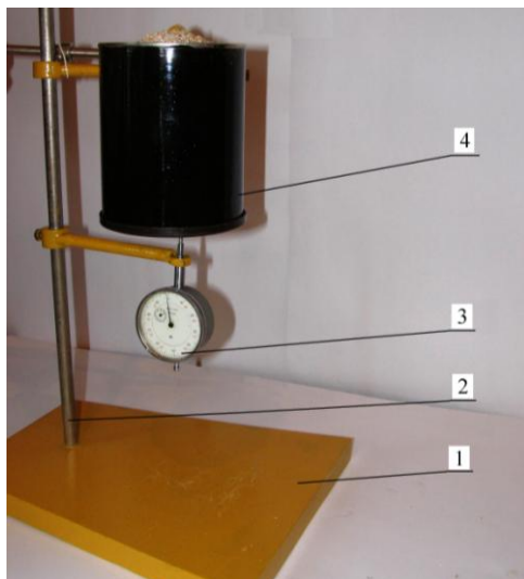
Рис. 7. Загальний вигляд установки для визначення виступу склепіння: 1 - платформа; 2 - стойка; 3 - індикатор переміщення; 4 - циліндрична ємність
