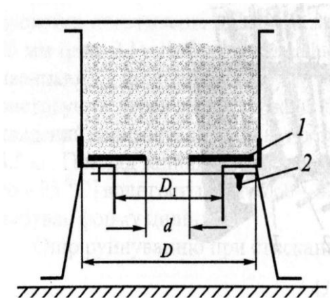
Рис. 4.Схема приладу для визначення критичного діаметра отвору склепінеутворення: 1 – діафрагма; 2 – заслінка
