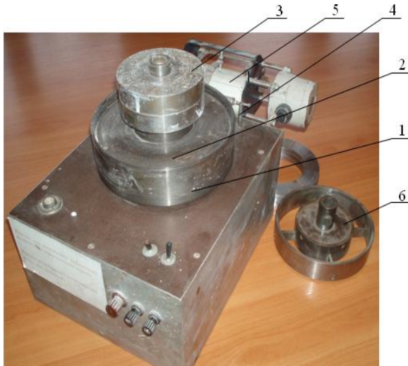
Рис. 2. Прилад для визначення коефіцієнтів зовнішнього і внутрішнього тертя сипучих матеріалів: 1 – бункер; 2 – рухомий диск; 3 – ваги; 4 – динамометричний пристрій; 5 – самописець; 6 – пристрій для зрушення сипучого матеріалу
