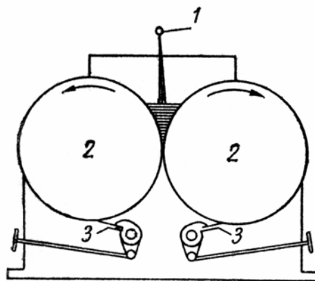
Рисунок 1.7 – Двовальцева сушарка: 1 – живлюча труба; 2 – барабани; 3 – ножі-скребки
