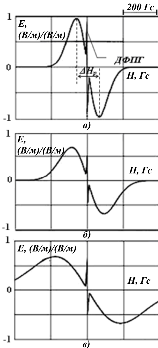
Рисунок 5.13 – Спектр полікристалічного порошку солі MnSO_4 (а) та зразків, що витримувались за відносної вологості 10 (б) та 80% (в)
