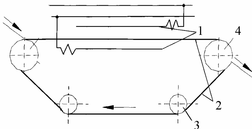
Рисунок 1.10 – НВЧ-сушарка: 1 – електроди; 2 – стрічка; 3 – підтримуючі ролики; 4 – ведучі ролики
