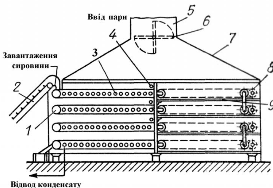
Рисунок 1.3 – Конвеєрна чотиристрічкова сушарка: 1 – ведучий барабан; 2 – похилий транспортер; 3 – калорифер; 4 – перегрібач; 5 – витяжна труба; 6 – шибер; 7 – витяжний ковпак; 8 – натяжний барабан; 9 – стрічкоочишувач
