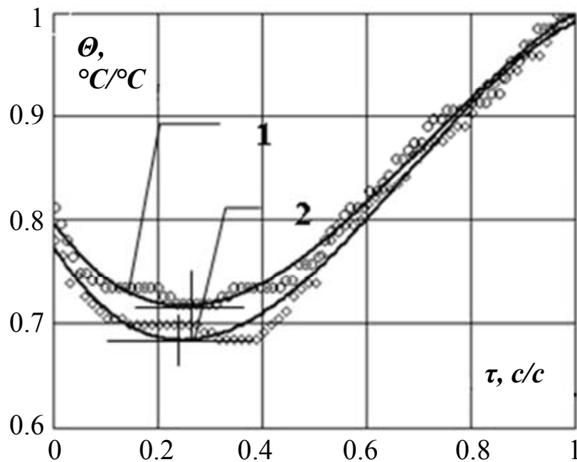
Рисунок 3.19 – Кінетика відносної температури об'єкта з високою теплопровідністю під час ЗТП-сушіння за умови температури сушильного агента, °С: 1 – 60; 2 – 75
