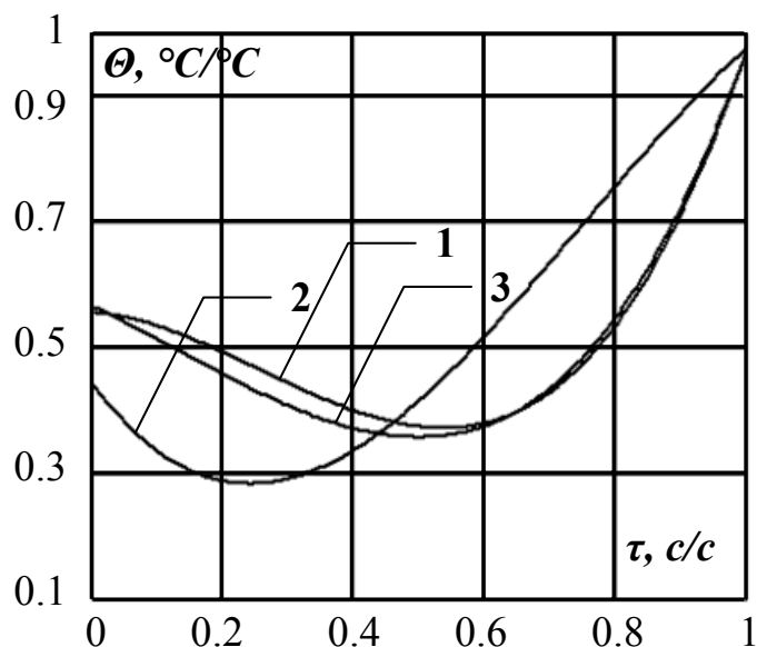
Рисунок 3.27 – Кінетика відносної температури під час ЗТП-сушіння зразків із щільністю, \text{кг/м}^3 : 1 – 330; 2 – 390; 3 – 540
