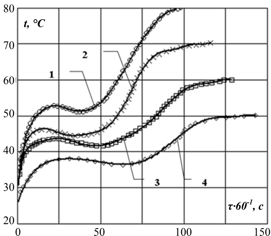
Рисунок 5.1 – Кінетика температури під час ЗТП-сушіння подрібненої плодово-ягідної сировини з КПТ за умови різної температури сушильного агента, ^\circ\text{C} : 1 – 80; 2 – 70; 3 – 60; 4 – 50
