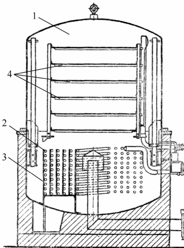
Рисунок 1.9 – Сублімаційна сушарка: 1 – сушильна шафа; 2 – конденсатор; 3 – скребки; 4 – лотки
