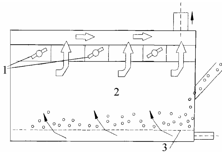
Рисунок 1.5 – Сушарка з ПЗШ: 1 – заслінки; 2 – сушильна камера; 3 – перфорована решітка
