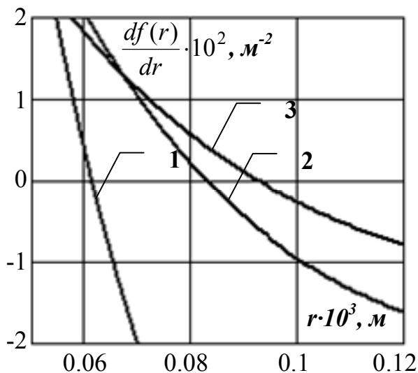
Рисунок 3.8 – Перша похідна від функції розподілу пухирчиків за радіусами для часу, що пройшов після збивання: 1 – \tau=0 с; 2 – \tau=1200 с; 3 – \tau=2400 с
