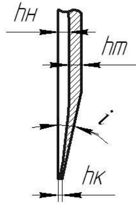
Рис. 1 – Зміна товщини несучого і твердого шару
