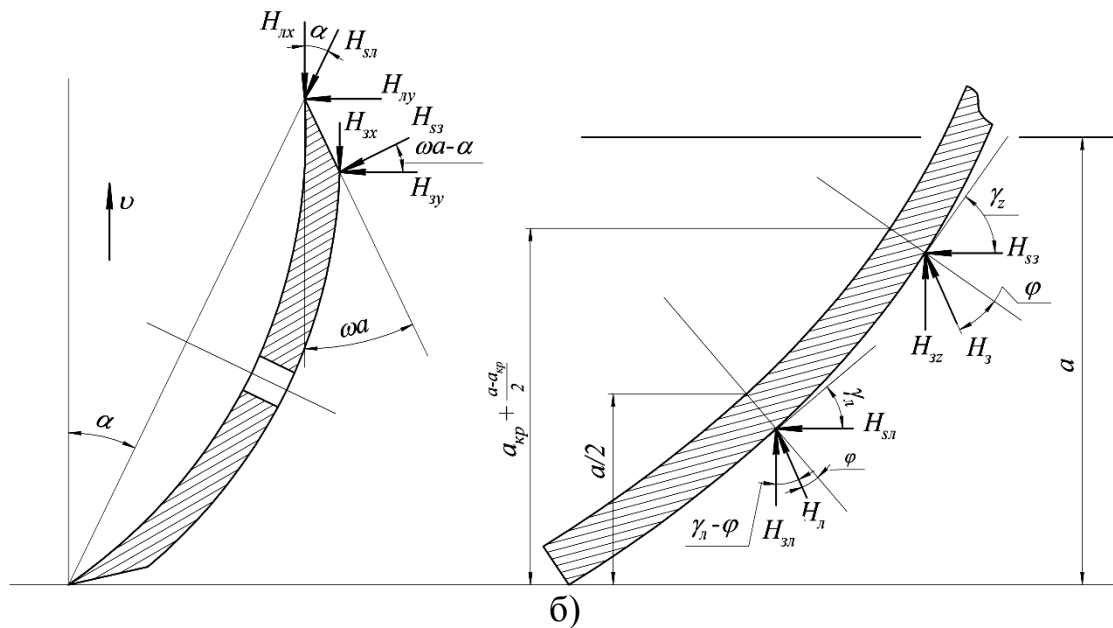
Рис. 2 – Сили що діють на внутрішню (а) і зовнішню (б) поверхню РО ДГЗ з зовнішнім загостренням.
