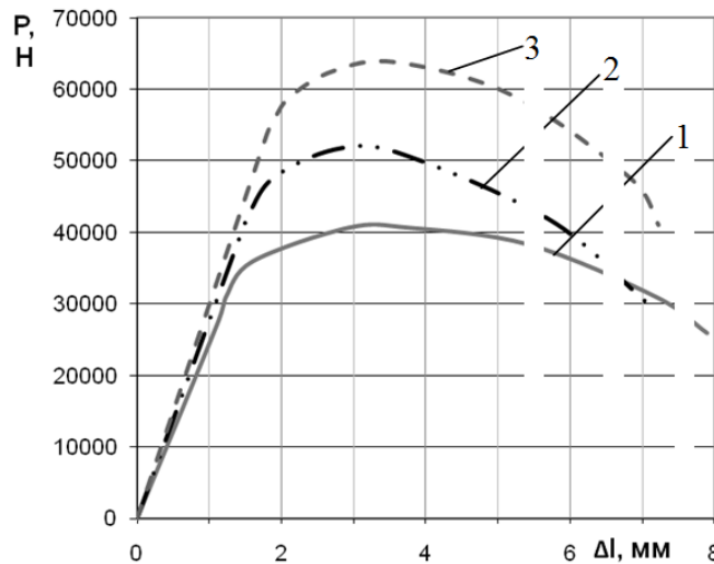
Рисунок 2 – Криві розтягання шатунних болтів у вихідному стані та після ІБ за двома режимами: 1 – вихідний стан; 2 – перший режим ІБ; 3 – другий режим ІБ
