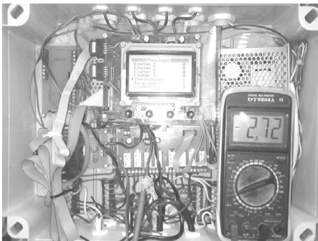
Рисунок 4 – Фрагмент апаратної реалізації інтелектуального блоку САУ очисткою стічних вод промислових об'єктів на базі контролера Atmega
