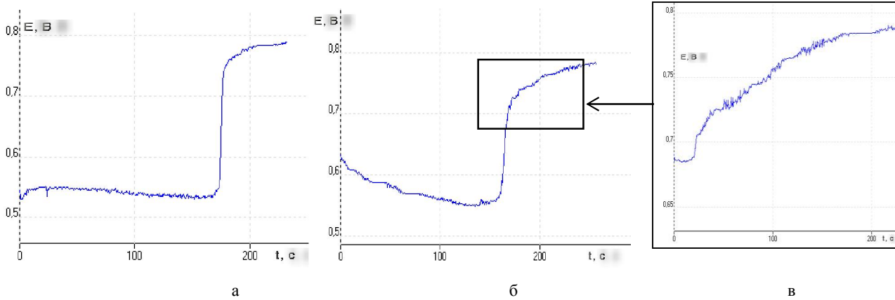
Рис. 2 – Криві кулонометричного титрування (залежність електрорушійної сили (E, В) від часу (t, c), скан з програми PicoLog Recorder): а – розчин АК з концентрацією 76,63 мкг/г (I=9,921 МА, m_p = 2,030 г); б – розчин АК з концентрацією 75,01 мкг/г в 3% розчині желатини (I=9,923 МА, m_p = 2,145 г); в – розчин 3% желатини (I=9,919, m_p = 4,140 г)
