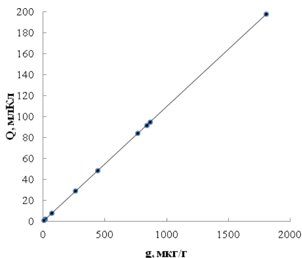
Рис. 1 – Залежність між вмістом АК (g, мкг) та кількістю електрики для електрогенерації титранту бром (Q, мЛкЛ) для модельних водних розчинів АК
