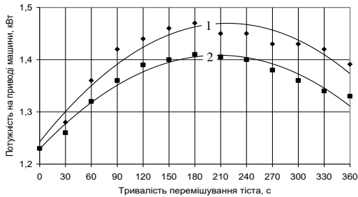
Рис. 2. Змінення потужності на приводі в процесі замісу при t_0 = 35\text{ }^\circ\text{C} : 1 – базовий місильний орган; 2 – новий місильний орган
