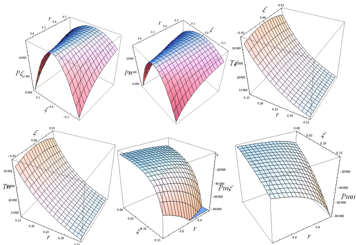
Рисунок 3 – Графики распределений давлений, построенные по точным выражениям и их разложением в ряды
