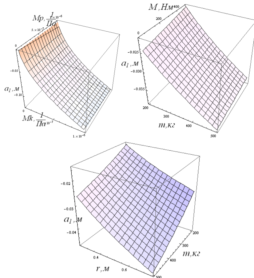
Рисунок 4 – Графики зависимости величины задней границы контакта от деформативных свойств колеса, приложенной к колесу массы, крутящего момента и радиуса колеса
