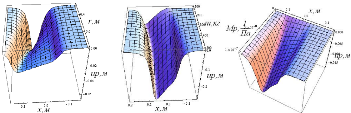
Рисунок 7 – Графики зависимости горизонтальной составляющей перемещений почвы в зоне контакта в зависимости от радиуса колеса r , массы m , приведенной к колесу, и деформативных свойств почвы M_p
