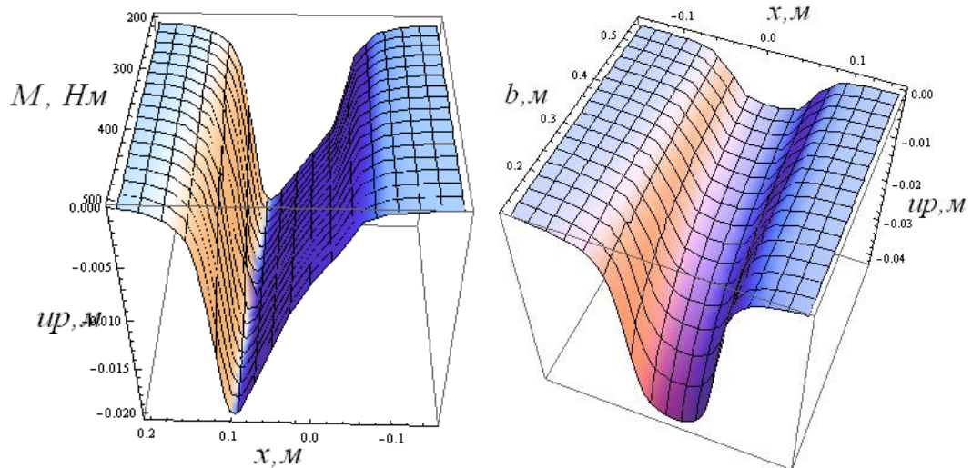
Рисунок 8 – Графики зависимости горизонтальной составляющей перемещений почвы в зоне контакта в зависимости от крутящего момента на колесе M и ширины колеса b
