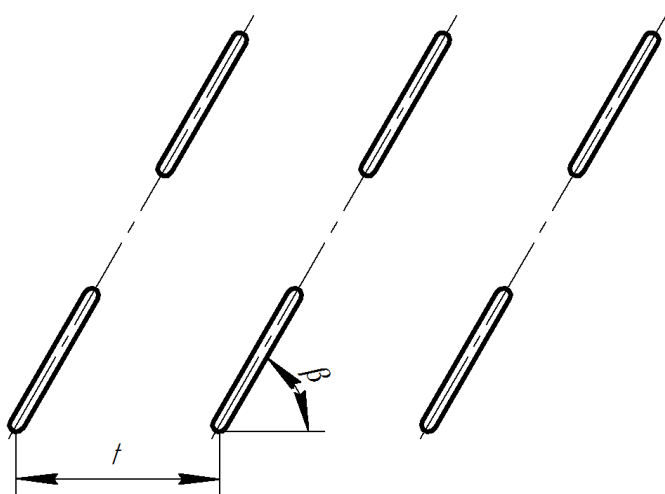
Рисунок 1 – Схема розташування гумових рифлів на поверхні труби шнека
