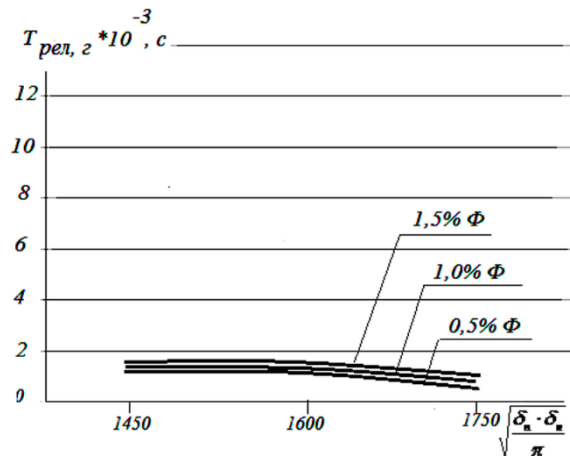
Рис.4. Залежності зміни часу релаксації структури гелю від внутрішнього тертя структури матеріалів трибоелементів і концентрації фулеренів ( \Phi )
