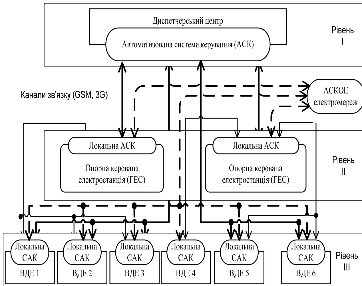
Рисунок 1 – Структурна схема АСК розосередженими джерелами енергії в електричних мережах
