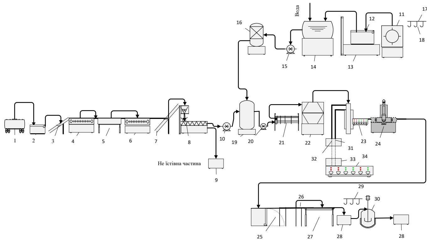
Рисунок А.33 – Апаративно-технологічна схема виробництва варення, джему та конфітюру:
