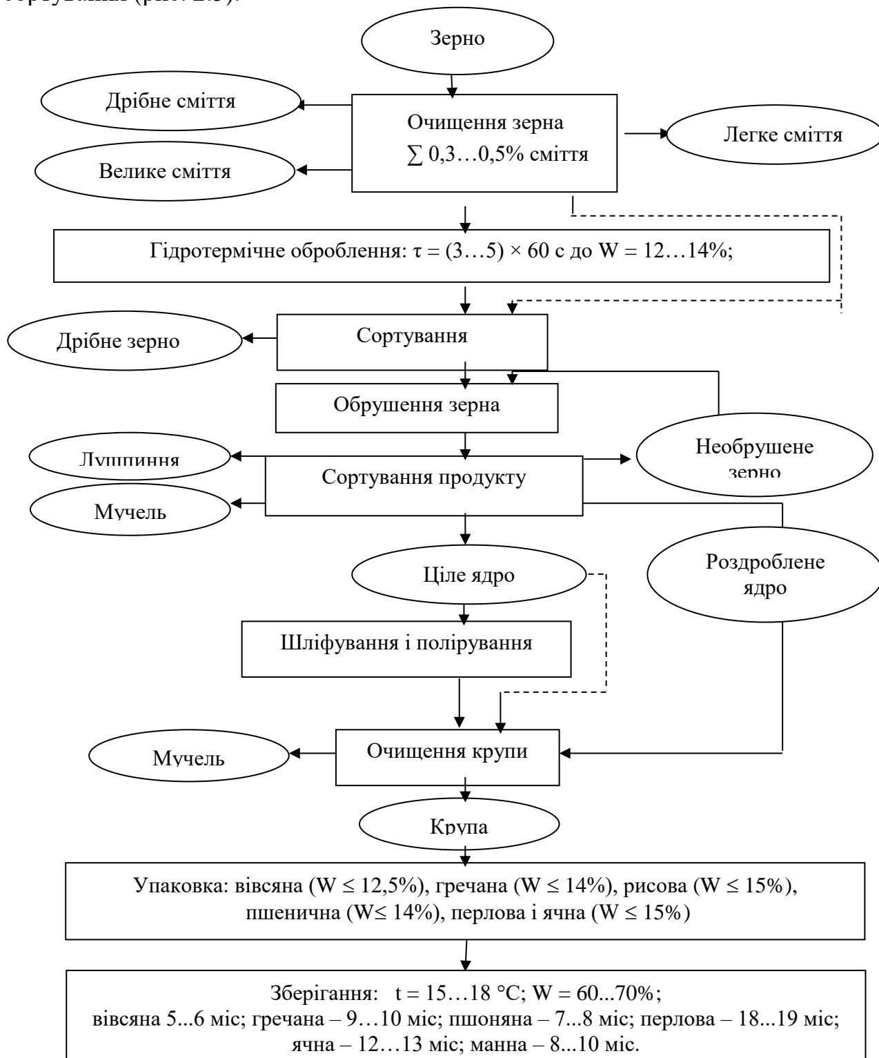
Рисунок 2.5 - Загальна технологічна схема отримання крупи
