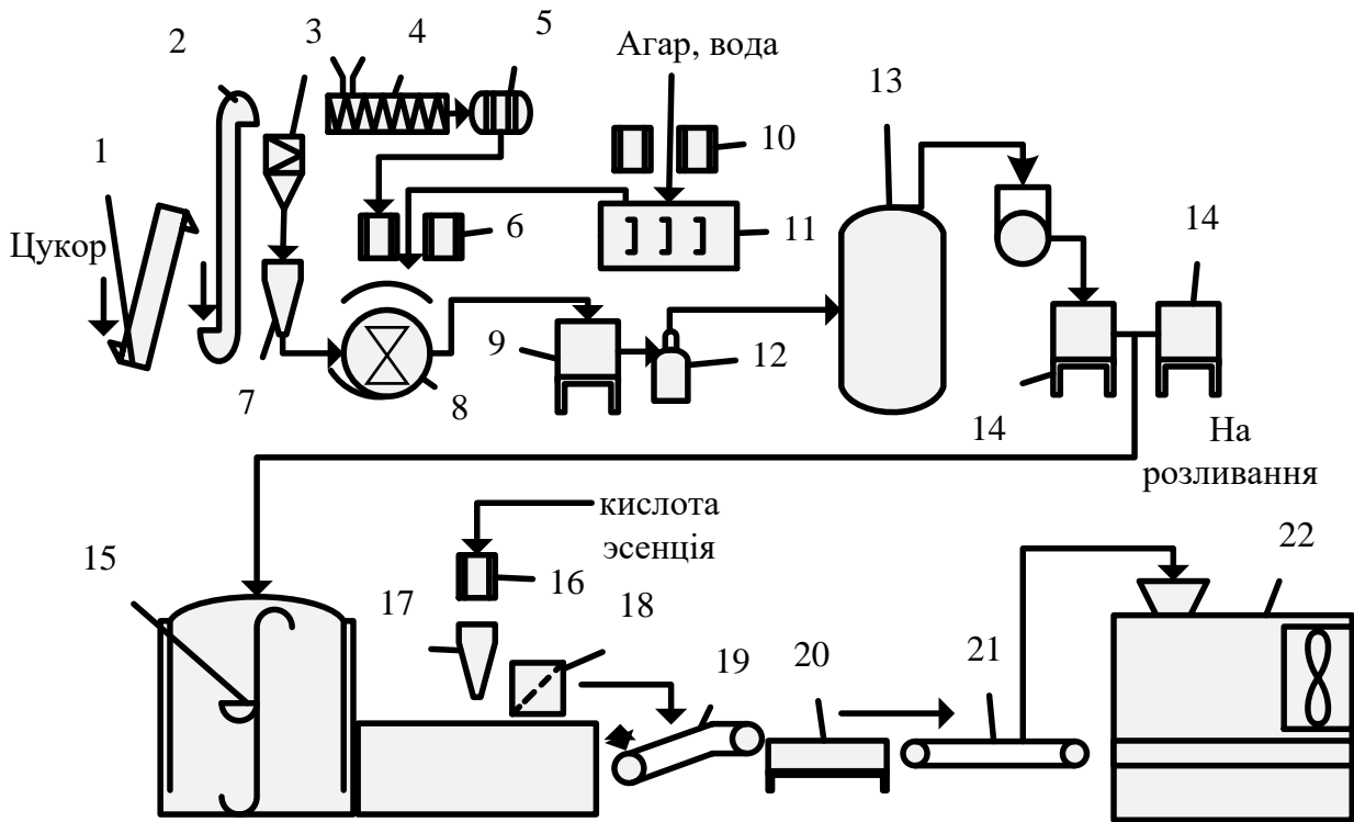
Рисунок А.3 – Апаратурно-технологічна схема виробництва желеїно-формового мармеладу на агарі: 1 – просіювач; 2 – норія; 3 – збірник-накопичувач; 4 – подрібнювач; 5 – сито; 6, 10, 16 – дозатори об'ємні; 7 – ваги автоматичні; 8 – котел із мішалкою; 9, 14 – ємності проміжні; 11 – пектинорозчиняльник; 12 – плунжерний насос дозатор; 13 – апарат змійовиковий варильний; 15 – апарат для відливання; 17 – змішувач; 18 – бункер відливної машини; 19 – система конвеєрів; 20 – барабан; 21 – конвеєр; 22 – автомат для охолодження
