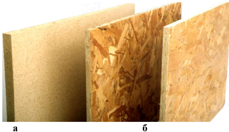
Рисунок 3.11 – Види плит: а – ДСП, б – МДФ
