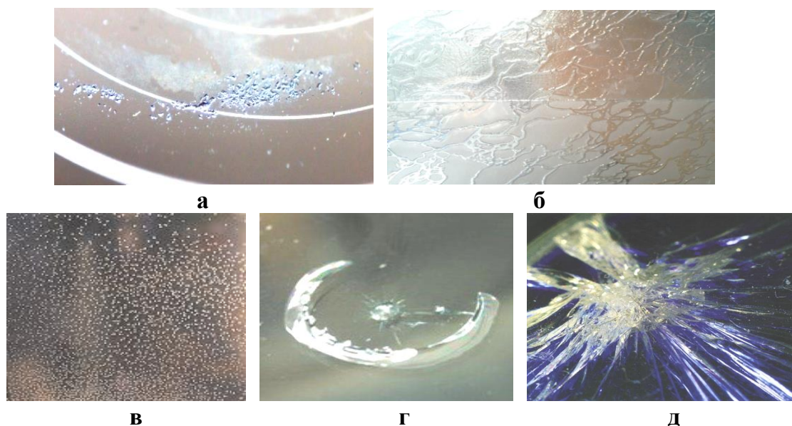
Рисунок 1.20 – Види дефектів скляних виробів: а – недопресовка; б – засорка в – мошка; г – шлір; д – свіль
