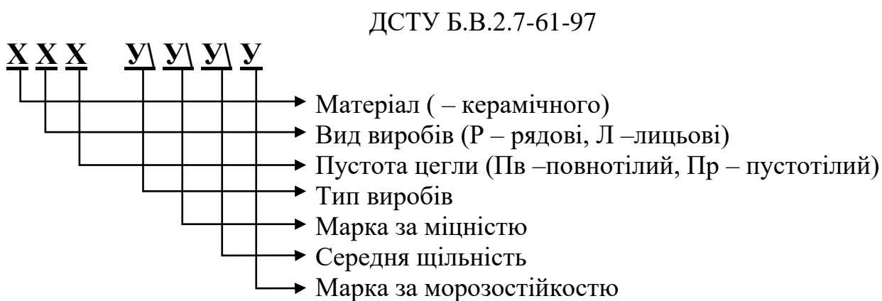
Рисунок 3.6 – Розшифрування позначок на маркуванні цегли
