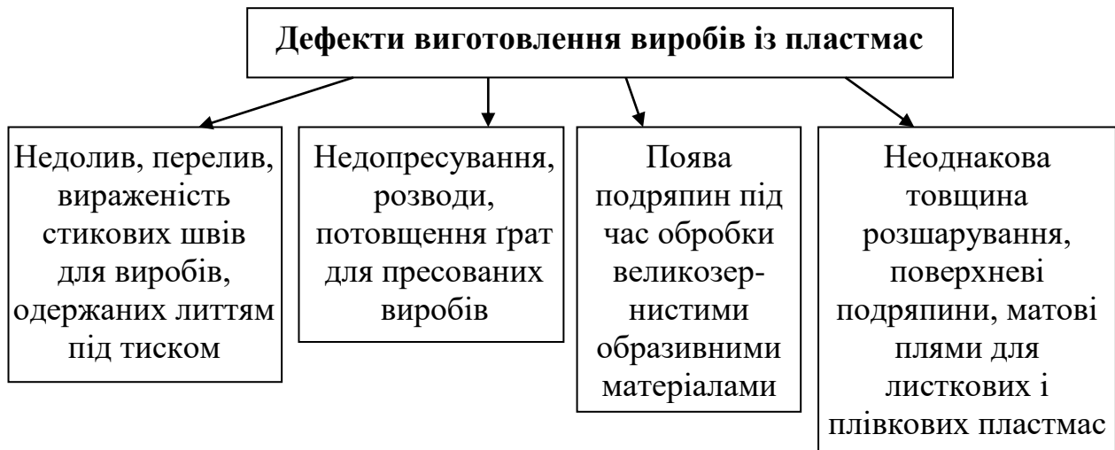
Рисунок 1.10 Дефекти виготовлення виробів із пластмас
