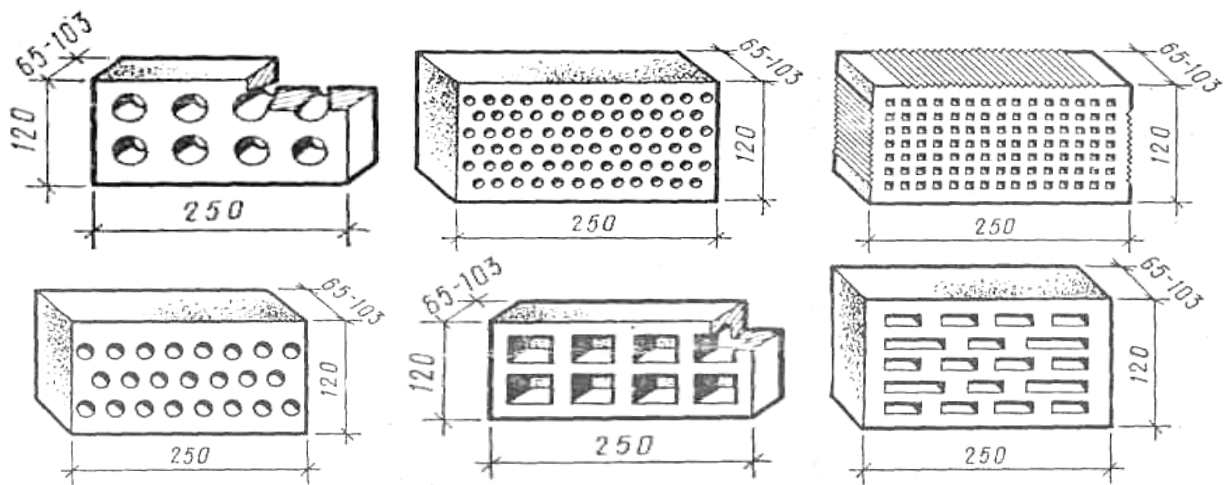
Рисунок 3.3 – Різновиди пустотілої цегли
