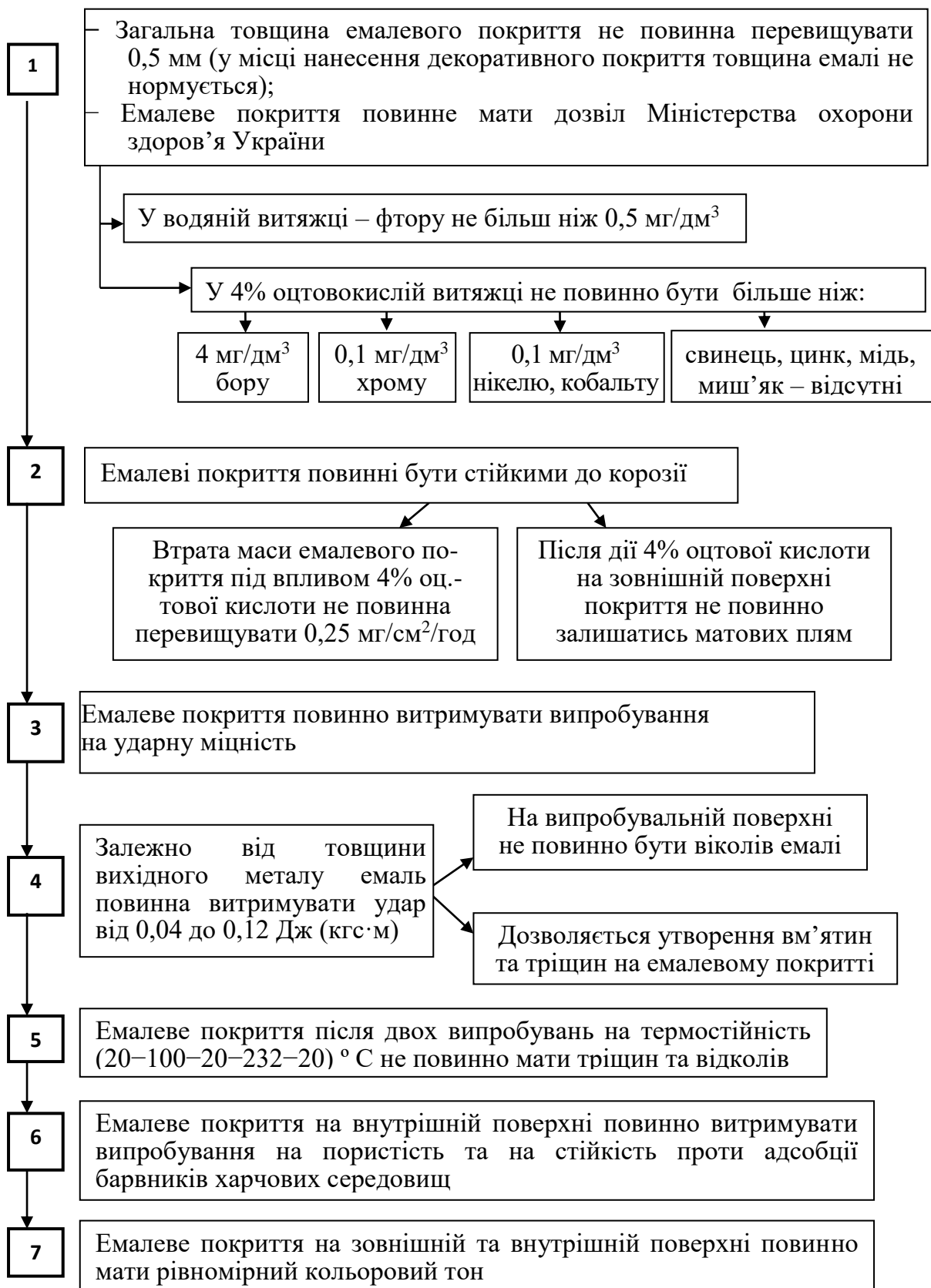
Рисунок 1.65 – Вимоги до механічної та хімічної стійкості емалевого покриття побутового посуду
