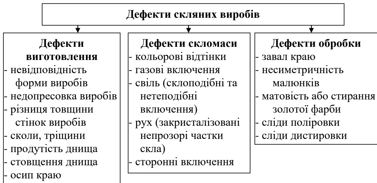
Рисунок 1.19 – Дефекти скляних виробів
