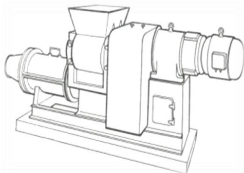
Рисунок 1.33 – Глиномішалка
