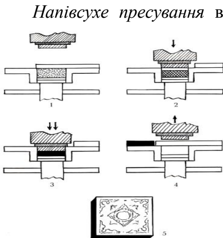
Рисунок 1.37 – Стадії пресування виробів
