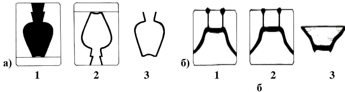
Рисунок 1.36 – Способи лиття виробів: а – наливний, б – зливний; 1 – форма, заповнена ливарним шлікером; 2 – підсушка відлитих виробів; 3 – виріб, вилучений із форми
