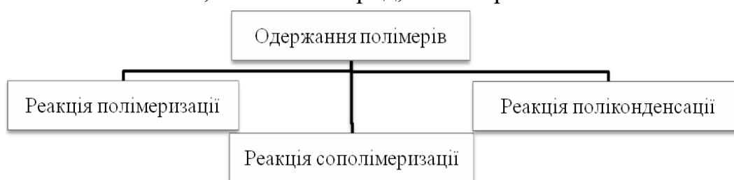
Рисунок 1.2 – Одержання полімерів
