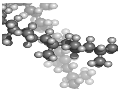
Рисунок 1.1 – Будова полімеру
