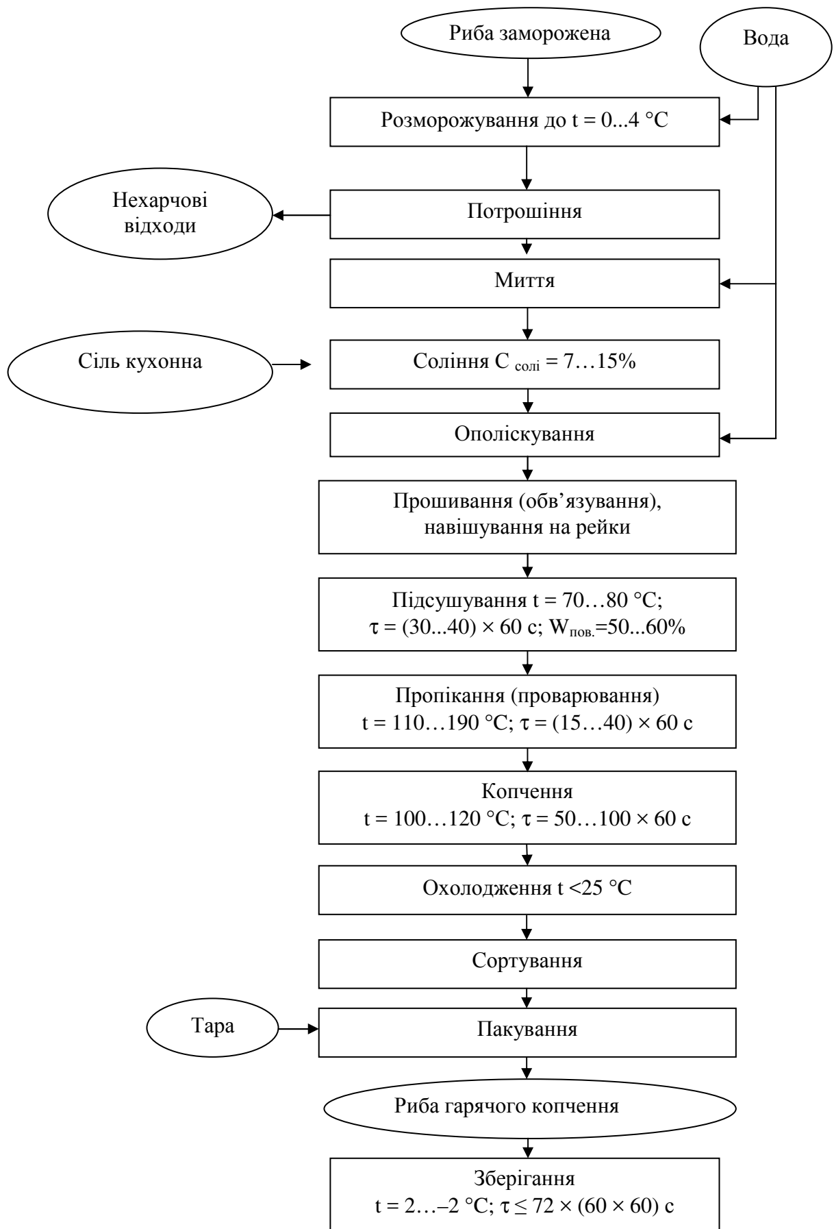
Рисунок 4.11 – Технологічна схема виробництва риби гарячого копчення
