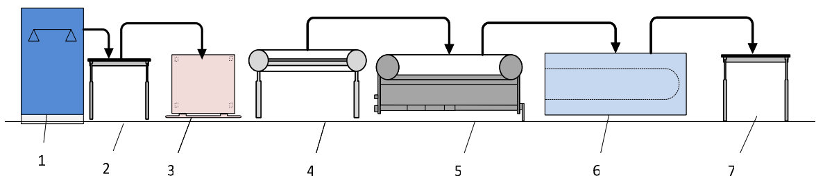
Рисунок 1.26 – Апаратурно-технологічна схема напівфабрикатів натуральних з яловичини, свинини та баранини за кулінарним призначенням: 1 – камера охолодження; 2 – стіл для обвалювання; 3 – візок; 4 – стіл для формування напівфабрикатів; 5 – машина пакувальна; 6 – камера швидкої заморозки; 7 – стіл для контролю якості
