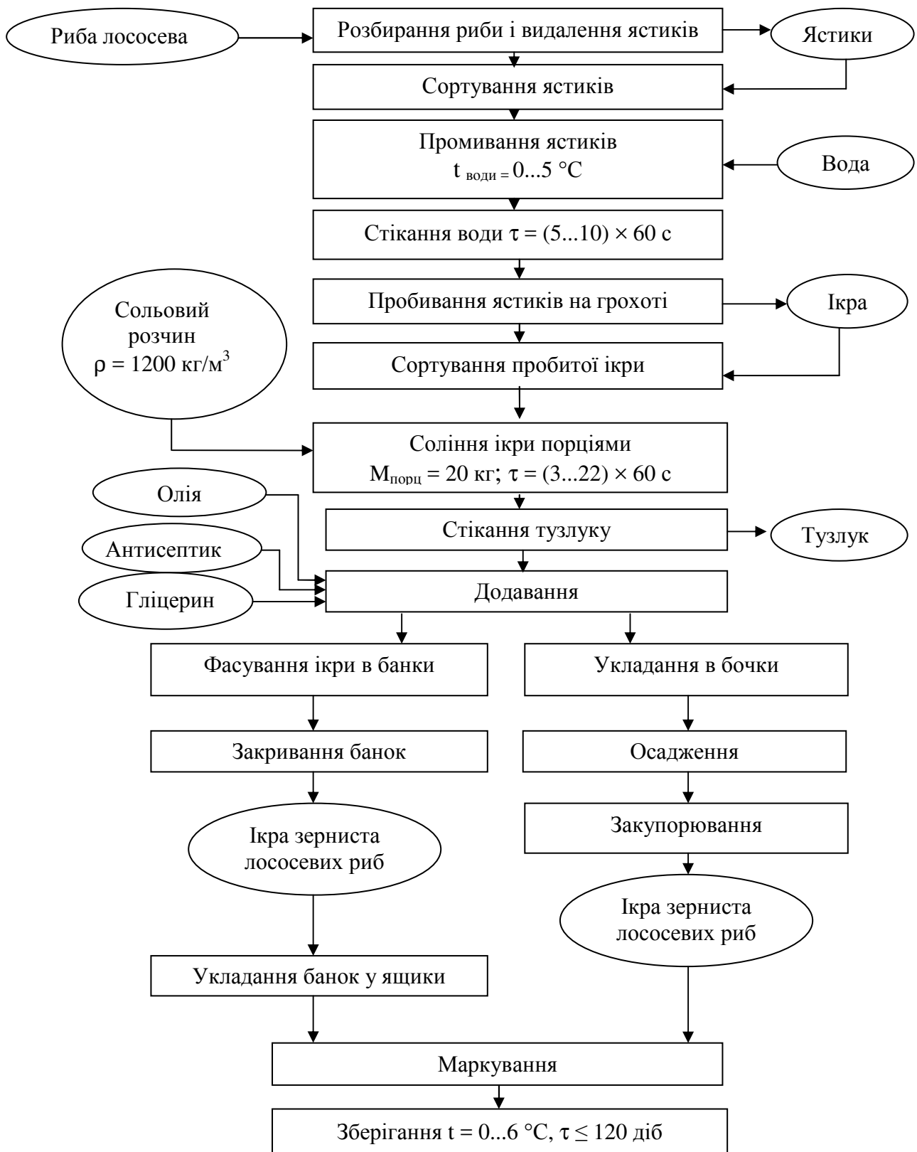
Рисунок 4.21 – Технологічна схема виробництва зернистої ікри лососевих риб
