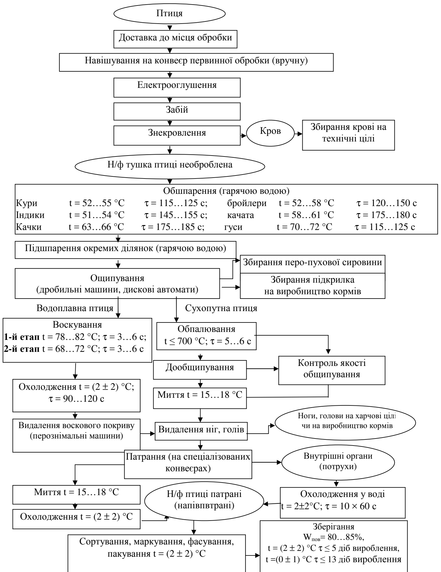
Рисунок 2.2 – Технологічна схема переробки птиці
