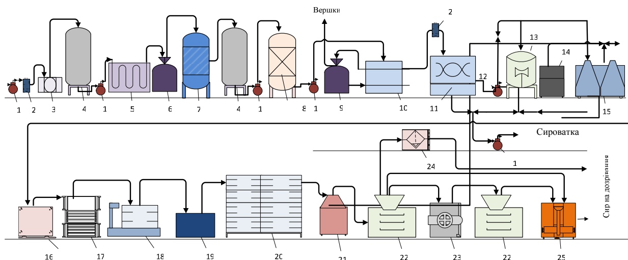
Рисунок 3.28 – Апаратурно-технологічна схема сичугових сирів: 1 – насос; 2 – лічильники-витратоміри; 3 – фільтр; 4 – резервуар для зберігання молока; 5 – теплообмінник пластинчастий; 6 – сепаратор-молокоочисник; 7 – охолоджувач пластинчастий; 8 – бак зрівняльний; 9 – сепаратор-вершковіддільник; 10 – установка пастеризаційно-охолоджувальна; 11 – ванна сироробна; 12 – насос; 13 – віддільник сироватки; 14 – форми підготовчі; 15 – апарат формувальний; 16 – візок для самопресування; 17 – преси; 18 – стелажі пересувні; 19 – етажер солильний; 20 – камера для дозрівання сиру; 21 – машина для миття сиру; 22 – машини для сушіння сиру; 23 – машина для нанесення латексного покриття на сир; 24 – машина вакуумпакувальна; 25 – парафінер
