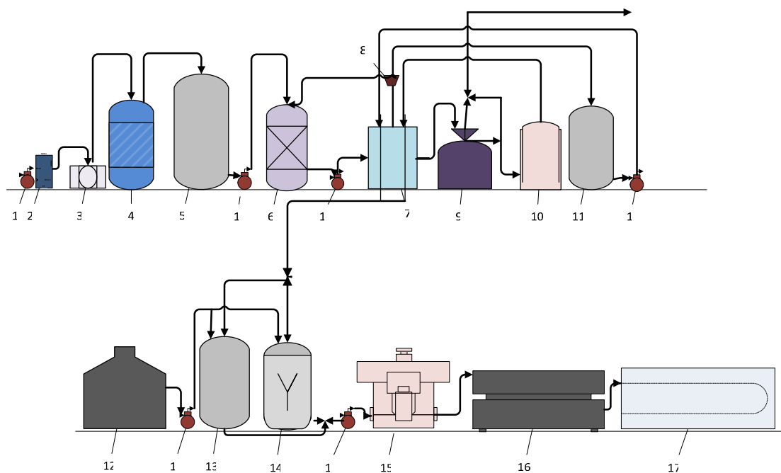
Рисунок 3.10 – Апаратурно-технологічна схема кисломолочних напоїв термостатним методом: 1 – насос; 2 – лічильник; 3 – фільтр; 4 – охолоджувач; 5 – резервуар проміжний; 6 – бачок зрівняльний; 7 – установка пастеризаційно-охолоджувальна; 8 – клапан зворотний; 9 – сепаратор-вершковіддільник; 10 – гомогенізатор; 11 – резервуар проміжний; 12 – ємність для закваски; 13 – резервуар для витримки суміші; 14 – апарат для сквашування; 15 – машина для пакування; 16 – камера термостатна; 17 – камера холодильна
