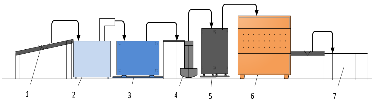
Рисунок 4.25 – Апаратурно-технологічна схема риби сушеної: 1 – транспортер подачі риби; 2 – машина для миття риби; 3 – чан для відмочування риби; 4 – машина для нанизування; 5 – рама; 6 – тунель для сушіння риби; 7 – стіл
