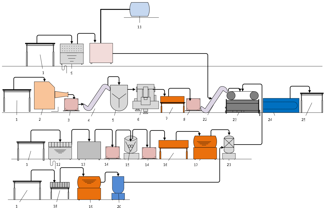
Рисунок 1.27 – Апаратурно-технологічна схема швидкозаморожених страв готових: 1 – стіл; 2 – вовчок; 3 – візок; 4 – підйомник; 5 – фаршмішалка; 6 – автомат для формування м'ясних напівфабрикатів; 7 – апарат для смаження; 8 – візок; 9 – машина для миття круп; 10 – апарат для варіння каш; 11 – ємність для води; 12 – апарат для миття овочів; 13 – машина для очищення овочів; 14 – візок; 15 – подрібнювач овочів; 16 – апарат для пасерування; 17 – котел для варіння соусу; 18 – стіл для обробки кісток; 19 – котел для варіння бульйону; 20 – ємність для охолодження бульйону; 21 – гомогенізатор; 22 – підйомник; 23 – машина фасувальна; 24 – камера швидкої заморозки; 25 – стіл
