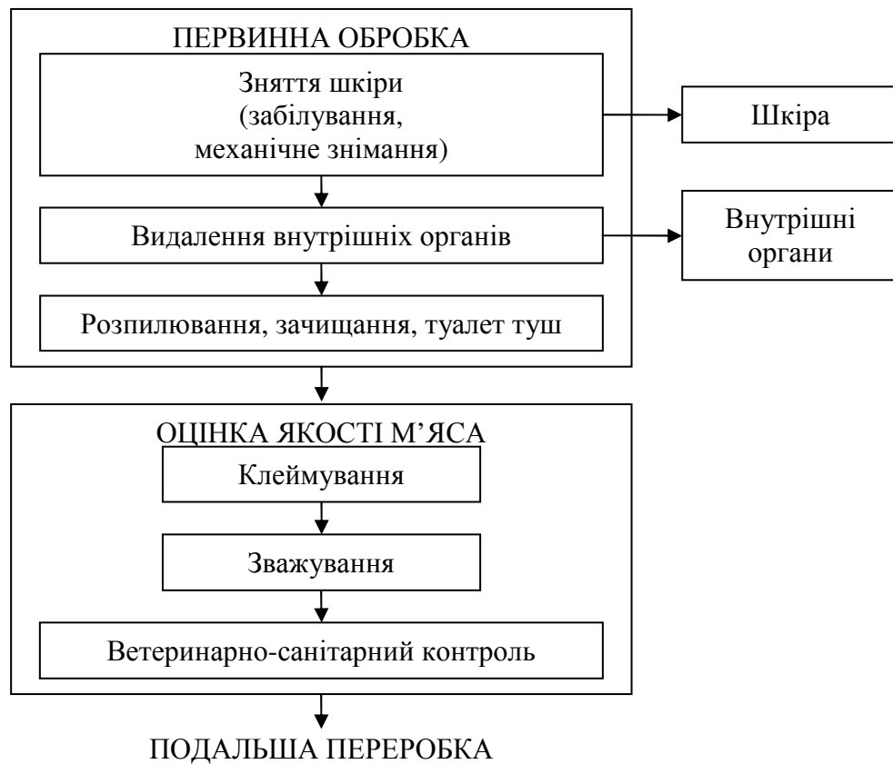
Рисунок 1.7 – Принципова схема первинної переробки туш забійних тварин
