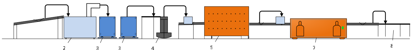
Рисунок 4.13 – Апаратурно-технологічна схема риби холодного копчення: 1 – транспортер подачі риби; 2 – машина для миття риби; 3 – чан для відмочування риби; 4 – машина для нанизування; 5 – кліматична установка для в'ялення риби з повним контролем технологічного процесу за заданими в систему управління програмами користувача; 6 – димогенератор; 7 – камера копильна тунельного типу; 8 – стіл
