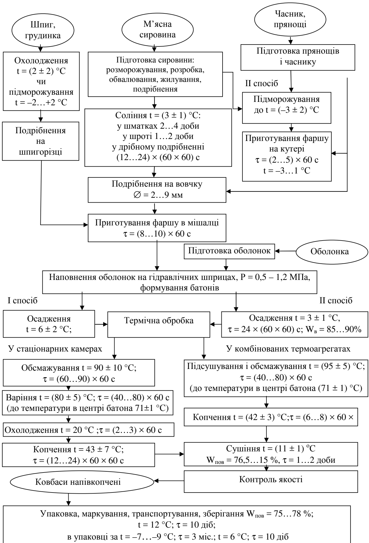
Рисунок 1.11 – Технологічна схема виробництва напівкопчених ковбас
