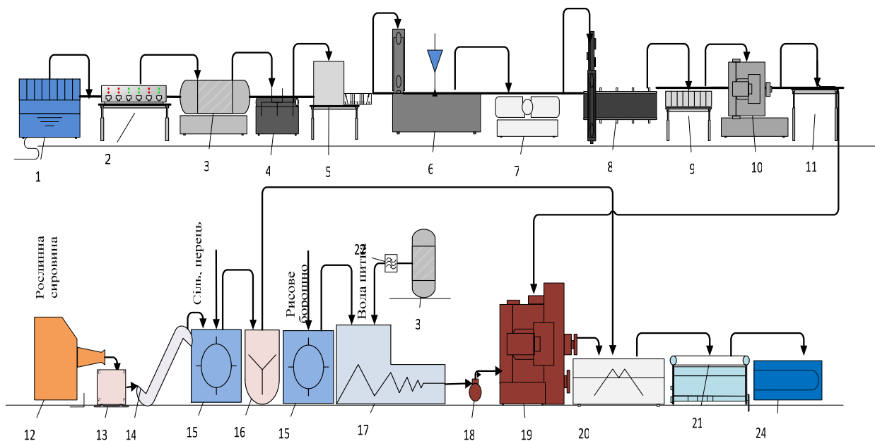
Рисунок 4.23 – Апаратурно-технологічна схема напівфабрикатів високого ступеня готовності з риби з використанням панірувань на основі рослинної сировини: 1 – дефростер водяний; 2 – конвеєр стрічковий; 3 – машина для зняття луски; 4 – машина для відділення плавників; 5 – машина для видалення голів риби; 6 – універсальний пристрій для переробки риби; 7 – машина для видалення хребетних і ребрових кісток; 8 – машина для зняття шкіри; 9 – конвеєр для інспекції; 10 – апарат для виробництва н/ф; 11 – стіл; 12 – подрібнювач; 13 – візок; 14 – підйомник; 15 – просіювач; 16 – змішувач; 17 – змішувач для приготування кляру; 18 – насос; 19 – ємність для кляру; 20 – ємність для панірування; 21 – конвеєр; 22 – фільтр для води; 23 – камера швидкої заморозки
