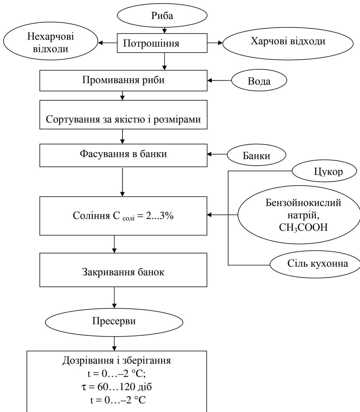
Рисунок 4.18 – Технологічна схема виробництва пресервів із риби
