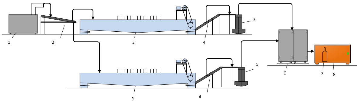
Рисунок 4.12 – Апаратурно-технологічна схема риби гарячого копчення: 1 – мийна машина; 2 – машина сортувальна; 3 – ванни механізовані для засолу; 4 – транспортери; 5 – машина нанизувальна; 6 – рама; 7 – димогенератор; 8 – камера копильна
