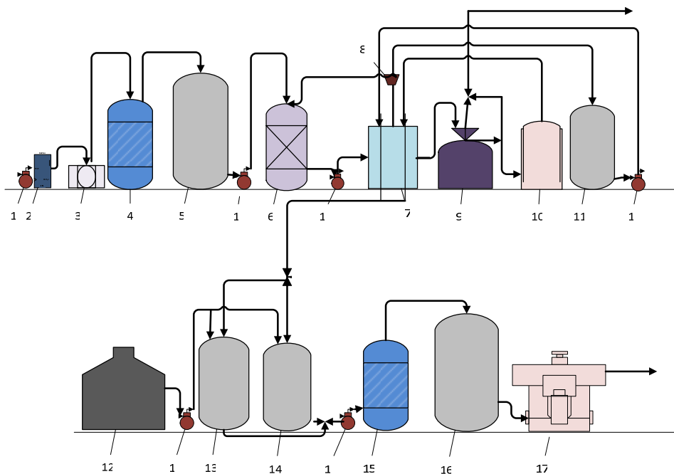
Рисунок 3.9 – Апаратурно-технологічна схема кисломолочних напоїв резервуарним методом: 1 – насос; 2 – лічильник; 3 – фільтр; 4 – охолоджувач; 5 – резервуар проміжний; 6 – бачок зрівняльний; 7 – установка пастеризаційно-охолоджувальна; 8 – клапан зворотний; 9 – сепаратор-вершковіддільник; 10 – гомогенізатор; 11 – резервуар проміжний; 12 – ємність для закваски; 13 – резервуар для витримки суміші; 14 – апарат для сквашування; 15 – охолоджувач; 16 – резервуар проміжний; 17 – машина для пакування
