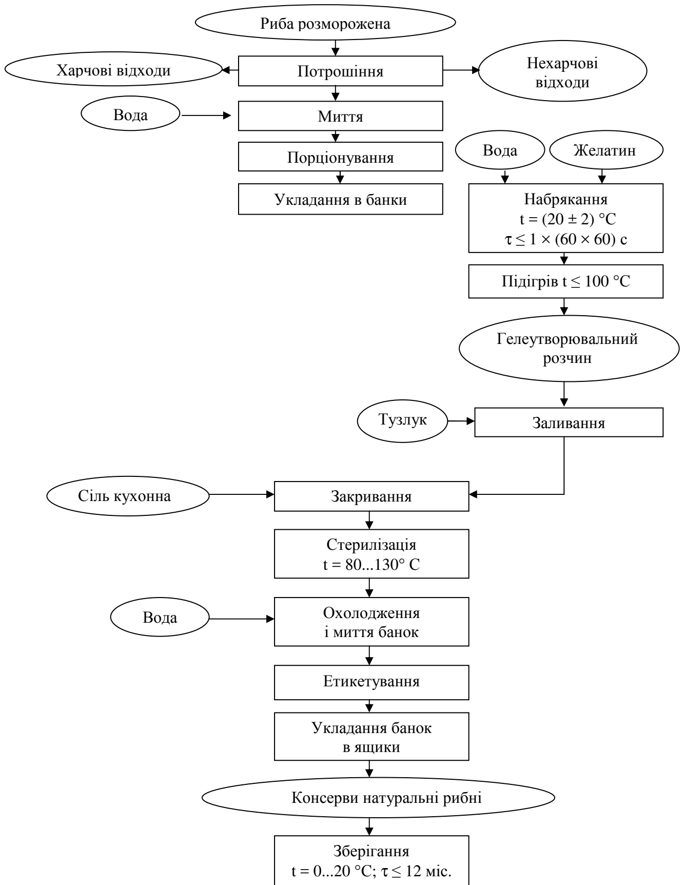
Рисунок 4.14 – Технологічна схема виробництва консервів натуральних
