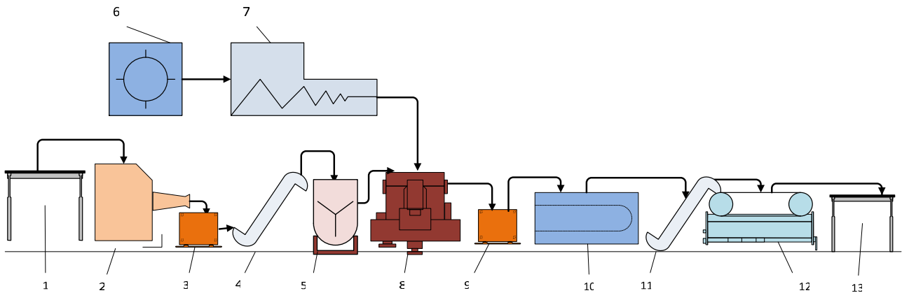
Рисунок 1.28 – Апаратурно-технологічна схема пельменів: 1 – стіл; 2 – вовчок; 3 – візок ; 4 – підйомник; 5 – фаршмішалка; 6 – просіювач; 7 –тістомісильна машина; 8 – автомат пельменний; 9 – візок; 10 – камера швидкої заморозки; 11 – підйомник; 12 – машина пакувальна; 13 – стіл
