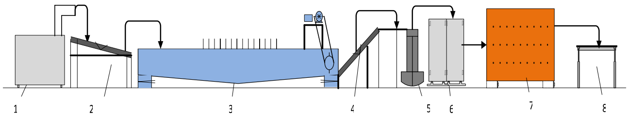
Рисунок 4.24 – Апаратурно-технологічна схема риби в’яленої: 1 – мийна машина; 2 – машина сортувальна; 3 – ванни механізовані для засолу; 4 – транспортери; 5 – машина нанизувальна; 6 – рама; 7 – кліматична установка для в’ялення риби з повним контролем технологічного процесу за заданими в систему управління програмами користувача; 8 – стіл
