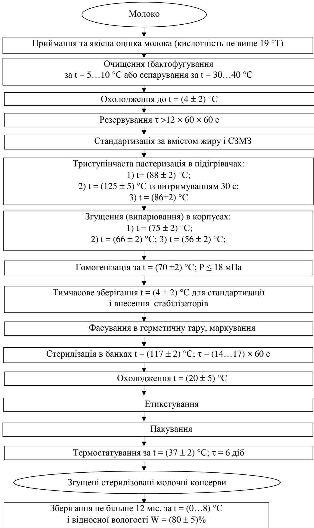
Рисунок 3.31 – Технологічна схема виробництва згущених стерилізованих молочних консервів
