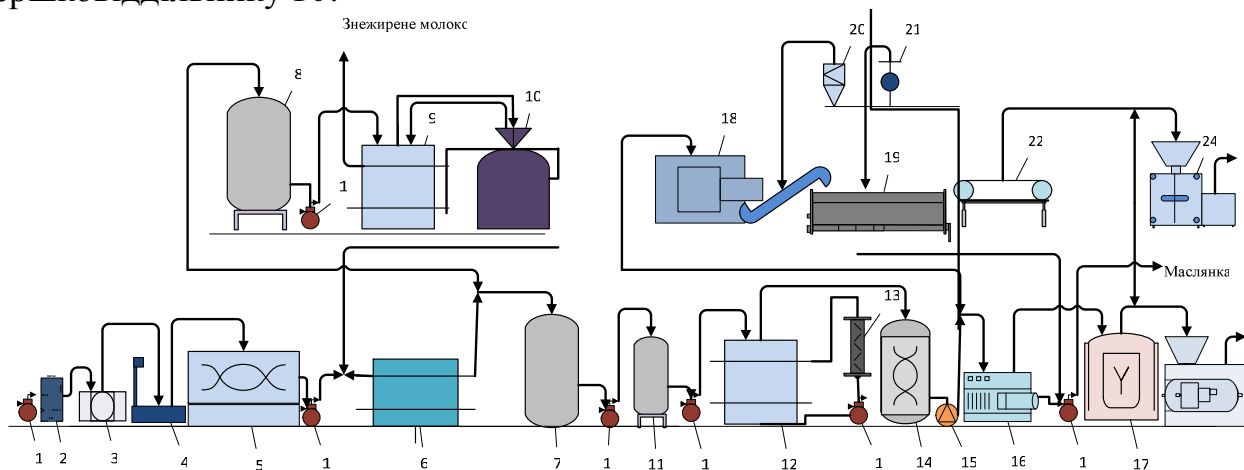
Рисунок 3.24 – Апаратурно-технологічна схема масла способом збивання: 1 – насос; 2 – лічильник; 3 – фільтр; 4 – ваги; 5 – ванна прийомна; 6 – теплообмінник пластинчастий; 7 – резервуар проміжний; 8 – ємність для молока; 9 – установка пастеризаційно-охолоджувальна; 10 – сепаратор-вершковіддільник; 11 – бак зрівняльний; 12 - установка пастеризаційно-охолоджувальна; 13 – установка вакуумдезодораційна; 14 – апарат вершкодозрівальний; 15 – насос гвинтовий; 16 – маслоутворювач періодичної дії; 17 – гомогенізатор-пластифікатор; 18 – маслоутворювач безперервної дії; 19 – бачок для маслянки; 20 – бачок для води; 21 – насос дозуючий; 22 – конвеєр; 23, 24 – машини фасувальні
