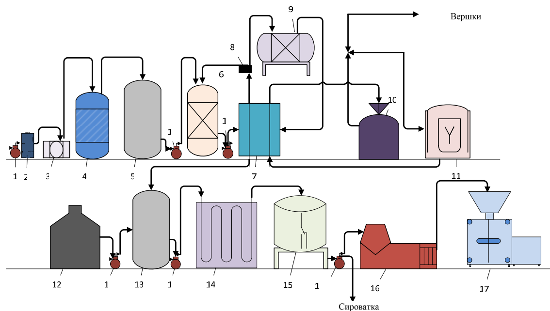
Рисунок 3.19 – Апаратурно-технологічна схема кисломолочного сиру: 1 – насос; 2 – лічильник; 3 – фільтр; 4 – охолоджувач; 5 – резервуар проміжний; 6 – бак зрівняльний; 7 – установка пастеризаційно-охолоджувальна; 8 – клапан зворотний; 9 – витримувач трубчастий; 10 – сепаратор-вершковіддільник; 11 – гомогенізатор; 12 – ємність для закваски; 13 – резервуар для сквашування; 14 – теплообмінник трубчастий; 15 – зневоджувач барабанний; 16 – охолоджувач двоциліндровий; 17 – автомат для фасування і пакування сиру
