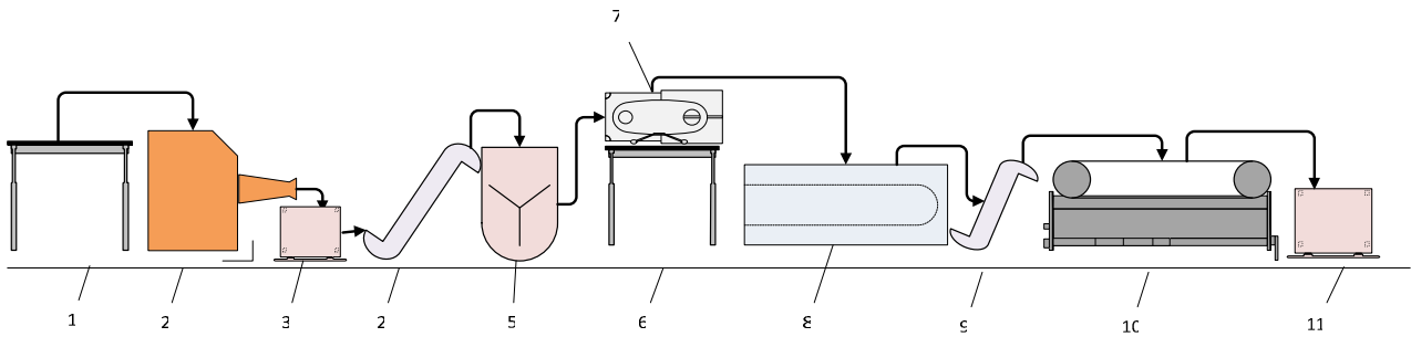
Рисунок 1.25 – Апаратурно-технологічна схема заморожених посічених напівфабрикатів: 1 – стіл; 2 – вовчок; 3 – візок; 4 – підйомник; 5 – фаршмішалка; 6 – стіл; 7 – автомат для формування напівфабрикатів; 8 – камера швидкої заморозки; 9 – підйомник; 10 – машина пакувальна; 11 – стіл
