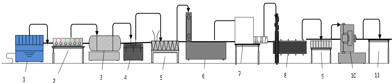
Рисунок 4.26 – Апаратурно-технологічна схема риби з кістковим скелетом: 1 – дефростер водяний; 2 – конвеєр стрічковий; 3 – машина для зняття луски; 4 – машина для відділення плавників; 5 – машина для відсікання голів; 6 – універсальний пристрій для переробки риби; 7 – машина для видалення хребетних і реберних кісток; 8 – машина для зняття шкіри; 9 – конвеєр для інспекції; 10 – апарат для виробництва н/ф; 11 – стіл
