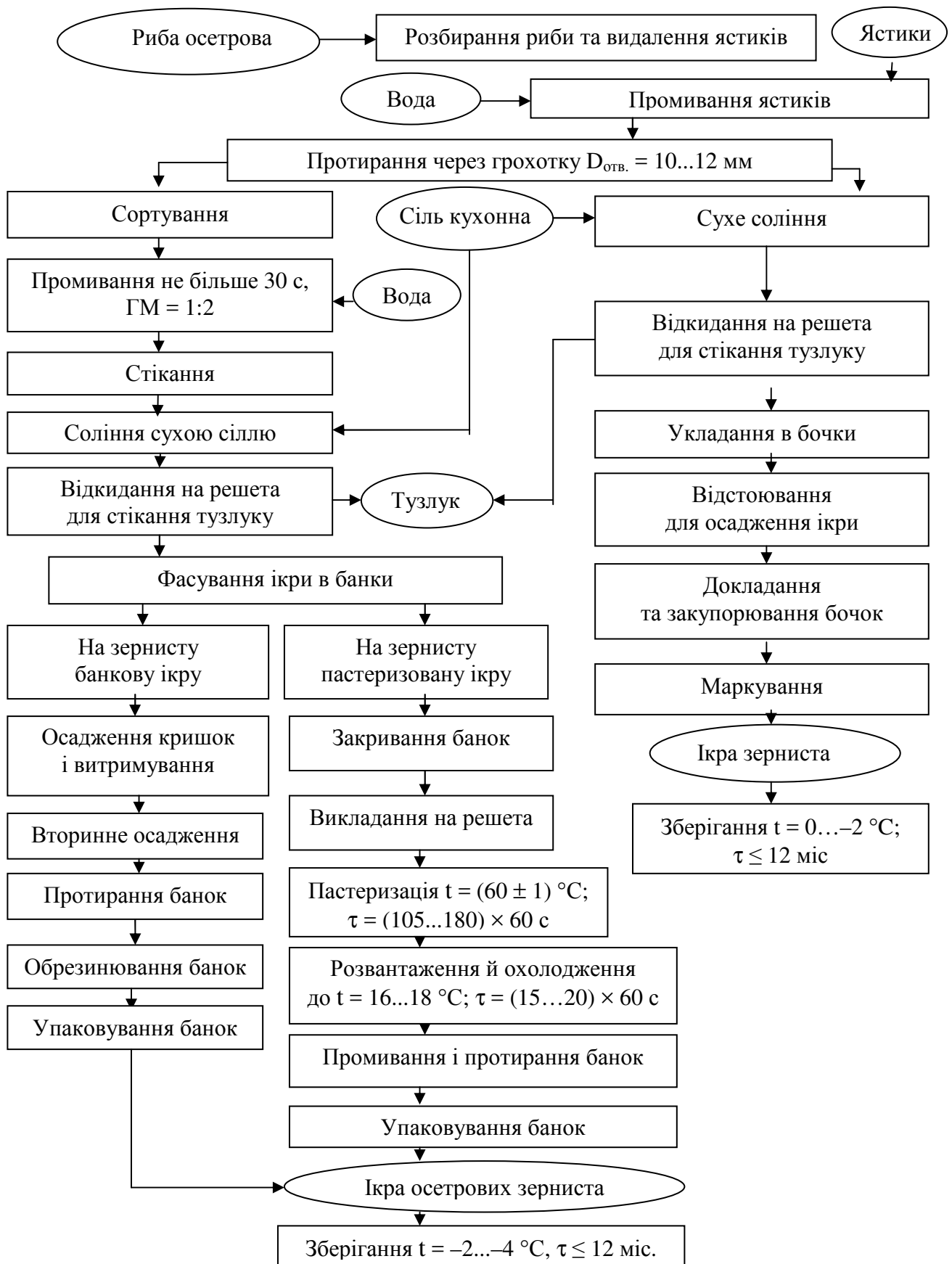
Рисунок 4.20 – Технологічна схема виробництва зернистої ікри осетрових риб
