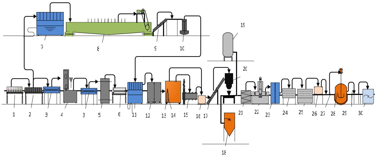
Рисунок 4.17 – Апаратурно-технологічна схема консервів з копченої риби в олії: 1 – конвеєр стрічковий; 2 – конвеєр для інспекції; 3 – транспортер мийний; 4 – універсальний пристрій для переробки риби; 5 – автомат для соління; 6 – конвеєр перев’язування шпагатом; 7 – дефростер (для розморожування дрібної риби); 8 – ванна механізована для засолу; 9 – транспортер; 10 – машина нанизувальна; 11 – транспортер для стікання зайвої вологи; 12 – рама; 13 – димогенератор; 14 – камера копильна; 15 – машина поділу на порції (для великої риби); 16 – візок; 17 – підйомник; 18 – автомат для шпарення; 19 – резервуар з олією; 20 – автомат набивний; 21 – клинчер; 22 – автоматична закатна машина; 23 – машина мийна; 24 – сітка однорядна; 25 – завантажувальний пристрій; 26 – вагонетка; 27 – шлях рейковий; 28 – автоклав для стерилізації; 29 – конвеєр; 30 – ванна з конвеєром
