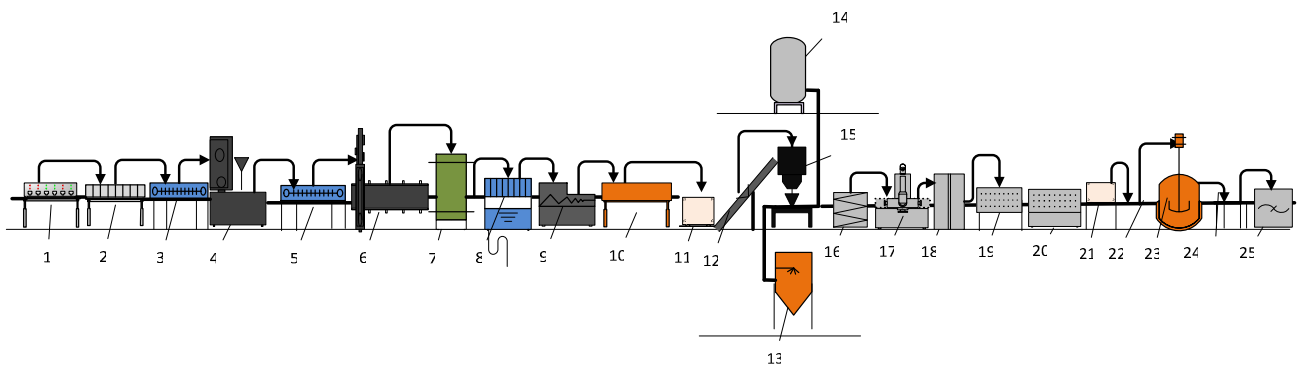
Рисунок 4.16 – Апаратурно-технологічна схема рибних консервів у томатному соусі: 1 – конвеєр стрічковий; 2 – конвеєр для інспекції; 3 – транспортер мийний; 4 – універсальний пристрій для переробки риби; 5 – транспортер мийний; 6 – машина поділу на порції; 7 – автомат для соління; 8 – транспортер для видалення зайвої вологи; 9 – апарат для панірування; 10 – апарат для смаження; 11 – візок; 12 – підйомник; 13 – автомат для шпарення; 14 – резервуар із томатним соусом; 15 – автомат набивний; 16 – клинчер; 17 – автоматична закатна машина; 18 – машина мийна для закупорених банок; 19 – сітка однорядна; 20 – завантажувальний пристрій; 21 – візок; 22 – шлях рейковий; 23 – автоклав для стерилізації; 24 – конвеєр; 25 – ванна з конвеєром
