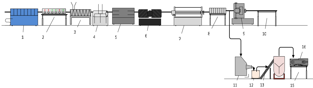
Рисунок 4.27 – Апаратурно-технологічна схема риби з хрящовим скелетом: 1 – дефростер; 2 – конвеєр стрічковий; 3 – машина для відсікання голів; 4 – машина для відділення плавників; 5 – машина для видалення спинної хорди (візіги); 6 – машина для філерування; 7 – машина для зачищення шкіри та ланкування; 8 – конвеєр для інспекції; 9 – апарат для виробництва н/ф (порційні шматки); 10 – стіл; 11 – вовчок; 12 – візок; 13 – підйомник; 14 – фаршмішалка; 15 – стіл; 16 – автомат для формування напівфабрикатів
