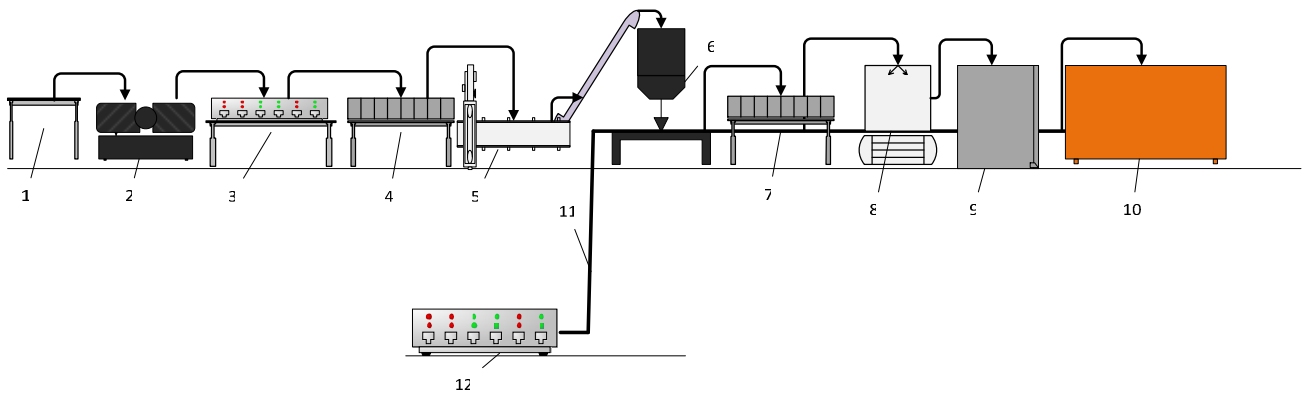
Рисунок 4.19 – Апаратурно-технологічна схема рибних пресервів: 1 – стіл; 2 – машина для розділення на філе; 3 – конвеєр стрічковий; 4 – конвеєр для інспекції; 5 – машина для зняття шкіри; 6 – автомат набивний; 7 – конвеєр для інспекції; 8 – машина дозувально-наповнювальна; 9 – машина для закручування без вакууму; 10 – комплекс устаткування для впаковування пресервів; 11 – накопичувальний конвеєр; 12 – мийна машина для тари
