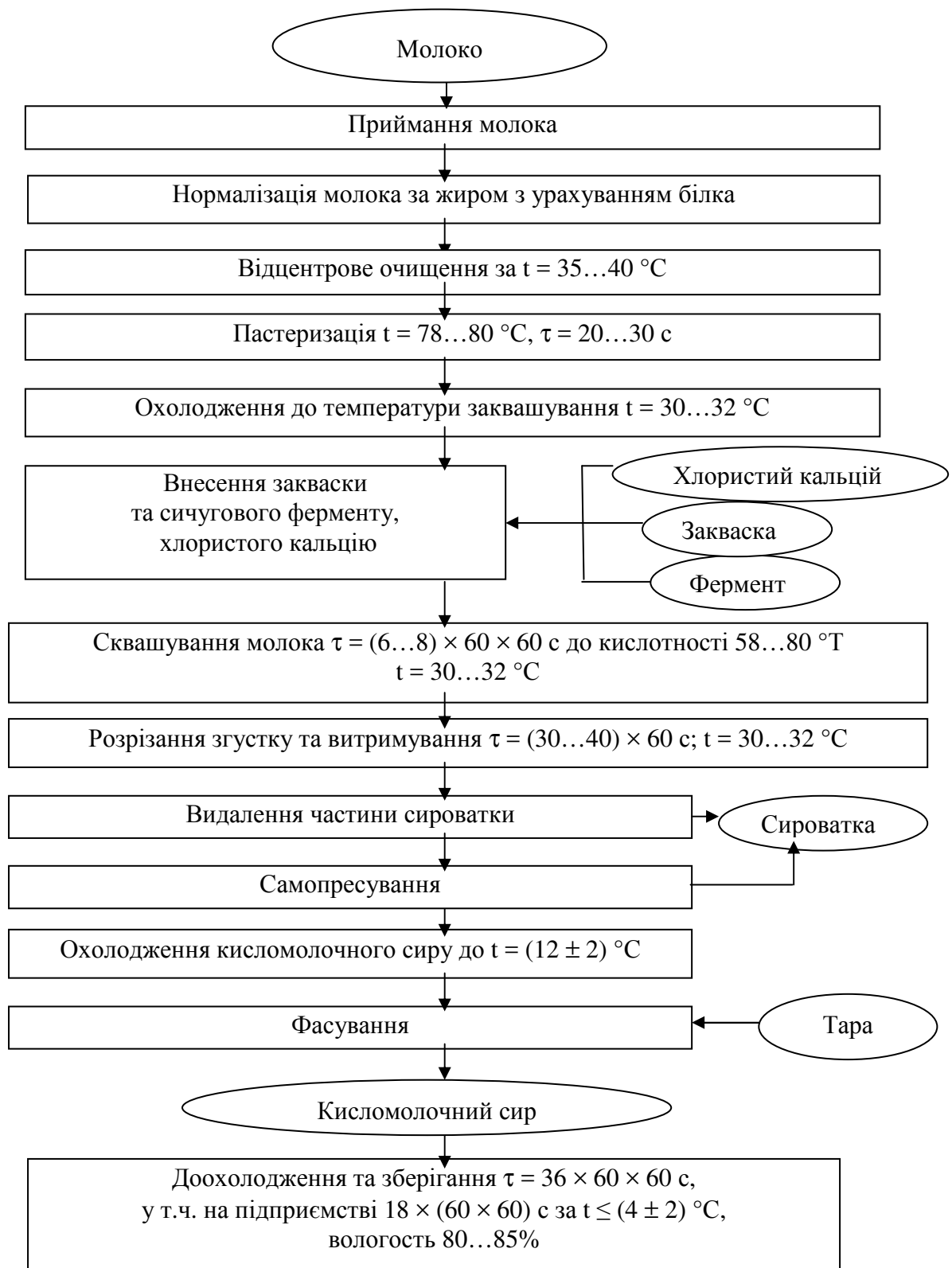
Рисунок 3.18 – Технологічна схема виробництва сиру кисломолочного кислотно-сичуговим способом
