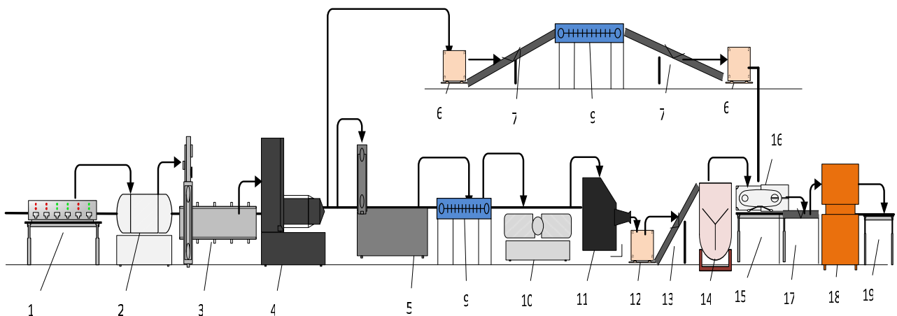
Рисунок 4.28 – Апаратурно-технологічна схема риби фаршированої зі спинним плавником, розташованим біля хвоста: 1 – конвеєр стрічковий; 2 – машина для зняття луски; 3 – машина для зняття шкіри; 4 – машина для видалення хребтних і реберних кісток; 5 – універсальний пристрій для переробки риби; 6 – візок; 7 – підйомник; 8, 9 – транспортери мийні; 10 – машина для філерування; 11 – вовчок; 12 – візок; 13 – підйомник; 14 – фаршмішалка; 15 – стіл; 16 – автомат для формування напівфабрикатів; 17 – стіл для перевязки шпагатом; 18 – термокамера; 19 – стіл для інспекції
