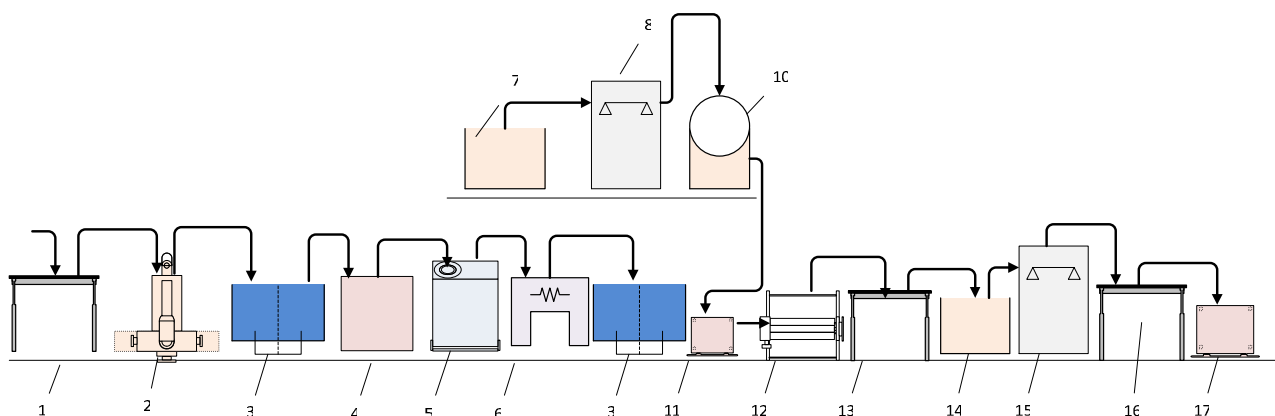
Рисунок 2.3 – Апаратурно-технологічна схема переробки птиці: 1 – стіл; 2 – апарат для електроглушення; 3 – ванна для знекровлювання; 4 – ванна для ошпарювання; 5 – машина для зняття пера; 6 – установка для обпалювання; 7 – ванна для воскування; 8 – пристрій для охолодження воскомаси; 9 – ванна; 10 – машина для зняття воскового нальоту; 11 – візок; 12 – машина для відрізання ніг і голів; 13 – стіл для патрання; 14 – ванна; 15 – холодильна камера; 16 – стіл; 17 – візок
