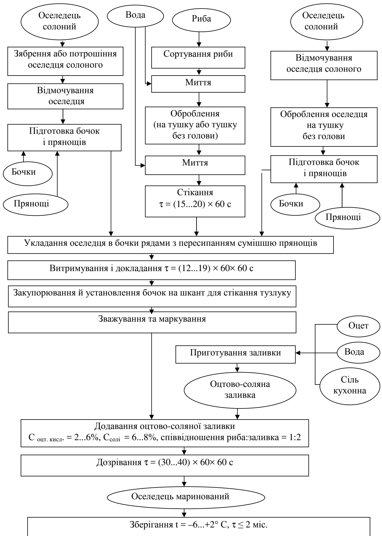
Рисунок 4.9 – Технологічна схема виробництва оселедця маринованого
