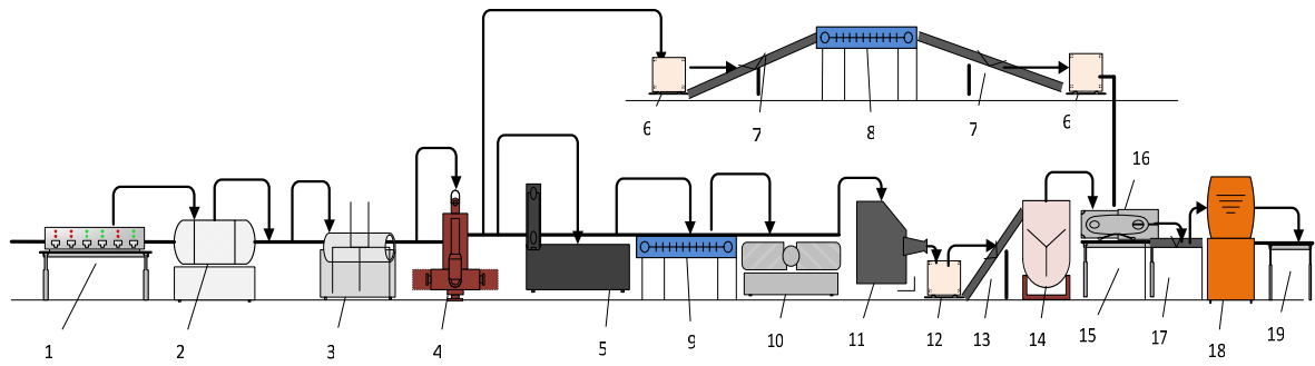
Рисунок 4.29 – Апаратурно-технологічна схема риби фаршированої зі спинним плавником уздовж усієї спини: 1 – конвеєр стрічковий; 2 – машина для зняття луски; 3 – машина для розрубання плавників (крім спинного) та вирізання спинного (глибокі надрізи до ребер і перерізання їх); 4 – машина для зламування хвоста біля хребта і голови та видалення хребта через надрізи в спині; 5 – універсальний пристрій для переробки риби; 6 – візок; 7 – підйомник; 8, 9 – транспортери мийні; 10 – машина для філерування; 11 – вовчок; 12 – візок; 13 – підйомник; 14 – фаршмішалка; 15 – стіл; 16 – автомат для фарширування; 17 – стіл для загортання та перев’язування шпагатом; 18 – котел для варіння н/ф; 19 – стіл для охолодження та знімання шпагату і марлі
