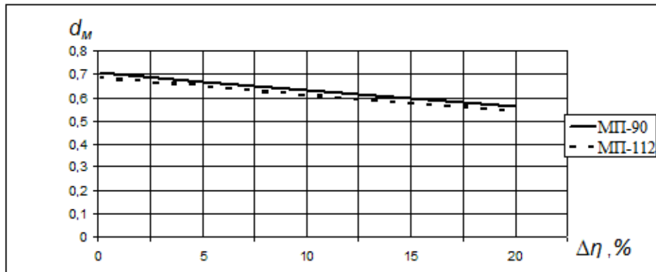
Рис. 12 Зависимости изменения декремента затухания d_M при уменьшении к.п.д. моторов \Delta\eta
