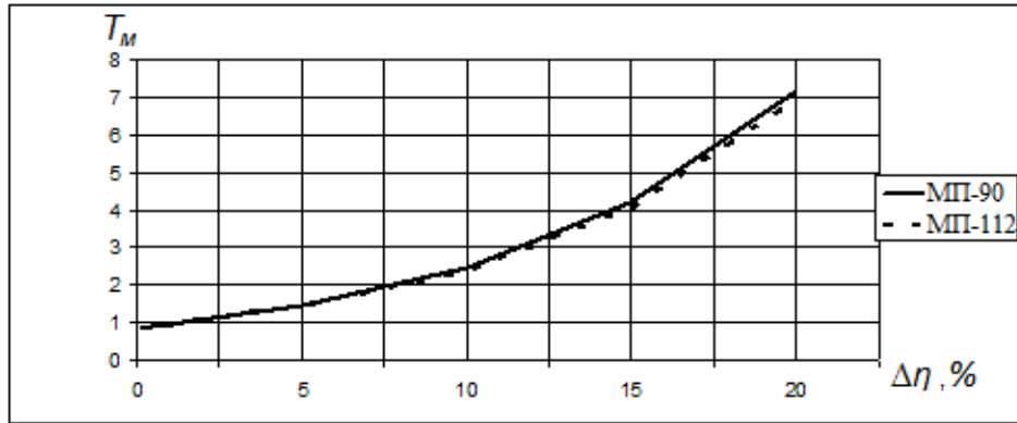
Рис. 11 Зависимости изменения постоянной времени T_M при уменьшении к.п.д. моторов \Delta\eta
