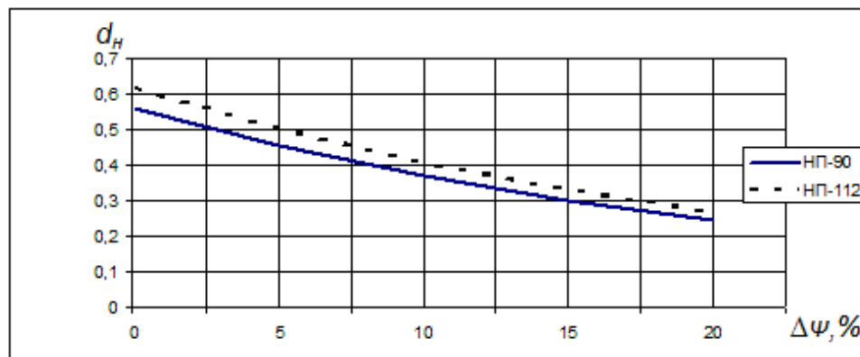
Рис. 6. Зависимости декрементов затухания d_n при уменьшении коэффициента подачи насосов \Delta\psi
