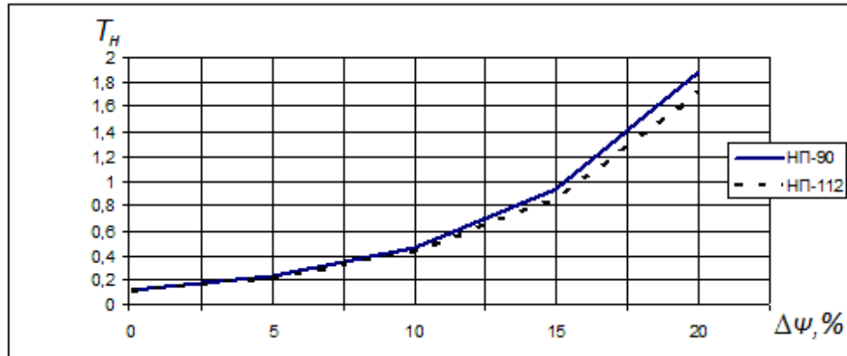
Рис. 5. Зависимости постоянных времени T_n при уменьшении коэффициента подачи насосов \Delta\psi
