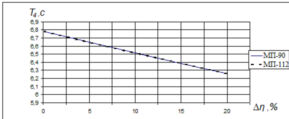
Рис. 10 Зависимости изменения постоянной времени T_4 при уменьшении к.п.д. моторов \Delta\eta
