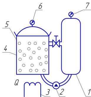
Рис. Пристрій для імпульсного заморожування: 1 – вакуумний ресивер; 2 – насос; 3 – холодильний компресор; 4 – технологічна ємність з матеріалом; 5 – вимірвальний перетворювач температури; 6, 7 – манометри
