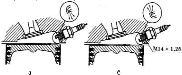
Рисунок 2 - Нераціональне (а) і раціональне (б) положення свічки запалювання
