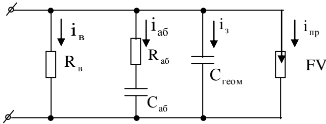
Рисунок 1 - Схема заміщення ізоляції: R_в - резистор, який характеризує опір струму витікання; C_{аб} - ємність, що зумовлена дипольною поляризацією; R_{аб} - резистор, який характеризує еквівалентні втрати при дипольній поляризації; C_{геом} - ємність електронної поляризації (залежить від геометричних розмірів ізоляції); FV - розрядник; \dot{i}_{пр} - струм пробую
