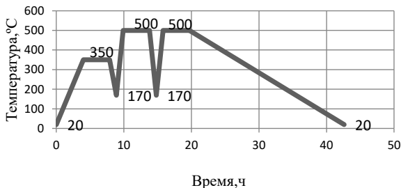
Рис.2. Рекомендуемая схема режима ТО, обеспечивающая получение оптимальных параметров, характеризующих структурное состояние сплава и твердости
