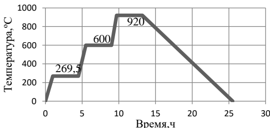
Рис.1. Схема режима ТО, в результате которой получены максимальные значения характеристик, описывающих степень неоднородности структуры исследуемых сплавов после термической обработки
