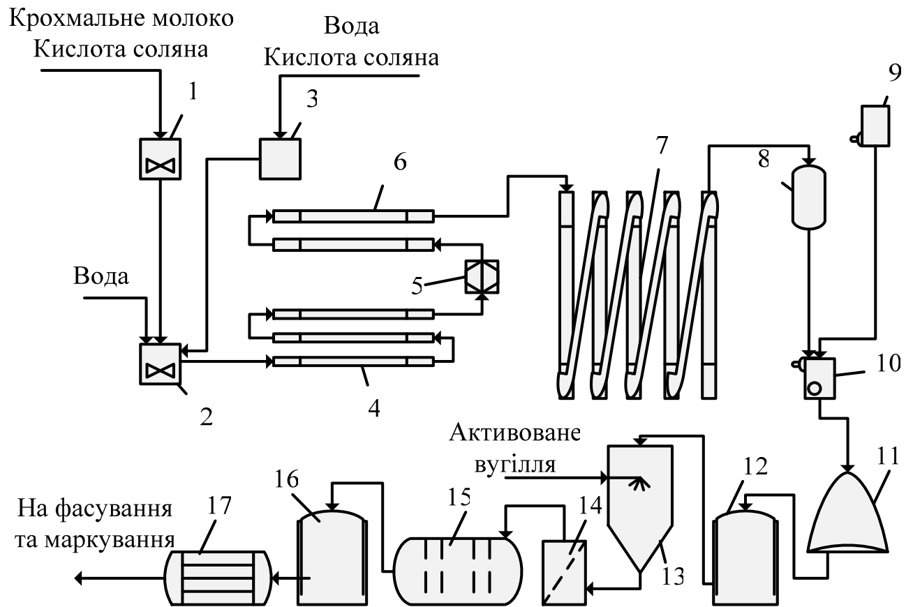
Рисунок А.15 – Апаративно-технологічна схема виробництва патоки: 1 – збірник первинний; 2 – збірник вторинний; 3 – збірник соляної кислоти; 4 – теплообмінник; 5 – конденсатовідвідник; 6 – трубчастий нагрівач; 7 – мідний трубопровід для оцукрення; 8 – випарник; 9 – збірник кальцинованої соди; 10 – збірник кінцевої нейтралізації; 11 – скімер для очищення патоки; 12 – вакуум-фільтрувальна установка; 13 – реактор; 14 – фільтруюча установка; 15 – багатокорпусний випарний апарат; 16 – вакуум-апарат для уварювання; 17 – трубчастий охолоджувач
