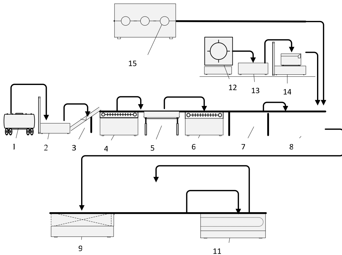
Рисунок А.36 – Апаратурно-технологічна схема виробництва плодів та ягід заморожених: 1 – електронавантажувач; 2 – контейнер; 3 – транспортер; 4, 6 – мийні машини; 5 – інспекційний конвеєр; 7 – елеватор; 8 – машина фасувальна; 9 – камера швидкого заморожування; 10 – пакувальна машина; 11 – холодильна камера для зберігання плодів та ягід заморожених; 12 – вібросто для просіювання; 13 – сність; 14 – ваги; 15 – мийна машина для тари; 16 – конвеєр для транспортування тари
