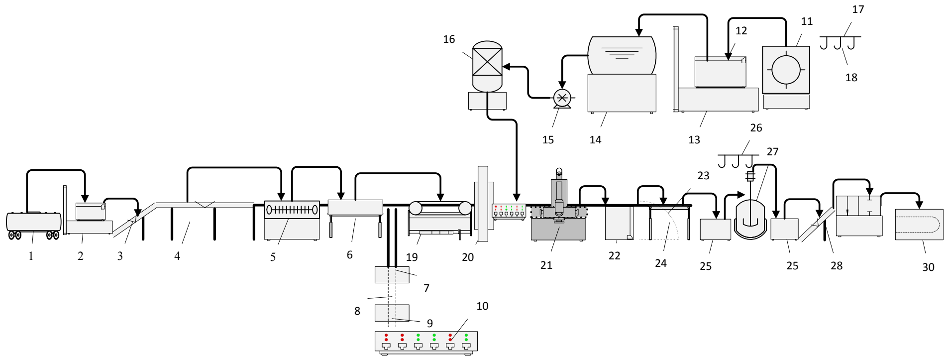
Рисунок А.35 – Апаратурно-технологічна схема виробництва плодів та ягід маринованих: 1 – відкидач тари; 2 – ваги; 3 – транспортер; 4 – інспекційний сортувальний конвеєр; 5 – мийна машина; 6 – калібрувальний конвеєр; 7 – ошпарювач; 8 – конвеєр; 9 – екран для перегляду пляшок; 10 – машина для миття пляшок; 11 – вібросито для просіювання; 12 – ємність; 13 – ваги; 14 – варильний казан з водою; 15 – насос; 16 – мірний збірник, 17 – балка; 18 – електротельфер; 19 – фасувальний конвеєр; 20 – автомат-наповнювач; 21 – автоматична закатна машина; 22 – бракеражний автомат; 23 – конвеєр; 24 – стіл-накопичувач; 25 – ємність; 26 – електротельфер; 27 – автоклав для стерилізації; 28 – транспортер; 29 – автоматична машина маркування; 30 – холодильна камера
