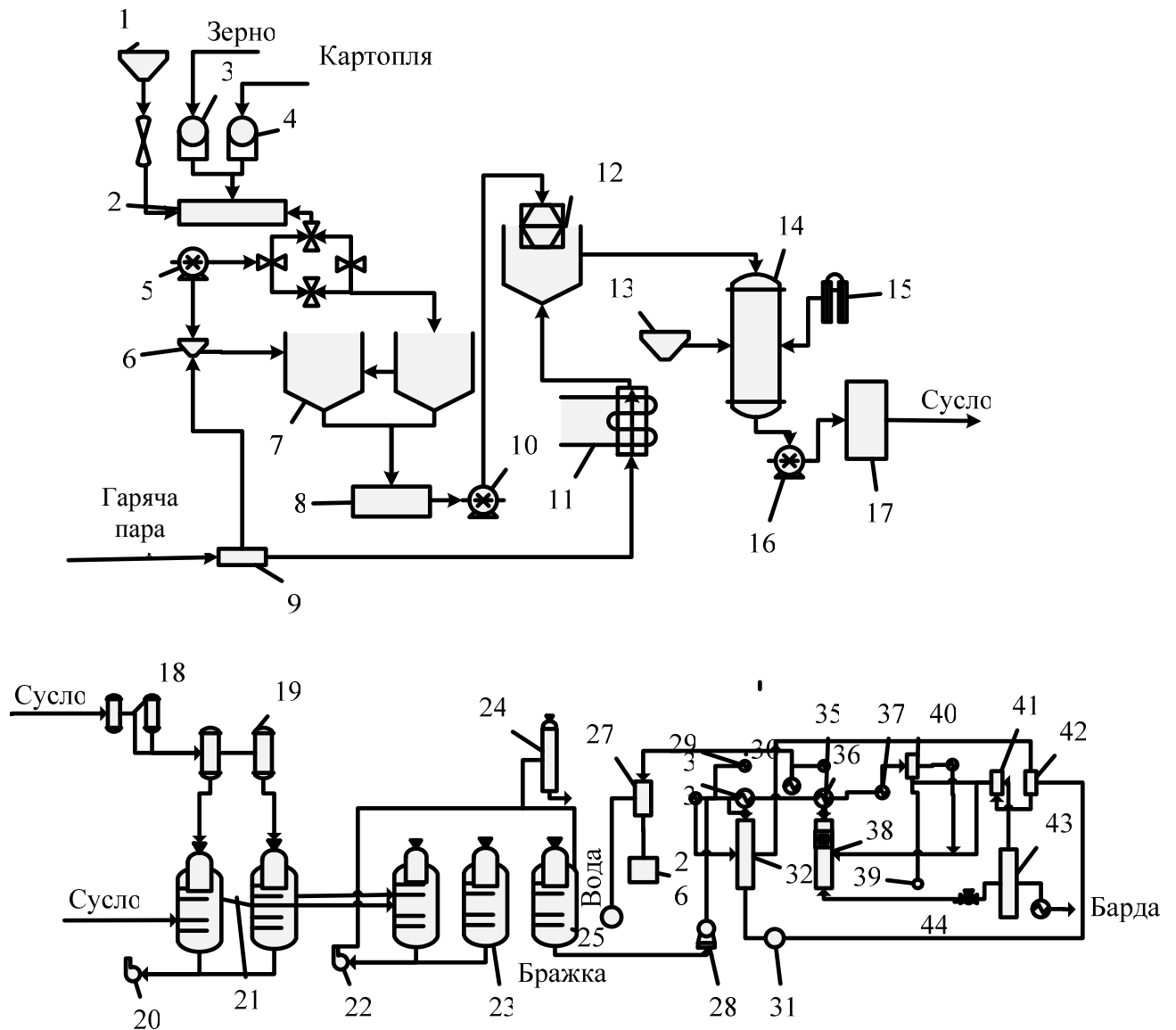
Рисунок А.18 – Апаратурно-технологічна схема виробництва спирту етилового ректифікованого харчового: 1 – збірник витратний; 2 – змішувач; 3, 4 – дробарки молоткові; 5, 10, 16, 20, 22, 25, 28, 31, 39 – насоси; 6 – головка контактна; 7 – апарат гідродинамічної і ферментативної обробки I ступеня; 8 – апарат гідродинамічної і ферментативної обробки II ступеня; 9 – розподільник; 11 – трубчастий стерилізатор; 12 – паросепаратор; 13 – збірник видатковий; 14 – випарник; 15 – збірник; 17 – апарат теплообмінний; 18 – дріжджанки; 19 – зброжувачі; 21 – апарат головний бродильний; 23 – апарат бродильний; 24, 29, 34 – спиртопастки; 26 – збірник барометричної води; 27 – барометричний конденсатор; 30, 36 – дефлегматори; 32 – колона ректифікації; 33 – конденсатор; 35 – вакуум-насос; 37 – теплообмінник; 38, 43 – брагоопераційні колони; 40 – сепаратор; 41 – колектор; 44 – пінопастка
