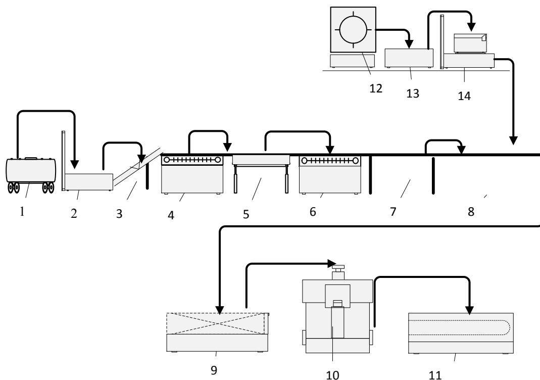
Рисунок А.31 – Апаратурно-технологічна схема виробництва плодів та ягід заморожених: 1 – електронавантажувач; 2 – контейнер; 3 – транспортер; 4, 6 – мийні машини; 5 – конвеєр інспекційний; 7 – елеватор; 8 – машина фасувальна; 9 – камера швидкого заморожування; 10 – машина пакувальна; 11 – холодильна камера для зберігання плодів та ягід заморожених; 12 – вібрсито для просіювання; 13 – ємність; 14 – ваги
