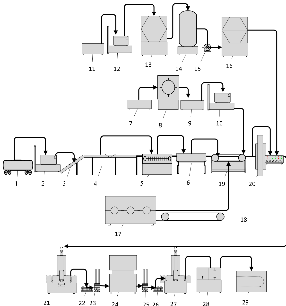
Рисунок А.32 – Апаратурно-технологічна схема виробництва плодів та ягід мочених: 1 – електронавантажувач; 2, 10, 12 – ваги; 3 – транспортер; 4 – інспекційний сортувальний конвеєр; 5 – мийна машина; 6 – калібрувальний конвеєр; 7, 9, 11 – контейнери; 8 – вібросито для просіювання; 13, 16 – двостінні казани; 14 – резервуар; 15 – насос плужерний; 17 – машина мийна для тари; 18 – конвеєр для транспортування тари; 19 – конвеєр для укладання плодів, житньої соломи, прянощів; 20 – автомат-наповнювач; 21, 27 – автоматичні закатні машини; 22, 26 – піддони; 23, 25 – електронавантажувачі; 24 – термокамера; 28 – автоматична машина для маркування; 29 – холодильна камера
