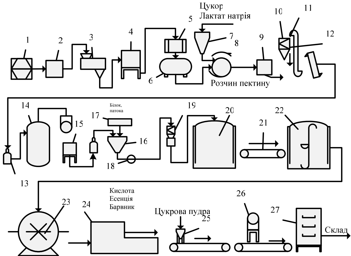
Рисунок А.4 – Апаратурно-технологічна схема виробництва зефіру на пектині: 1 – бочка; 2 – ємність із мішалкою; 3 – машина протиральна; 4 – ємність проміжна; 5 – дозатор об'ємний; 6 – пектинорозчиняльник; 7 – носовий дозатор; 8 – котел з мішалкою варильний; 9 – ємність приймальна; 10 – бункер проміжний; 11 – норія; 12 – просіювач; 13 – насос; 14 – апарат змійовиковий варильний; 15 – ємність; 16, 17, 18 – станції безперервної дії; 19 – воронка формувальної машини; 20 – апарат для охолодження; 21 – конвеєр; 22 – апарат для структуроутворення; 23 – апарат для підсушування; 24 – кліматична установка; 25 – машина для обсипання; 26 – ваги; 27 – стелажні візки
