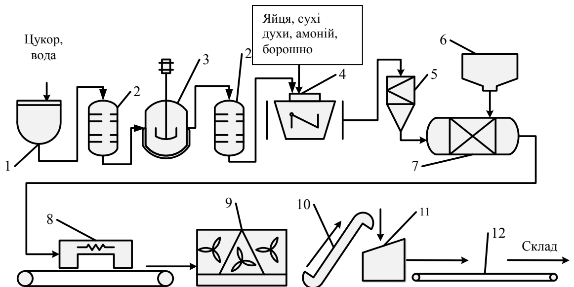
Рисунок А.6 – Апаратурно-технологічна схема виробництва пряників: 1 – ємність для розчинення цукру; 2 – фільтрувальний апарат; 3 – варильний апарат; 4 – машина місильна; 5 – машина формувально-відсадна; 6 – бачок для сиропу з паровою оболонкою; 7 – апарат для нанесення малюнка на пряники; 8 – піч конвеєрна; 9 – шафа охолоджувальна; 10 – транспортер передавальний; 11 – скидач; 12 – транспортер укладальний
