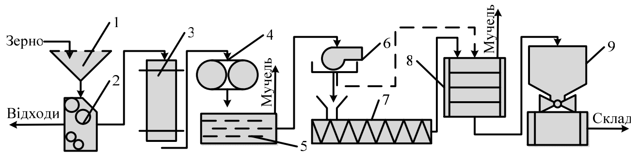
Рисунок А.12 – Апаратурно-технологічна схема виробництва круп: 1 – сепаратор; 2 – дуаспіратор; 3 – колонка магнітна; 4 – система лушення; 5 – розсів; 6 – аспіратор із замкнутим циклом повітря; 7 – машина шліфувальна; 8 – машина круповіддільна; 8 – машина фасувальна
