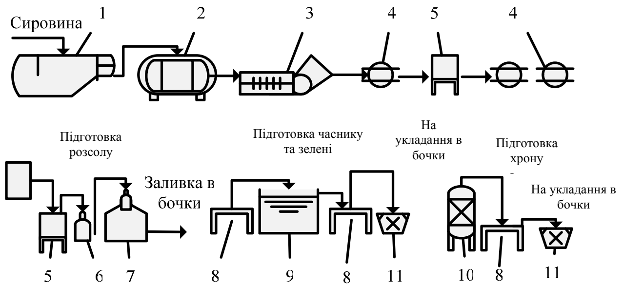
Рисунок А.26 – Апаратурно-технологічна схема виробництва солінь з овочів: 1 – машина мийна універсальна щіткова; 2 – машина мийна; 3 – транспортер інспекційний; 4 – ваги; 5 – бак накопичувальний; 6 – солерозчинник; 7 – реактор; 8 – стіл; 9 – ванна для миття зелені; 10 – овочерізка універсальна; 11 – ємність
