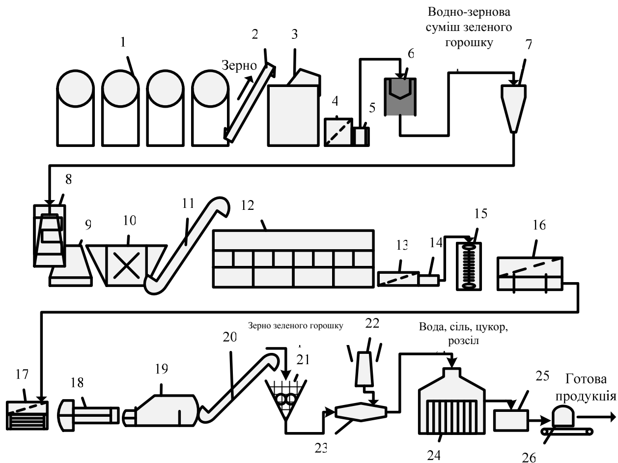
Рисунок А.28 – Апаратурно-технологічна схема виробництва консервів «Зелений горошок» (зі свіжої сировини): 1 – горохомолотарка; 2 – ківшовий конвеєр; 3 – сито вібраційне; 4 – віялка; 5 – машина флотаційна мийно-сортувальна; 6 – збірник; 7 – приймальний бункер; 8 – машина для відділення зерна від листя; 9 – машина двобарабанна мийна; 10 – машина флотаційна мийна; 11 – конвеєр; 12, 13 – машини барабанні сортувальні; 14 – насос; 15 – водороздільник; 16 – бланшувач; 17 – машина мийно-охолоджувальна; 18 – селектор прутковий; 19 – ополіскувач душовий; 20 – конвеєр; 21 – машина наповнювальна для горошку; 22 – пристрій для приготування розсолу; 23 – машина для наповнювання розсолем; 24 – стерилізатор; 25 – машина для миття і сушіння банок; 25 – машина лінійна етикетувальна; 26 – машина для укладання банок у ящики
