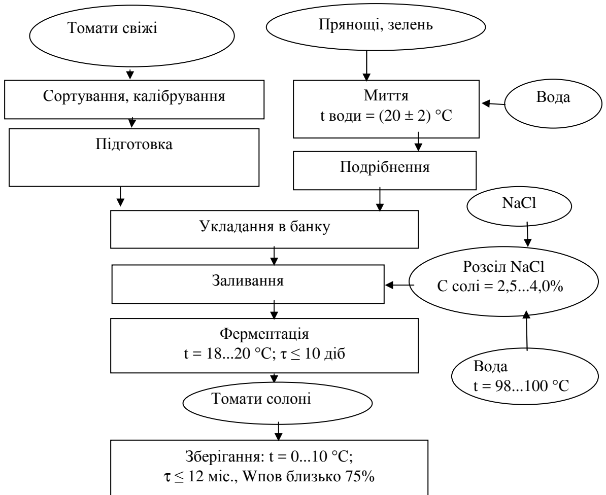
Рисунок 7.5 – Технологічна схема виробництва томатів солоних
