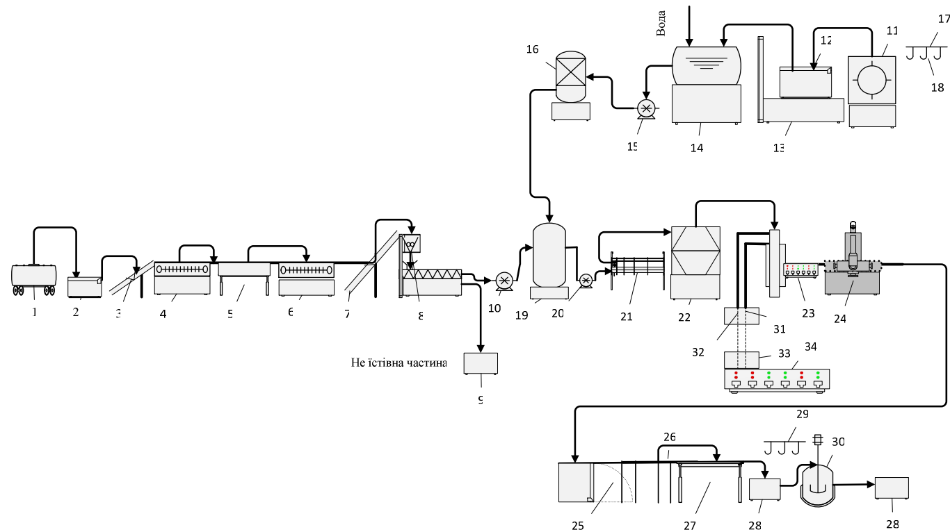
Рисунок А.33 – Апаратурно-технологічна схема виробництва варення, джему та конфітюру: 1 – відкидач тари; 2 – ємність; 3 – транспортер; 4, 6 – мийні машини; 5 – інспекційний конвеєр; 7 – елеватор; 8 – дискова дробарка; 9 – ємність для відходів; 10, 15, 20 – поршневі насоси; 11 – вібросто для просіювання; 12 – ємність; 13 – ваги; 14 – котел для варіння; 16 – мірний збірник; 17 – балка; 18, 29 – електротельфери; 19 – резервуар; 21 – трубчастий підігрівач; 22 – двостінний казан для підтримання постійної температури до початку фасування; 23 – розливний автомат; 24 – автоматична закатна машина; 25 – бракеражний автомат; 26, 32 – конвеєри; 27 – стіл-накопичувач; 28 – ємність; 30 – автоклав для стерилізації; 31 – ошпарювач; 33 – екран для перегляду пляшок; 34 – машина для миття пляшок
