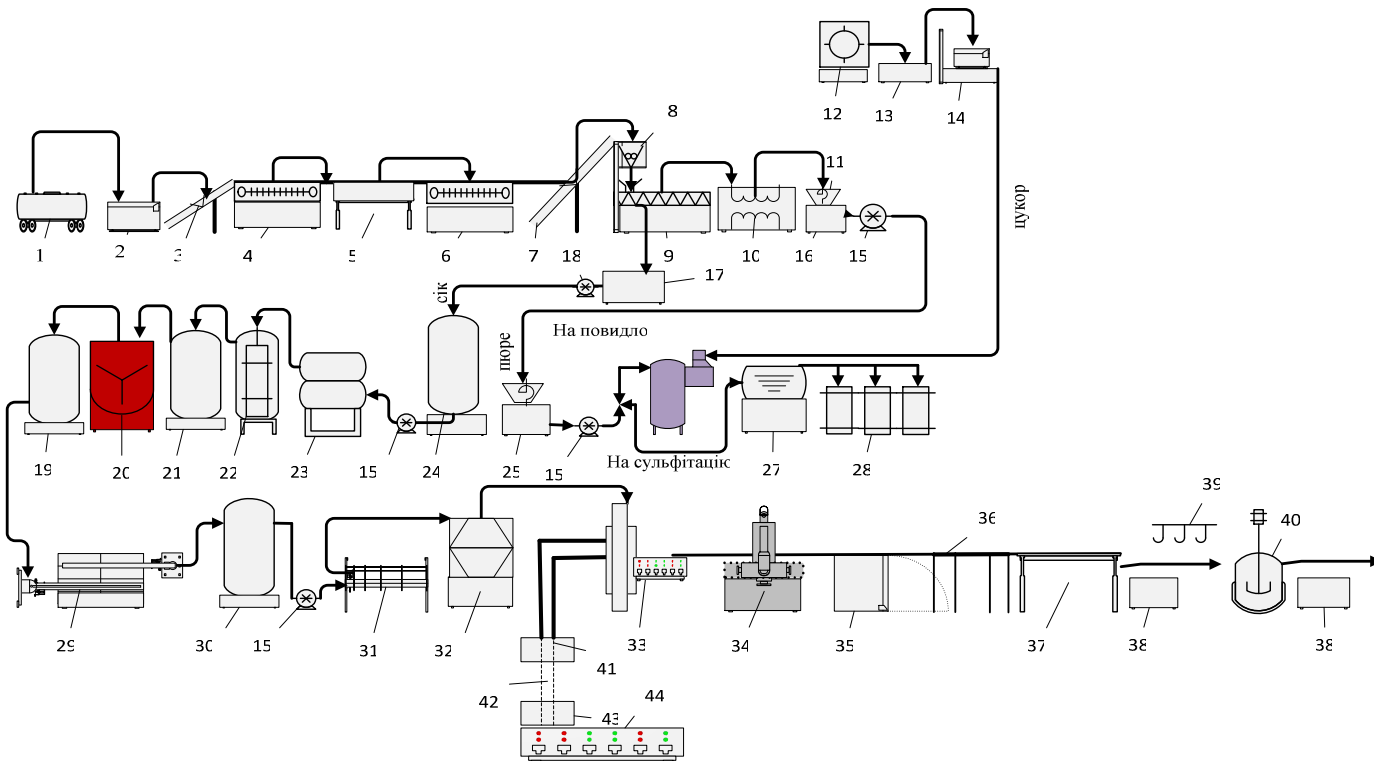
Рисунок А.34 – Апаратурно-технологічна схема виробництва повидла: 1 – відкидач тари; 2 – контейнер; 3 – транспортер; 4, 6 – мийні машини; 5 – інспекційний конвеєр; 7 – конвеєр; 8 – дискова дробарка; 9 – ємність для відходів; 10 – гвинтовий ошпарювач для вичавків; 11 – універсальна протиральна машина; 12 – вібрисито для просіювання; 13 – збірник; 14 – ваги; 15 – поршневий насос; 16 – ємність для протертого пюре; 17 – ємність для соку; 18 – плунжерний насос; 19 – резервуар; 20 – сепаратор; 21, 30 – резервуари; 22 – трубчастий охолоджувач; 23 – пастеризатор-охолоджувач; 24 – резервуар для відстоювання соку; 25 – протиральна машина; 26 – вакуум-апарат для виготовлення повидла або на сульфитацію; 27 – котел для варіння; 28 – бочки; 29 – фільтр-прес; 31 – трубчастий підігрівач; 32 – двостінний казан для підтримання постійної температури до початку фасування; 33 – розливний автомат; 34 – автоматична закатна машина; 35 – бракеражний автомат; 36, 42 – конвеєри; 37 – стіл-накопичувач; 38 – ємність; 39 – електротельфер; 40 – автоклав для стерилізації; 41 – ошпарювач; 43 – екран для огляду пляшок; 44 – машина для миття пляшок
