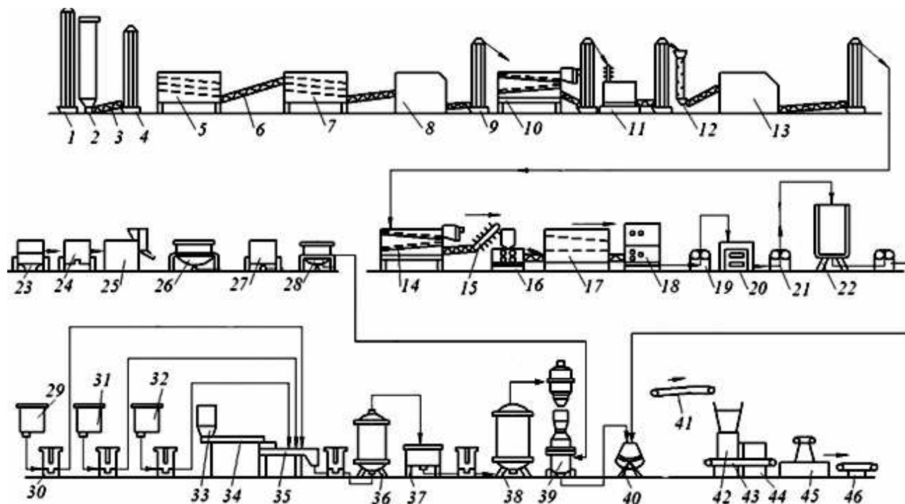
Рисунок А.2 – Апаратурно-технологічна схема виробництва халви: 1, 4, 9 – норії; 2 – бункер; 3, 6 – шнеки; 5 – сепаратор повітряно-ситовий; 7 – сепаратор; 8, 13 – машини рушильні; 10 – машина насінневіяльна; 11 – жаровня; 12 – шахтний охолоджувач; 14 – машина ситовіяльна; 15 – елеватор; 16 – верстат вальцьовий; 17 – сита вібраційні; 18 – верстат п'ятивалковий; 19 – насос шестеренний; 20 – машина протиральна; 21 – насос; 22 – збірник із мішалкою; 23 – ємність мийна; 24 – ємність для замочування; 25 – коренерізка; 26 – котел відкритий варильний; 27 – збірник проміжний; 28 – котел варильний; 29, 31, 32 – збірники для патоки, інвертного сиропу, води; 30 – насос-дозатор плунжерний; 33 – бункер для цукру; 34 – дозатор; 35 – змішувач; 36 – апарат змійовиковий варильний; 37 – збірник; 38 – вакуум-апарат змійовиковий безперервної дії; 39 – котел; 40 – машина місильна; 41 – конвеєр охолоджувальний; 42 – машина формувальна; 43 – конвеєр; 44 – конвеєр для охолодження; 45 – машина фасувальна; 46 – конвеєр
