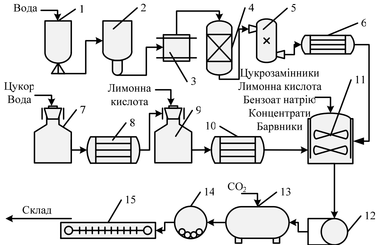
Рисунок А.24 – Апаратурно-технологічна схема виробництва напоїв безалкогольних: 1 – фільтр піщаний грубого очищення; 2 – керамічний свічковий фільтр; 3 – прес-фільтр тонкого очищення; 4 – фільтр катіонітовий; 5 – бактерицидна установка з ультрафіолетовими променями; 6 – холодильник; 7 – сироповарильний апарат; 8, 10 – теплообмінники; 9 – сироповарильний апарат; 11 – вертикальний купажний апарат; 12 – фільтр механічний; 13 – збірник напірний; 14 – лінія розливу; 15 – апарат етикетувальний
