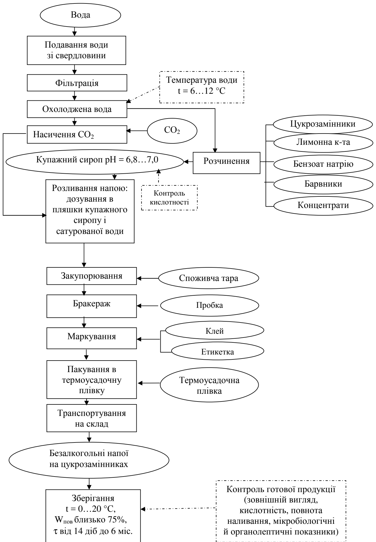
Рисунок 6.1 – Загальна технологічна схема напоїв безалкогольних на цукрозамінниках
