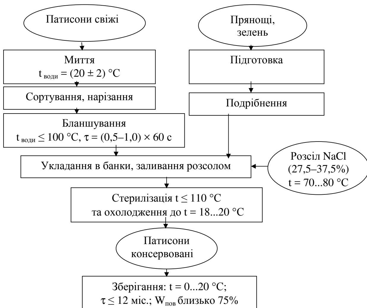
Рисунок 7.4 – Технологічна схема виробництва патисонів консервованих
