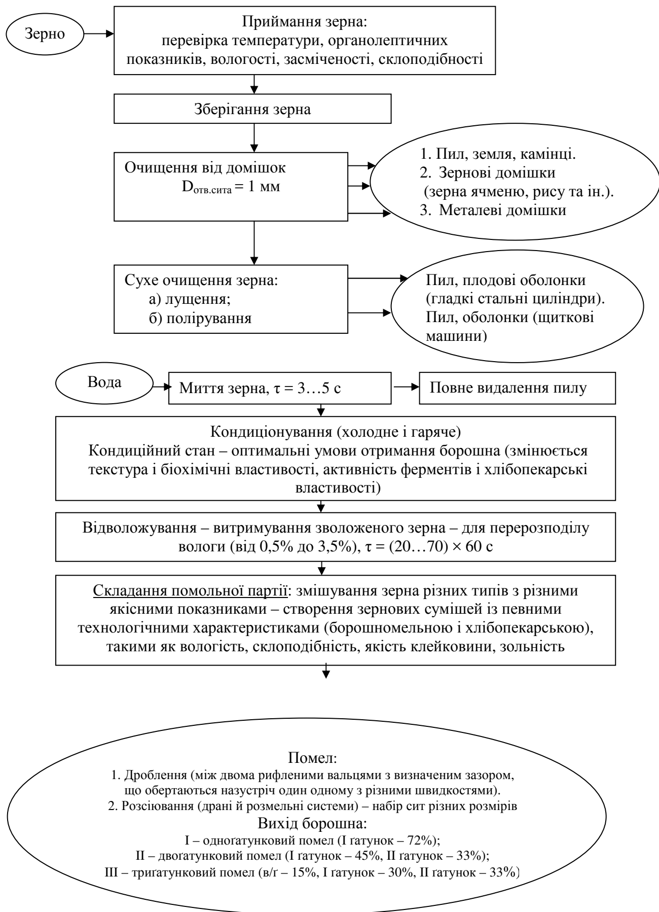
Рисунок 2.1 – Технологічна схема виробництва борошна пшеничного
