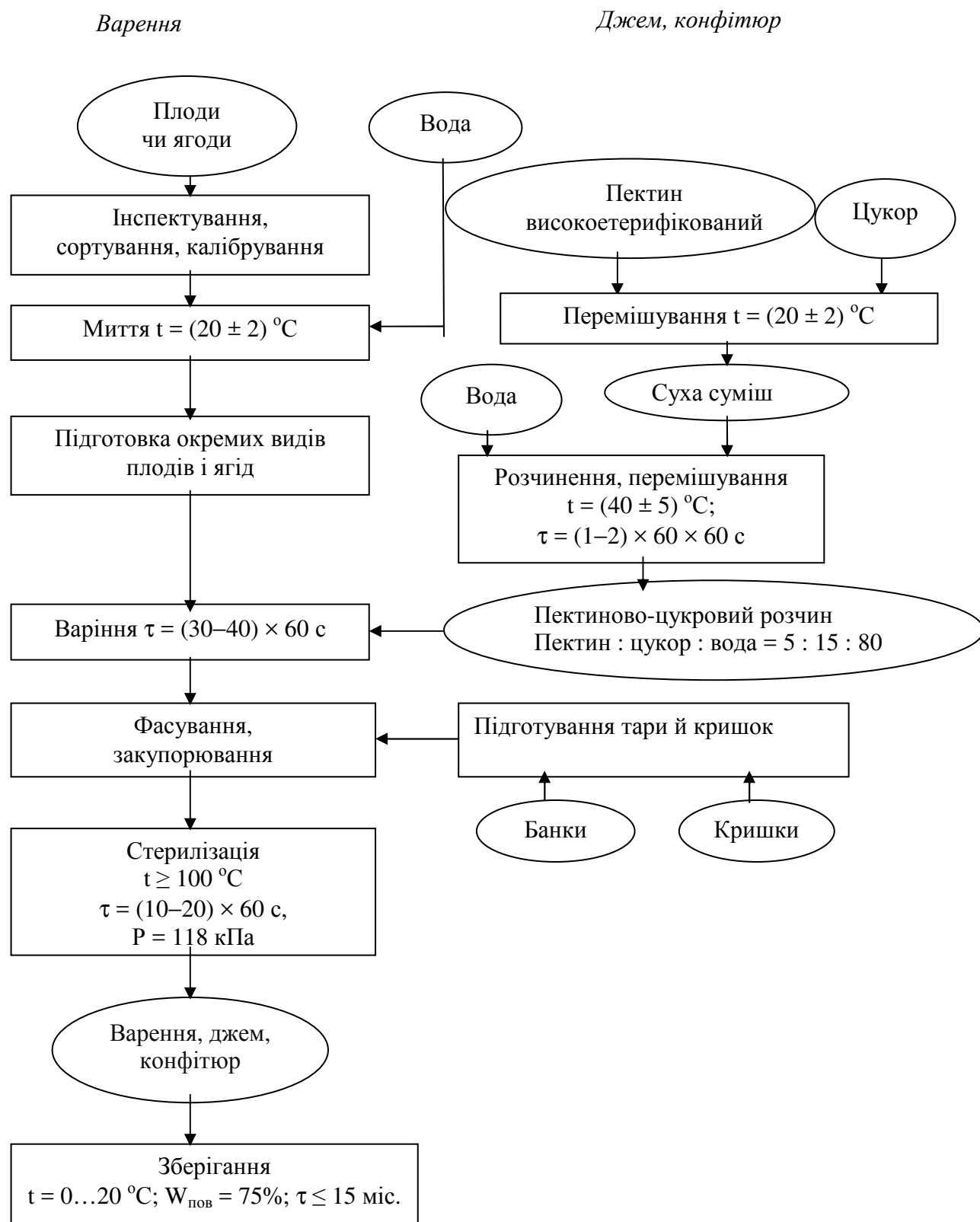
Рисунок 8.7 – Технологічна схема виробництва варення, джему та конфітюру
