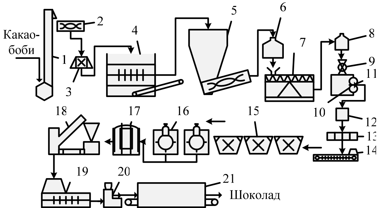
Рисунок А.1 – Апаратурно-технологічна схема шоколаду: 1 – норія ківшова; 2 – шнек; 3 – ваги; 4 – машина очищувально-сортувальна; 5 – сушарка; 6, 8 – бункери; 7 – машина дробильно-сортувальна; 9 – агрегат розмельний; 10 – збірник приймальний; 11 – насос шестеренний; 12 – збірник; 13 – дозатор; 14 – змішувач; 15 – млин; 16 – машина оздоблювальна; 17 – машина для конширування шоколаду; 18 – машина для темперування шоколаду; 19 – автомат формувальний; 20 – машина пакувальна; 21 – машина обандеролювальна
