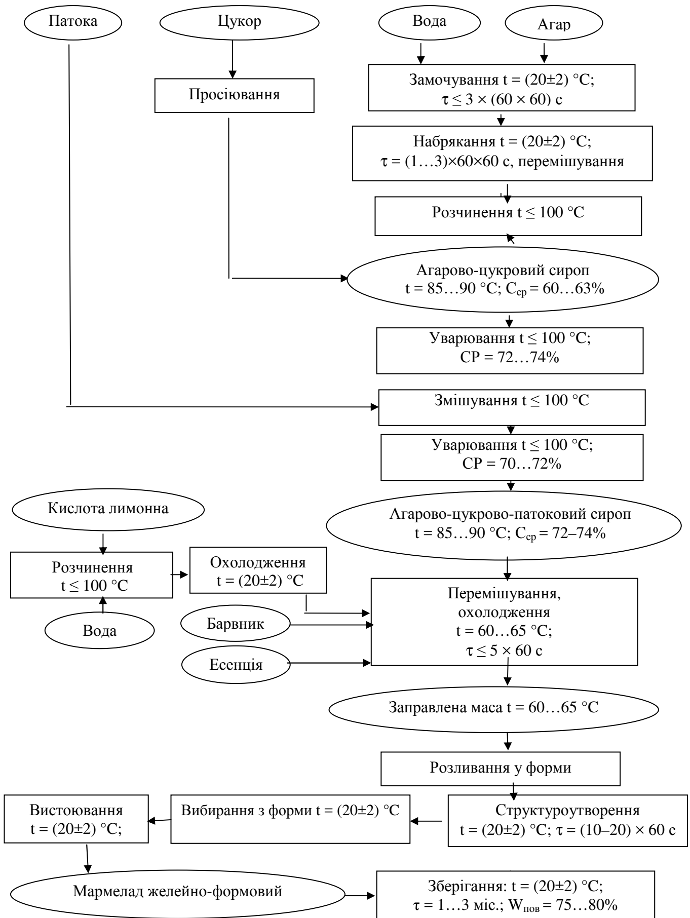
Рисунок 1.3 – Технологічна схема мармеладу желеино-формового на основі агару
