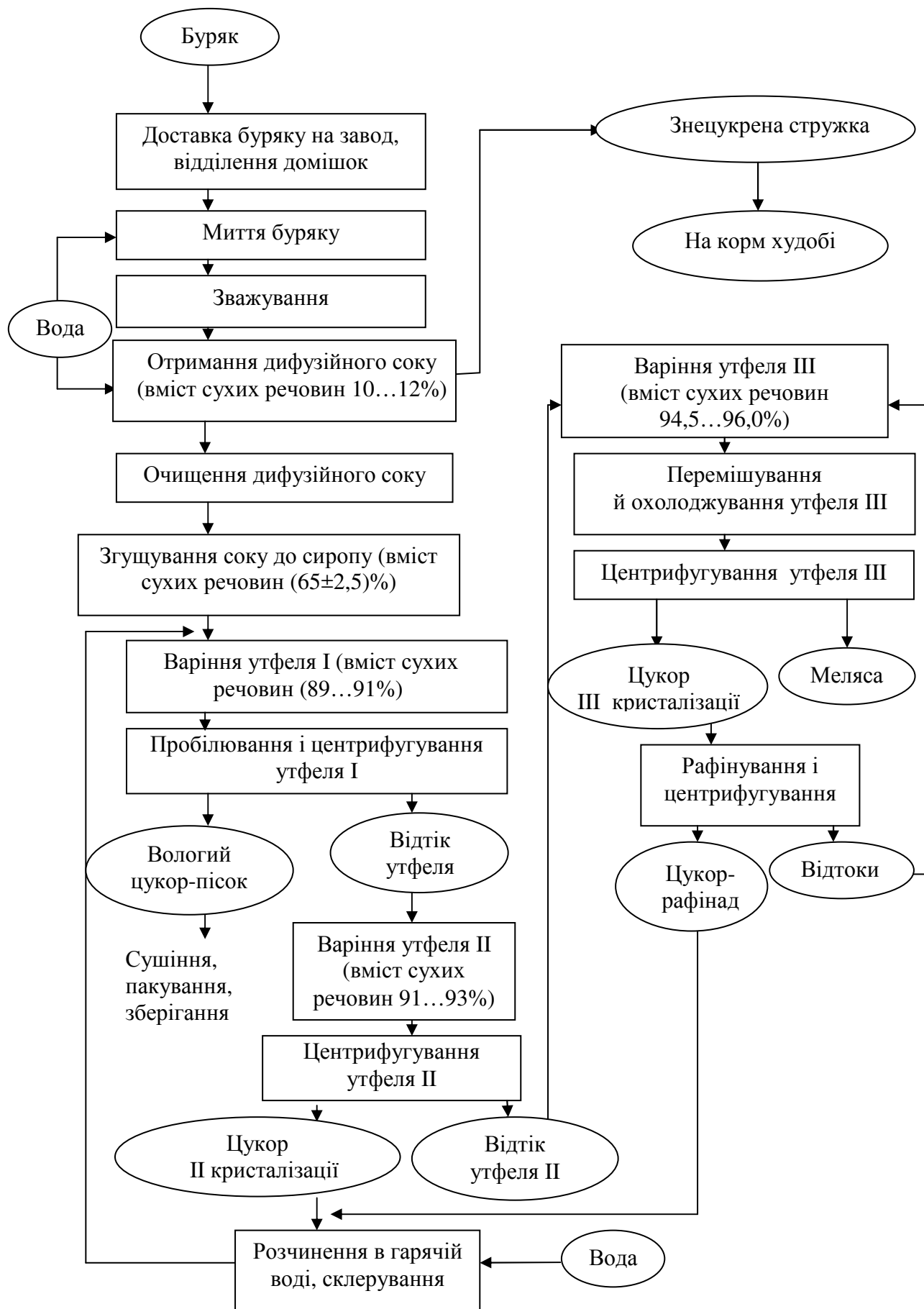
Рисунок 3.1 – Типова технологічна схема виробництва цукор-піску
