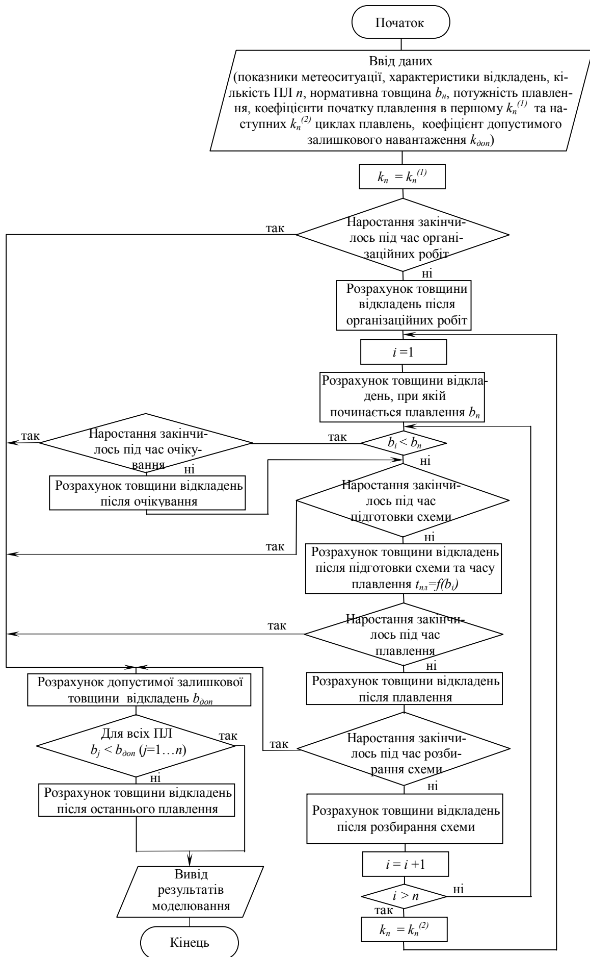
Рисунок 1 – Блок-схема алгоритму роботи імітаційної моделі плавлення ожеледі на групі взаємозв'язаних ПЛ 6–10 кВ ( i – номер лінії, на якій проводиться плавлення на даному етапі; b – товщина стінки відкладення).
