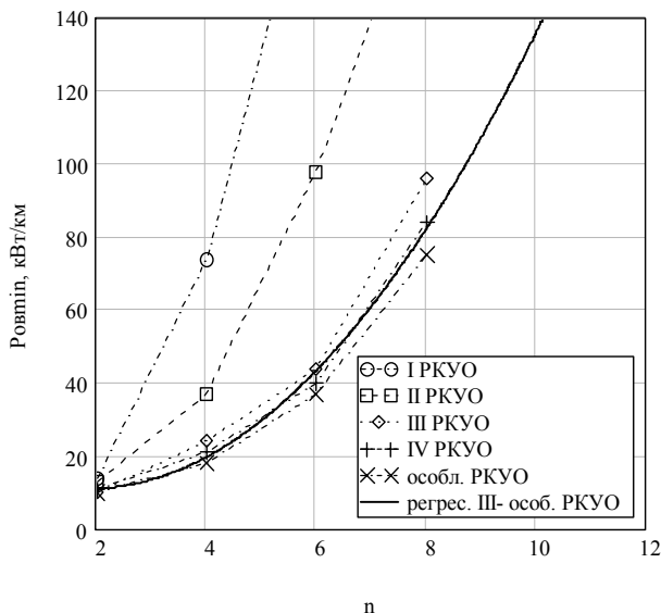
Рисунок 2 – Графіки залежностей P_{0e\min}=f(n) для різних РКУО.
