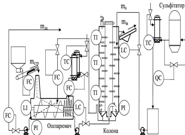
Рисунок 1 – Типова схема автоматизації дифузійної станції
