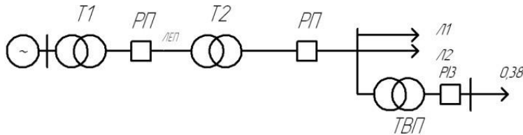
Рисунок 2 - Принципова схема місця установки лічильників обліку активної електричної енергії в двохелементній системі електропередавання: - система, в якій технологічний обсяг споживання електроенергії впливає на загальний небаланс
