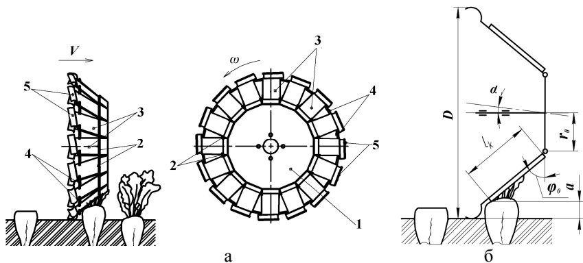
Рис. 1. Конструктивна (а) та кінематична (б) схеми нового копірно-роторного відокремлювача гички.
