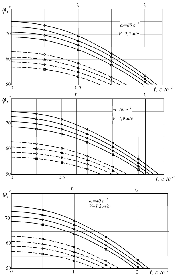
Рис. 5. Залежність кута відхилення робочого елемента від часу: \circ \triangle \diamond \square – відповідно кути відхилення останнього ріжучого та 1, 2, 3 наступних елементів системи; — кути відхилення робочих елементів у випадку взаємодії з коренеплодом h = 80 мм; - - кути відхилення робочих елементів у випадку взаємодії з коренеплодом h = 40 мм.
