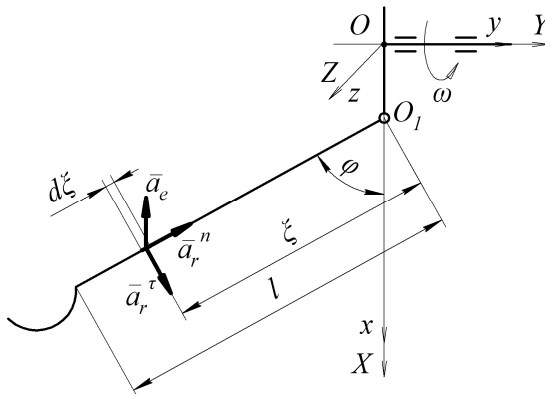
Рис. 2. Еквівалентна схема робочого органу.
