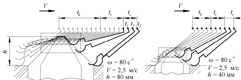
Рис. 6. Графічний аналіз копіювання головок коренеплодів робочими елементами копірно-роторного відокремлювача гички.
