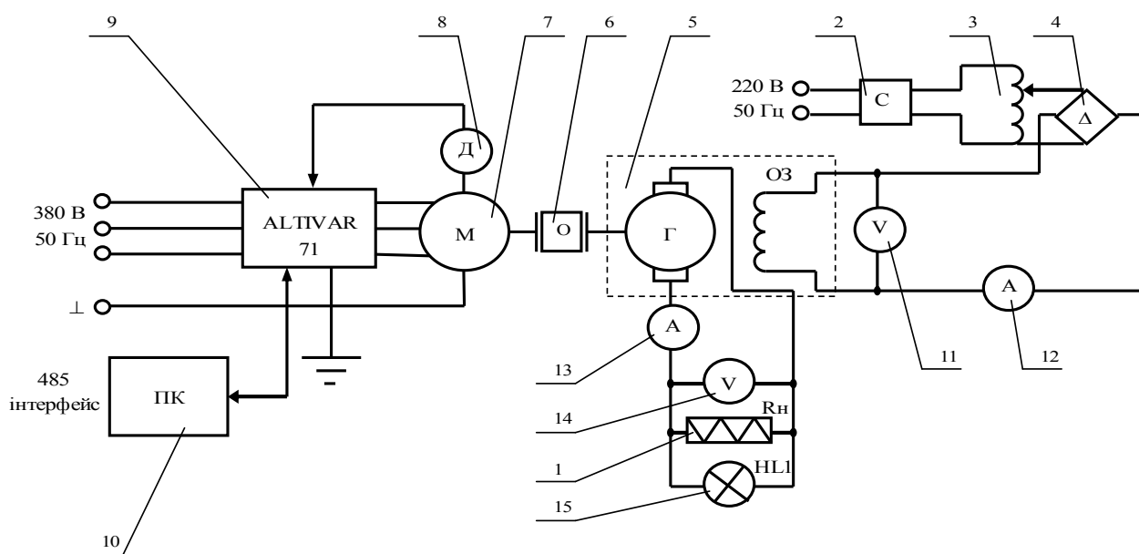
Рис. 2. Електрична схема стенду для дослідження механічних систем
