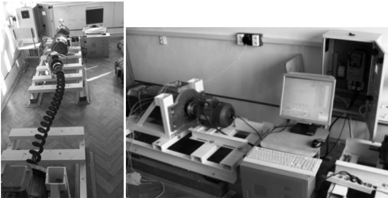
Рис. 3. Загальний вигляд стенду для дослідження механічних систем
