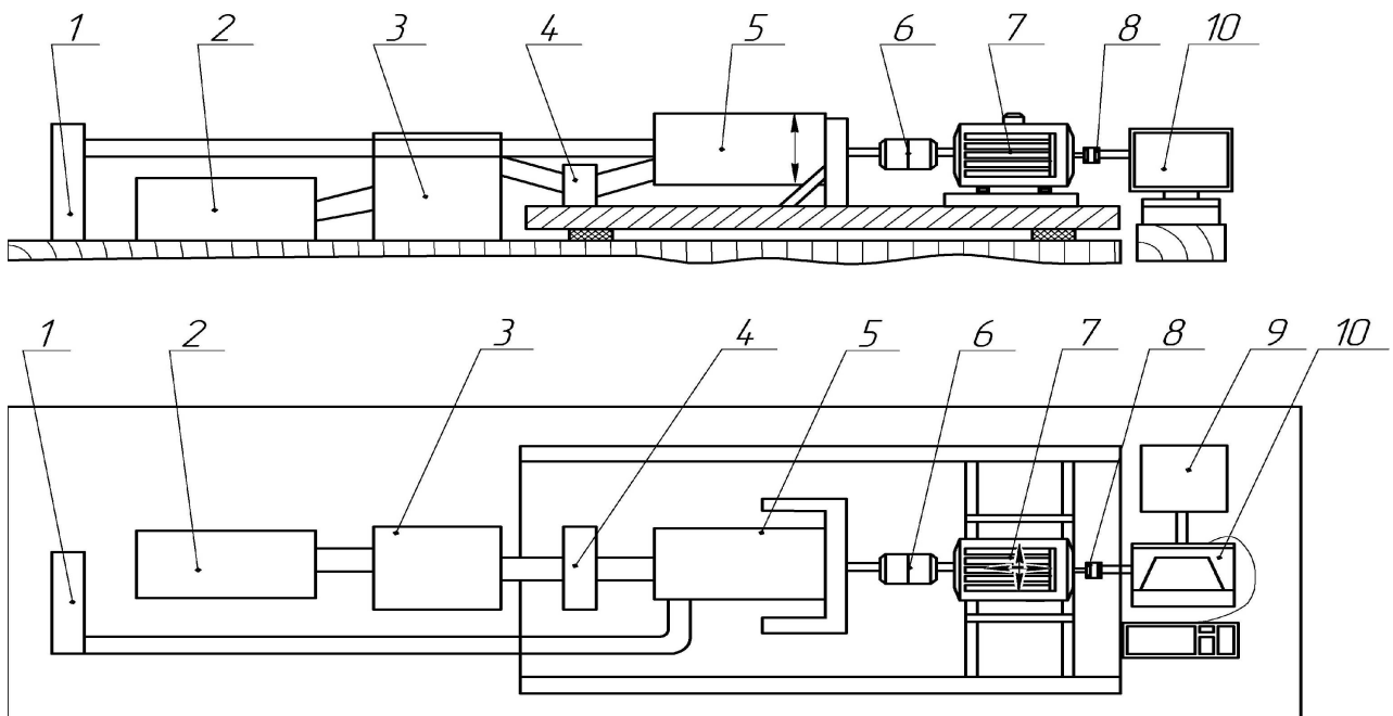
Рис. 1. Схема стенду для дослідження механічних систем
