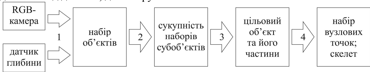
Рис. 2. Загальна структура алгоритму для ідентифікації об'єктів
