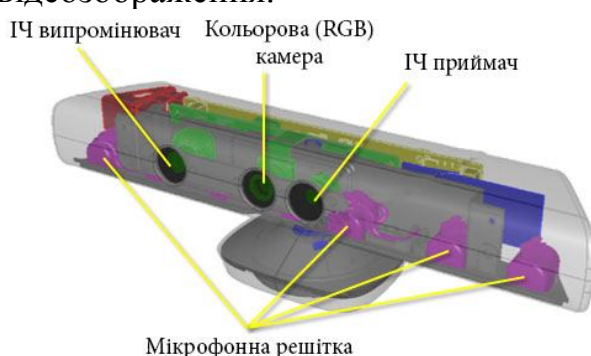
Рис. 1. Структура пристрою «Kinect»
