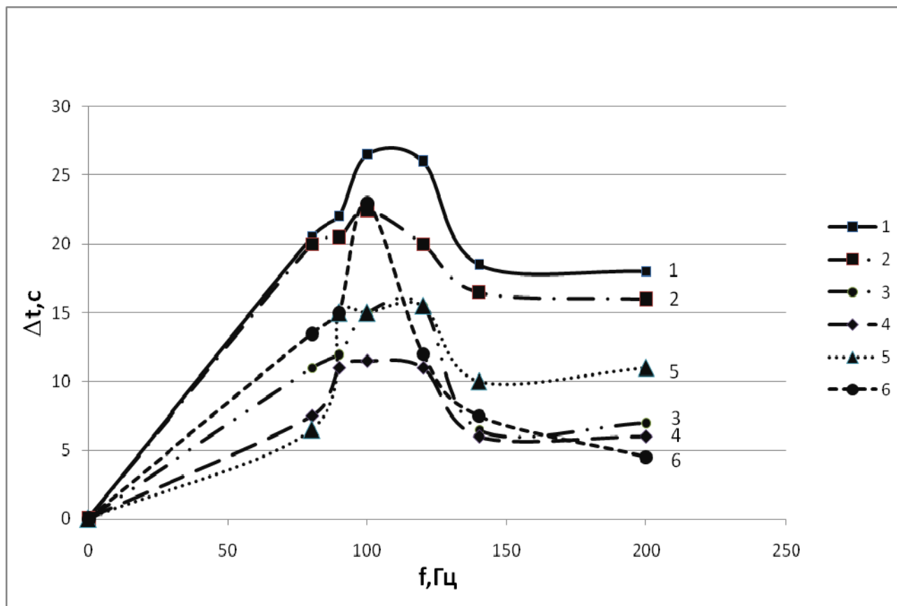
Рисунок 2 – Залежність скорочення часу нагрівання води від частоти імпульсів по варіантах спалювання пропану в повітрі порівняно з контролем
