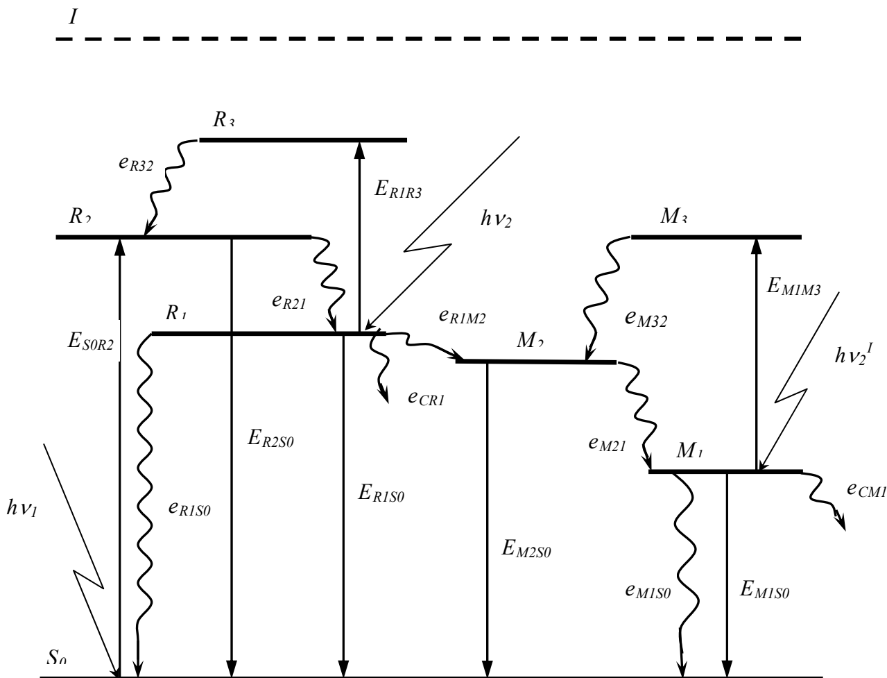
Рисунок 1 – Діаграма енергетичних рівнів та транспорту енергії в молекулі
