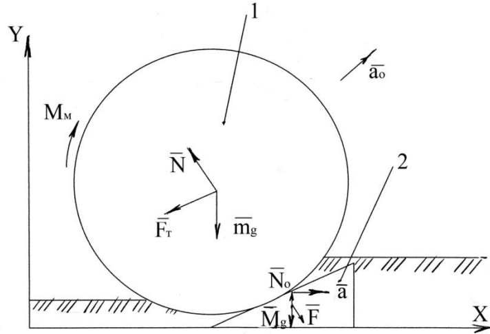
Рис 1 – Схема навантаження колеса у важких умовах експлуатації:
