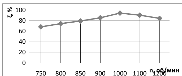
Рис.3 – Зависимость степени очистки зерна от частоты колебаний деки
