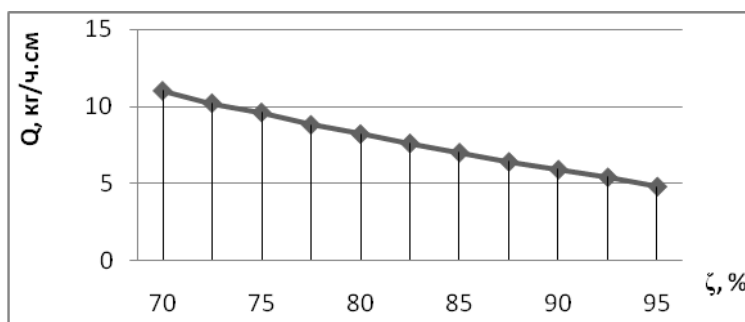
Рис. 4 – Зависимость степени очистки зерна от удельной производительности
