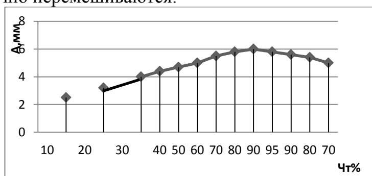
Рис.2 – Зависимость чистоты процесса сортирования зерновой массы от амплитуды колебаний деки
