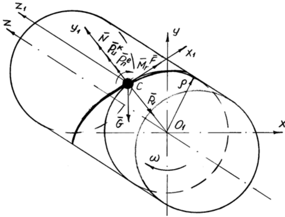
Рис.1 – Еквівалентна схема взаємодії бульби картоплі з поверхнею спірального сепаратора
