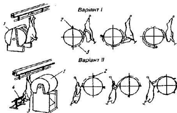
Рисунок 1.4 – Установка ФСБ для знімання шкур з туш ДРХ: 1 – барабан; 2 – палець; 3 – ланцюг; 4 – фіксатор
