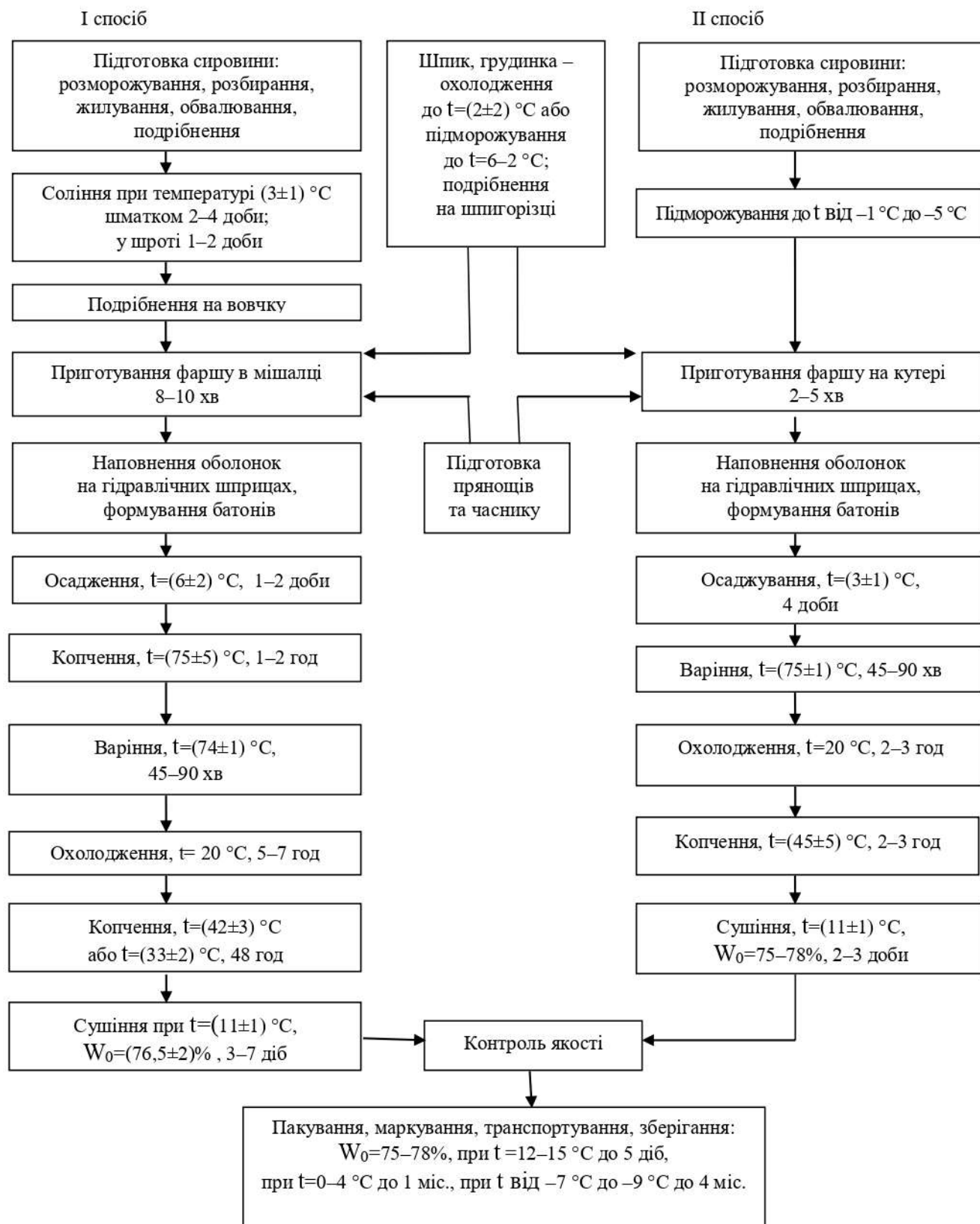
Рисунок 2.24 – Технологічна схема виробництва варено-копчених ковбас
