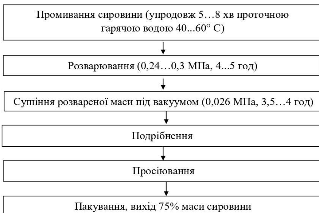
Рисунок 1.12 – Технологічний процес виробництва рого-копитного кормового борошна
