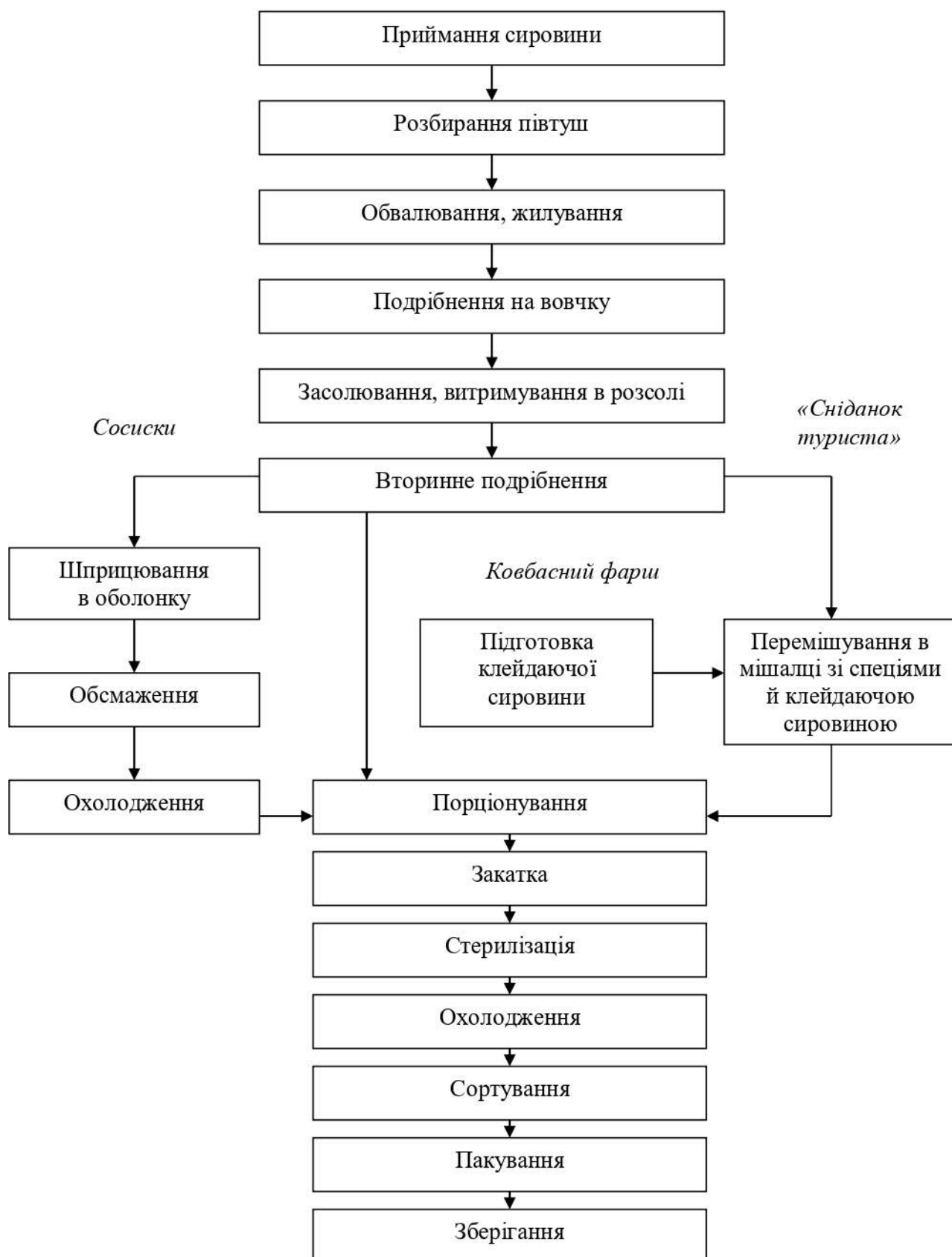
Рисунок 2.35 – Принципова технологічна схема виробництва фаршевих консервів та консервів із м'ясопродуктів
