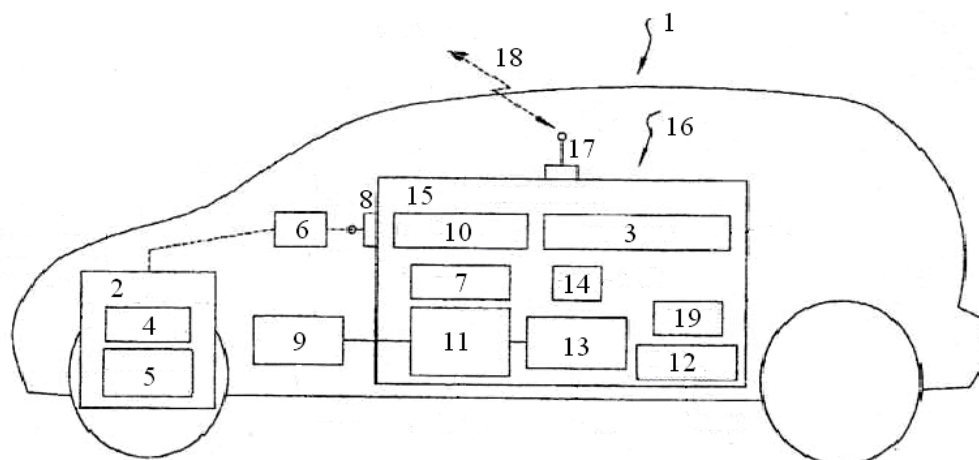
Рис. 10.7. Структурна схема системи телематики автомобіля
