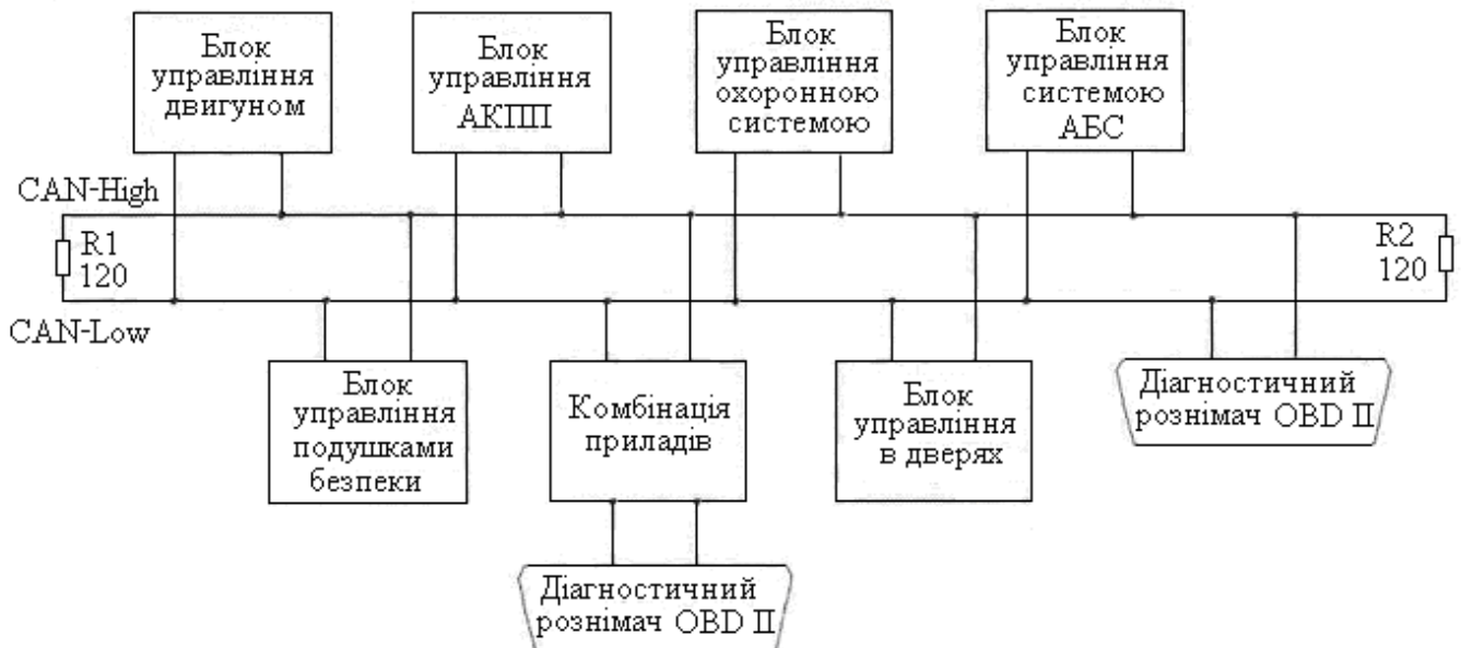
Рис. 7.3. Типова схема шини CAN
