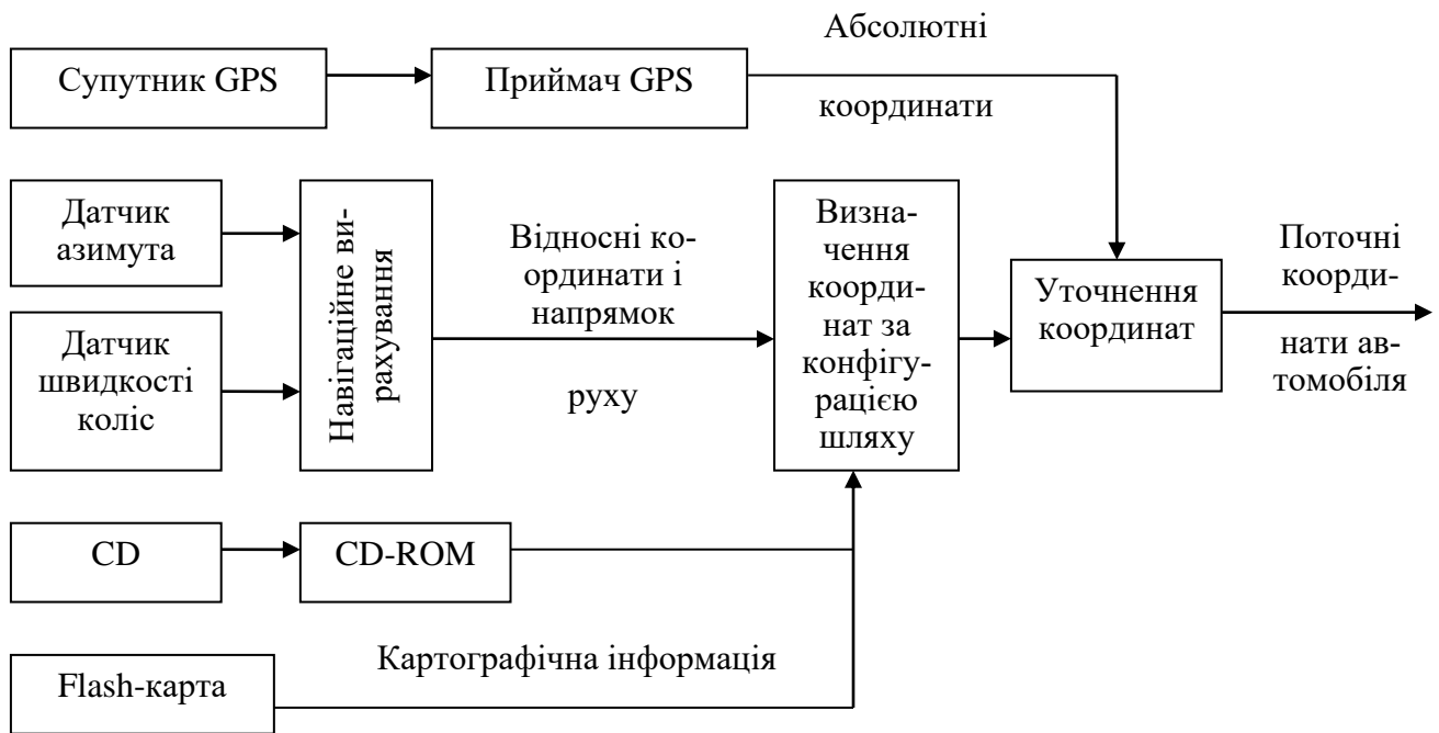
Рис. 5.7. Спрощена структура навігаційної системи
