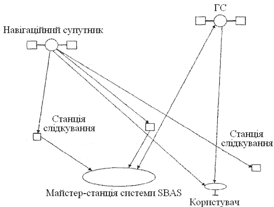
Рис. 5.5. Принцип дії системи SBAS
