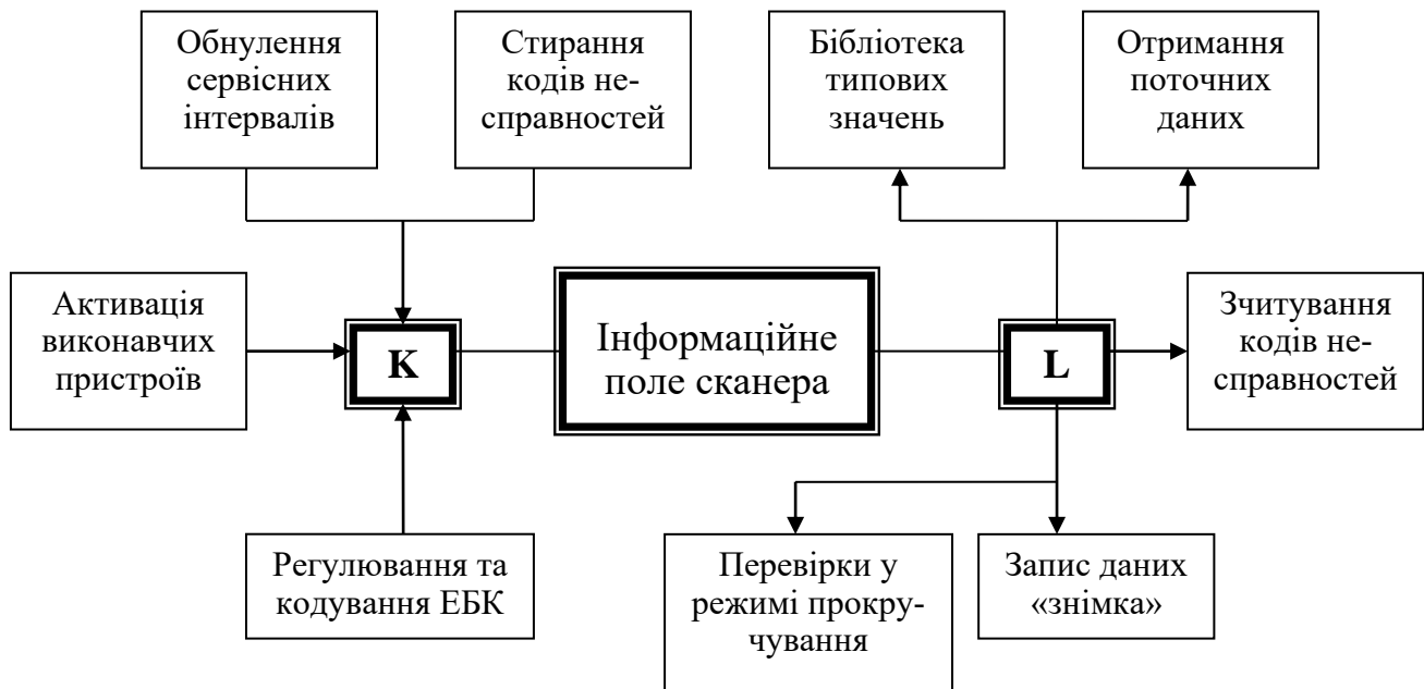
Рис. 7.13. Функціональні можливості сканера: К (control), L (line) – інформаційні канали
