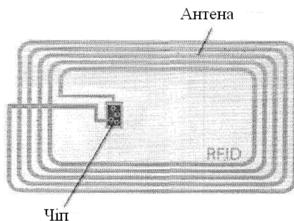
Рис. 6.2. Конструктивне виконання RFID-мітки
