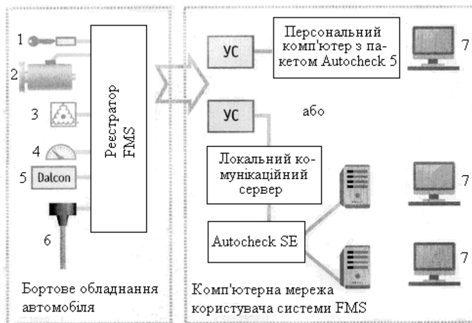
Рис. 10.24. Структурна схема системи FMS та взаємодія її елементів:
