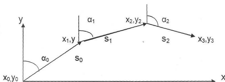
Рис. 5.12. Метод навігаційного вирахування шляху
