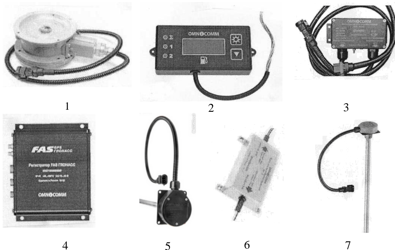
Рис. 10.22. Компоненти моніторингової системи Omnicomm:
