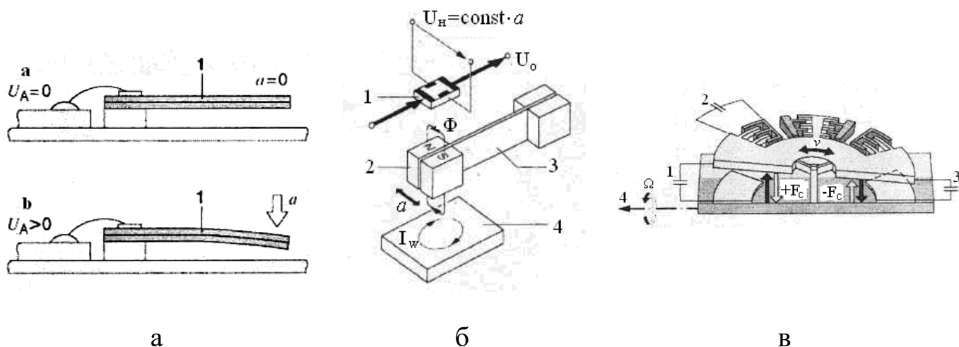
Рис. 8.6. Датчики зіткнення:
