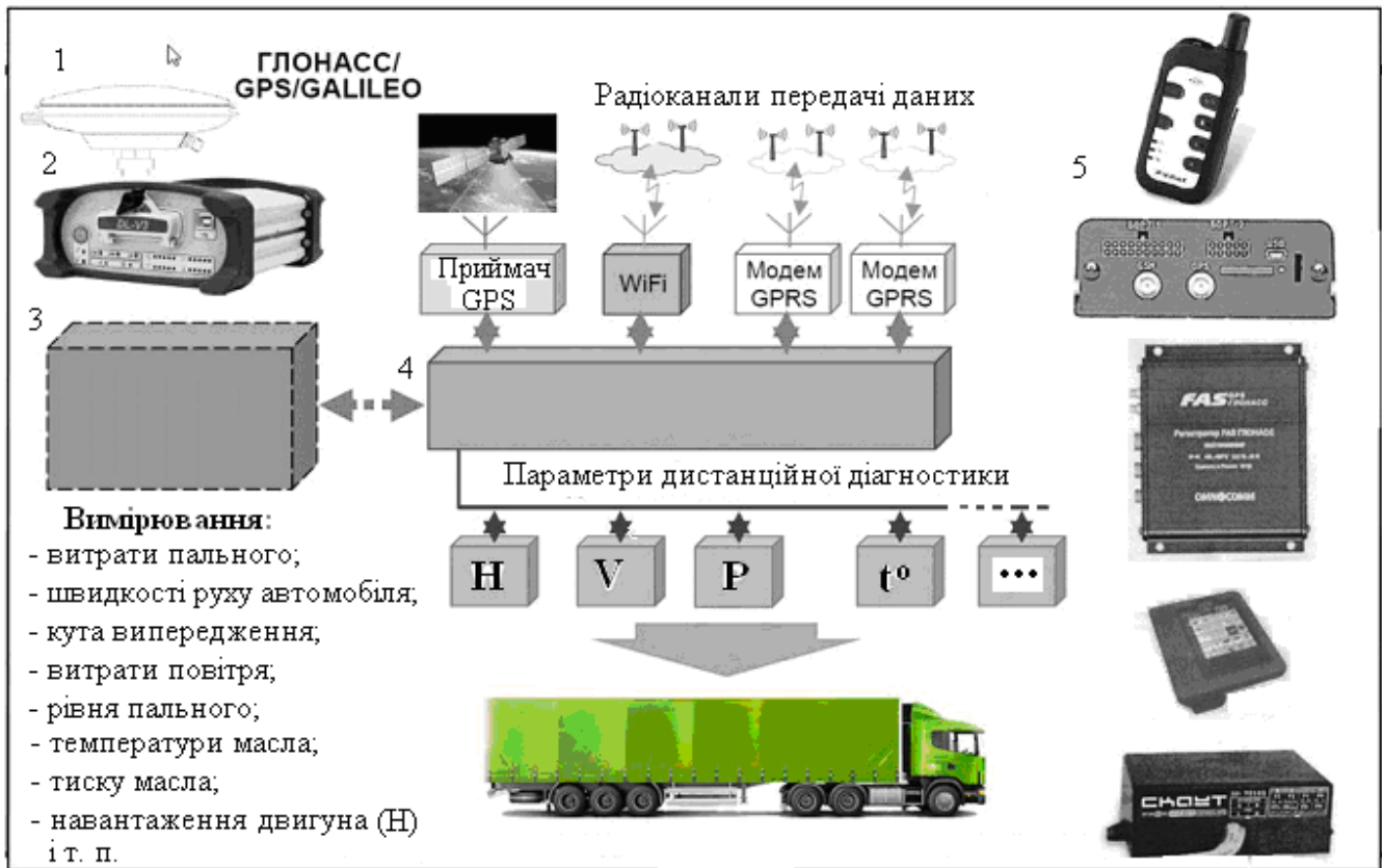
Рис. 7.20. Схема й обладнання системи дистанційної діагностики:
