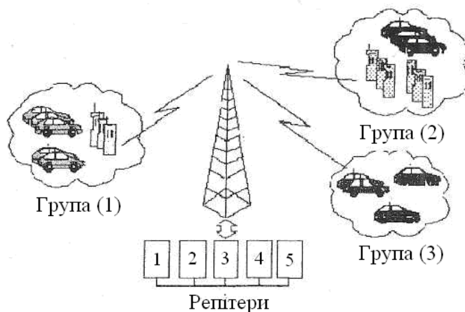
Рис. 6.21. Схема транкової мобільної радіосистеми
