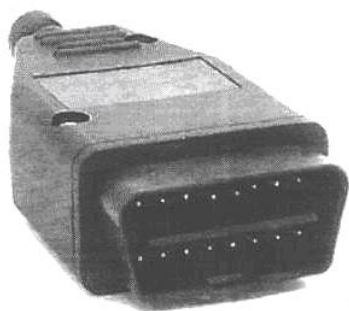
Рис. 7.15. Вигляд конектора діагностичного рознімача J1962 стандарту OBD-II
