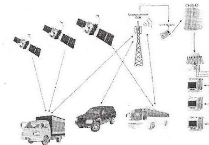
Рис. 10.14. Система моніторингу «ГЛОБУС»
