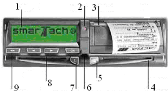
Рис. 6.12. Цифровий тахограф (а) та смарт-карти (б):
