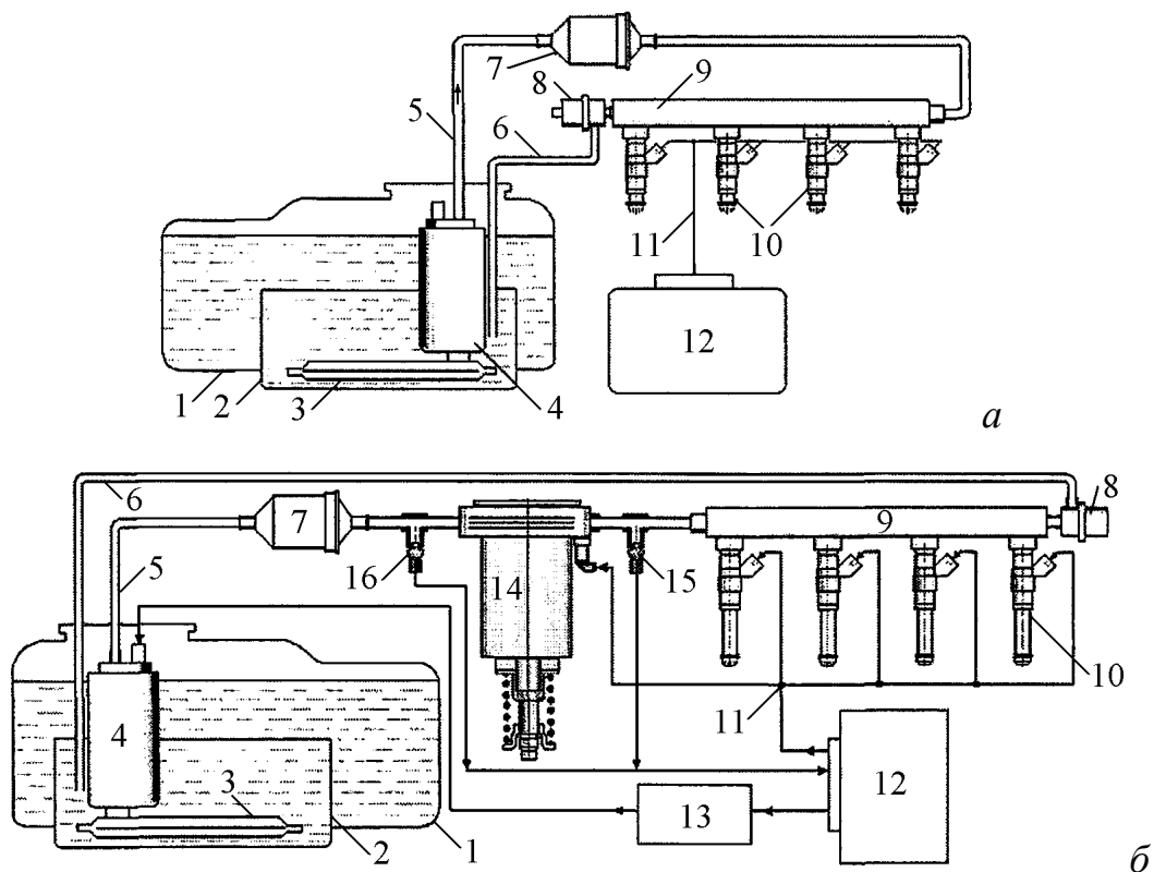
Рис. 9.13. Функціональні схеми систем упорскування бензину:
