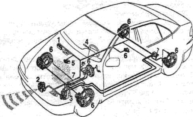
Рис. 8.1. Компоненти системи адаптивного круїз-контролю:
