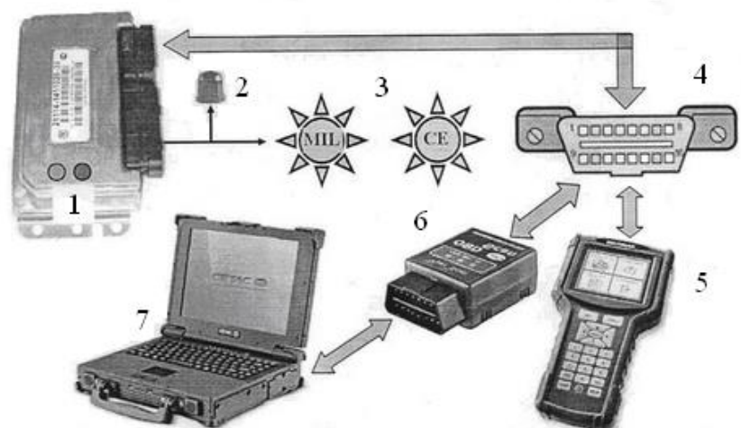
Рис. 7.13. Функціональні можливості сканера: К (control), L (line) – інформаційні канали
