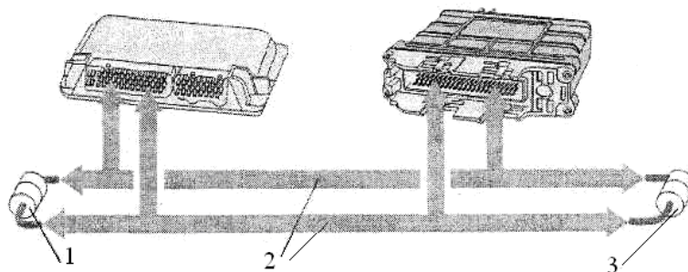
Рис. 7.7. Компоненти шини даних: 1 – термінал шини даних; 2 – провід шини даних; 3 – термінал шини даних
