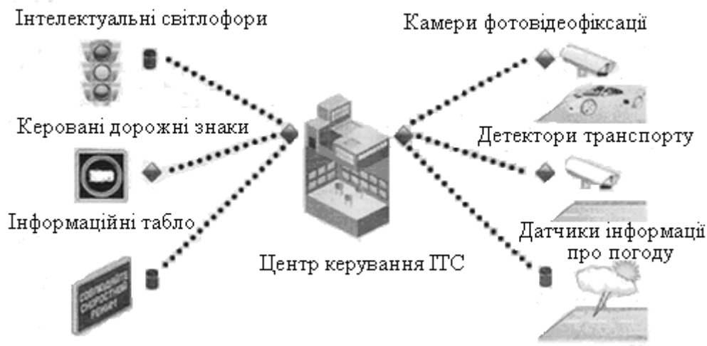
Рис. 3.5. Засоби інформаційного забезпечення контролю дорожніх умов
