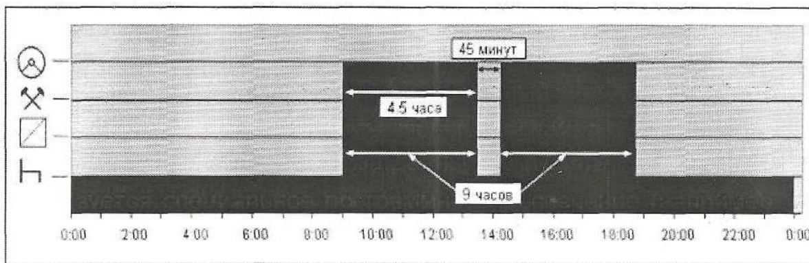
Рис. 6.18. Дані тахографа, представлені у вигляді гістограми
