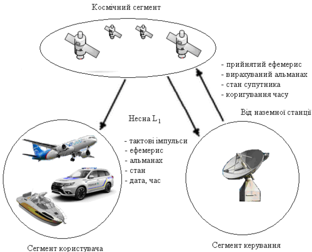
Рис. 5.3. Структура навігаційних повідомлень
