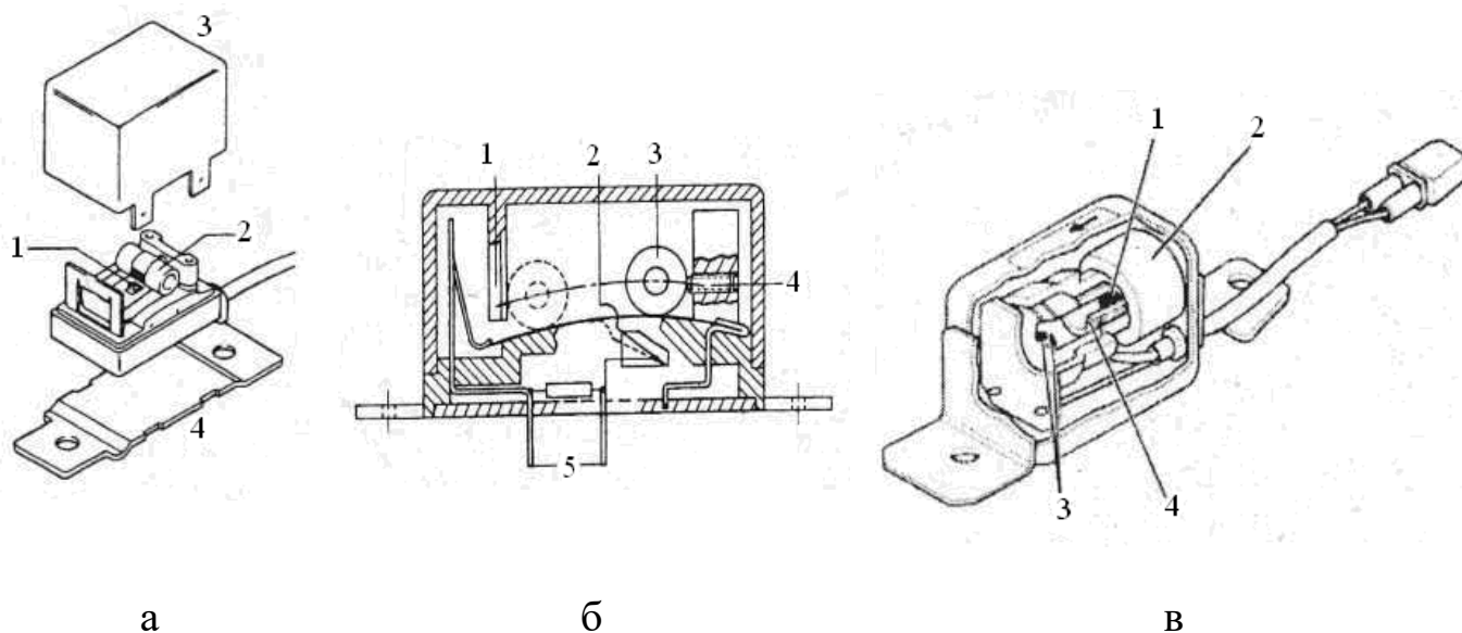
Рис. 8.7. Сенсори Crash:
