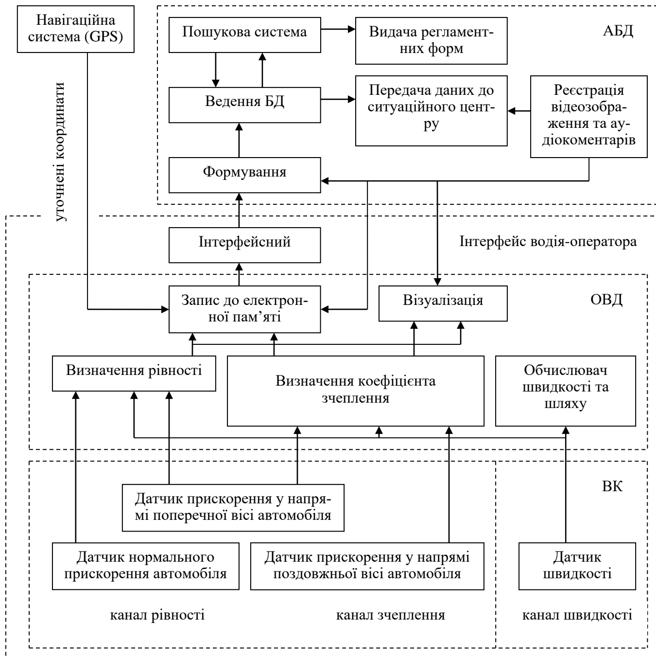
Рис. 3.3. Схема функціональна внутрішньої автомобільної телематичної системи
