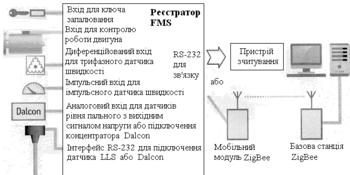
Рис. 10.23. Схема пристроїв реєстратора FMS
