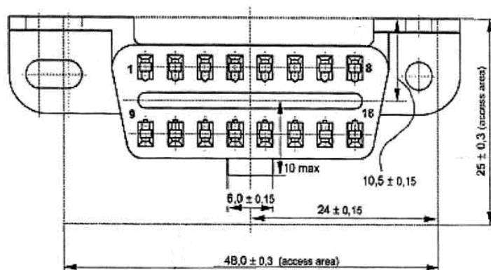
Рис. 7.16. Вигляд колодки діагностичного рознімача J1962 стандарту OBD-II
