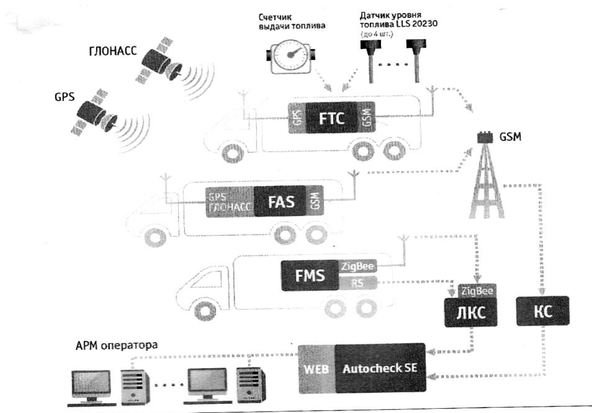
Рис. 10.21. Схема взаємодії систем FTC, FAS та FMS
