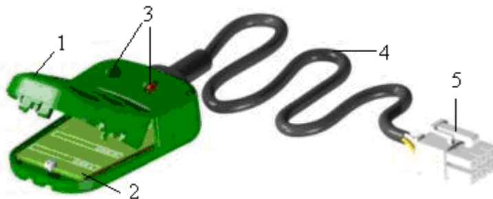
Рис. 7.9. Безконтактний пристрій CANCrocodile
