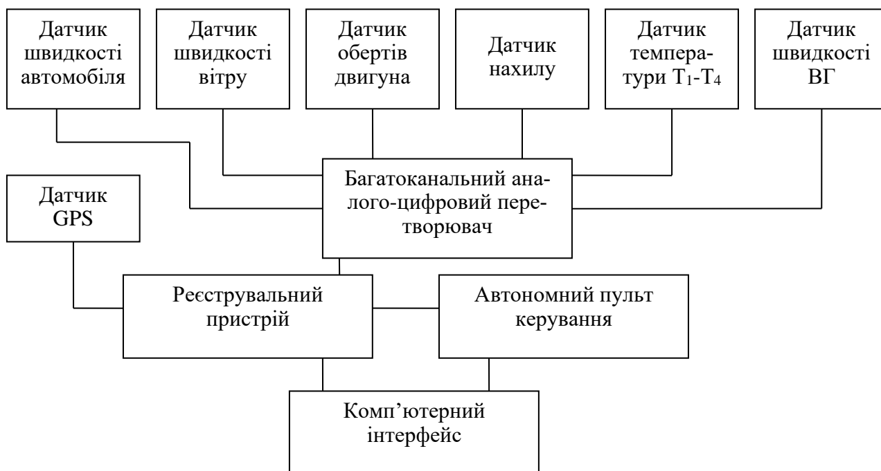
Рис. 5.16. Структурна схема системи моніторингу
