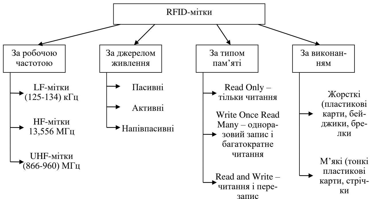
Рис. 6.3. Класифікація RFID-міток
