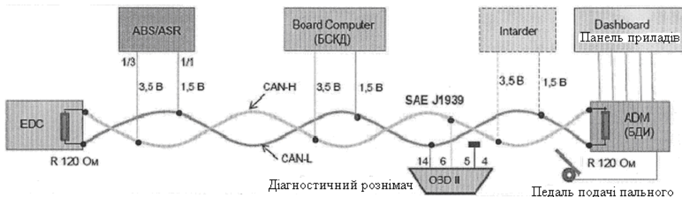
Рис. 7.2. Підключення пристроїв до шини CAN
