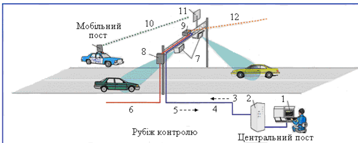
Рис. 4.19. Структурна схема автоматизованого комплексу «Кріс»:
