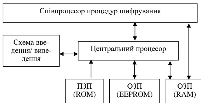
Рис. 6.14. Схема мікропроцесора смарт-карти
