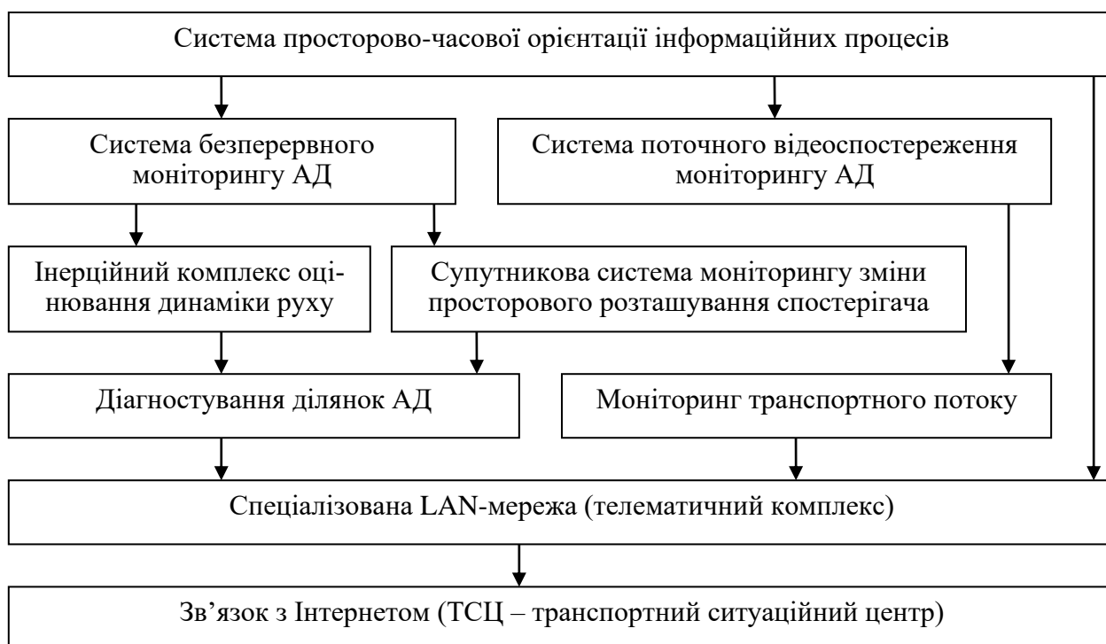
Рис. 3.2. Комплекс технічних засобів інтерактивного моніторингу АД
