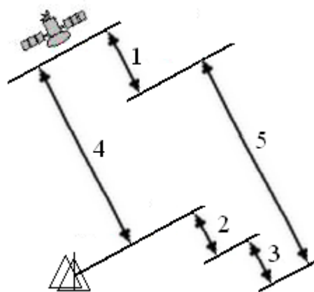
Рис. 5.17. Помилки у визначенні дальності:
