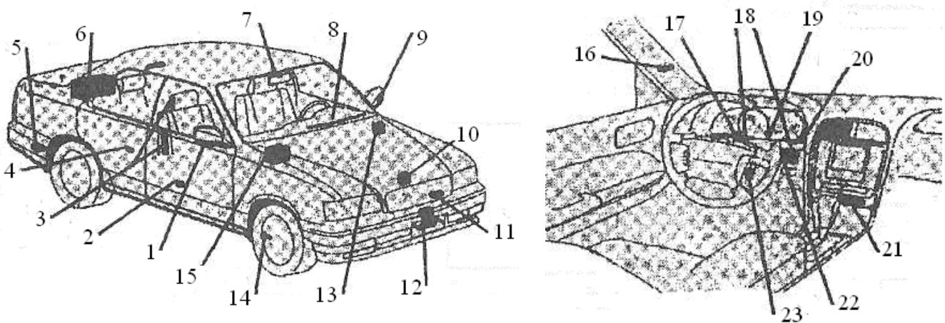
Рис. 9.5. Система датчиків та виконавчих пристроїв забезпечення безпеки автомобіля:
