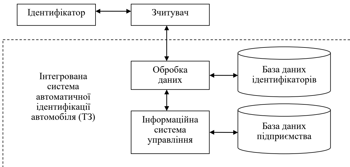
Рис. 4.14. Принципова схема роботи системи автоматичної ідентифікації автомобіля
