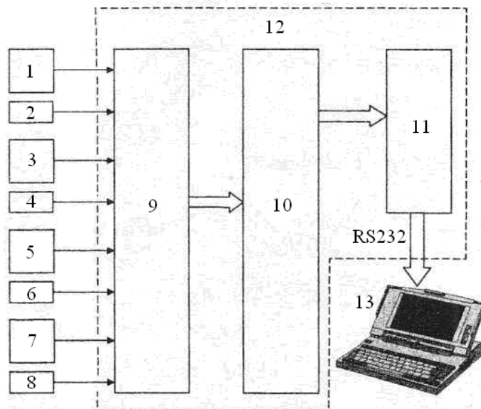
Рис. 10.2. Спрощена схема пристрою для моніторингу руху транспортних засобів:
