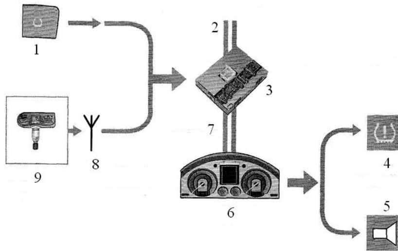
Рис. 8.15. Компоненти системи сигналізації та контролю тиску в шинах автомобілів Phaeton, Touareg і Passat:
