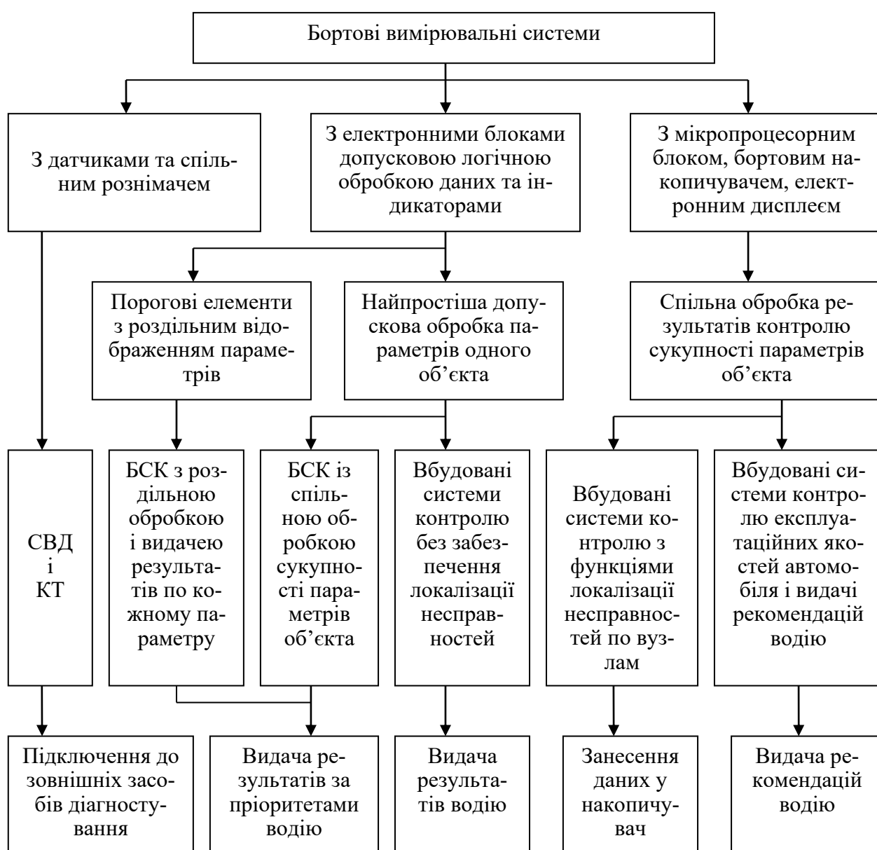
Рис. 7.10. Класифікація вбудованих засобів діагностування
