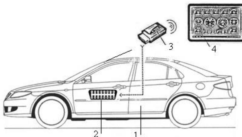
Рис. 10.12. Схема розташування гаджетів тестових систем з бездротовим пристроєм зв'язку на борту автомобіля:
