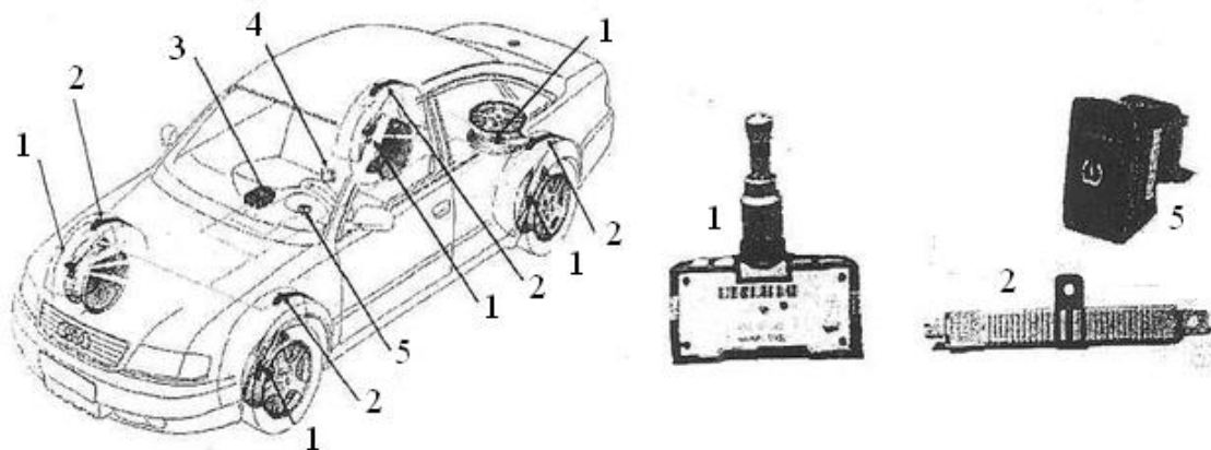
Рис. 8.14. Система контролю тиску в шинах TSS:
