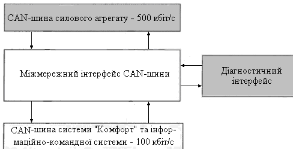
Рис. 7.6. Блок-схема міжмережного інтерфейсу
