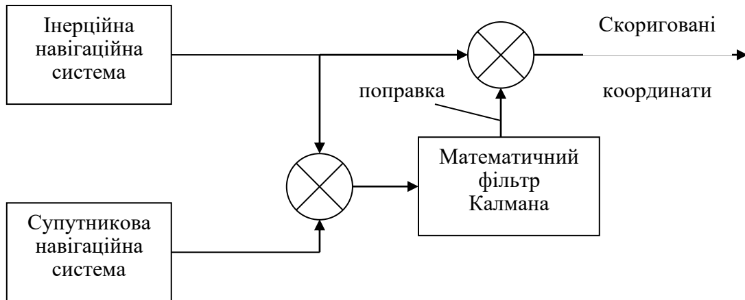
Рис. 5.13. Функціональна схема інтегрованої навігаційної системи
