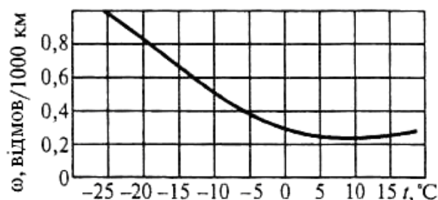
Рис. 2.3. Вплив температури навколишнього повітря на зміну загальної кількості відмов автомобілів (за даними НІІАТ)
