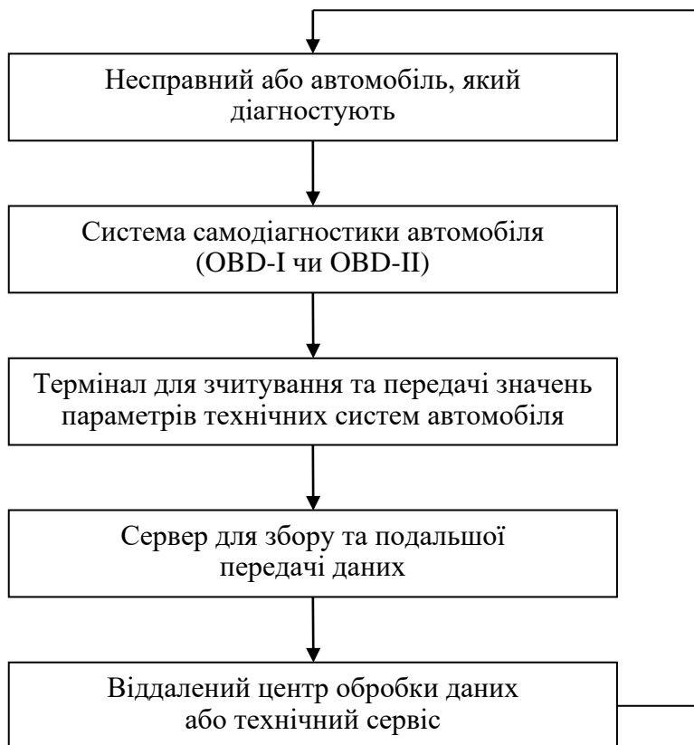
Рис. 7.18. Схема взаємодії елементів сервісу дистанційного діагностування автомобілів
