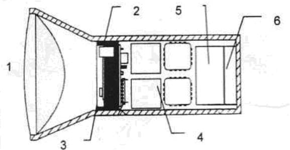
Рис. 8.2. Датчик швидкості:
