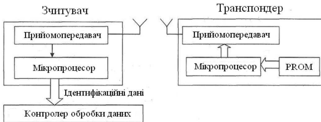
Рис. 6.1. Принцип дії RFID-системи
