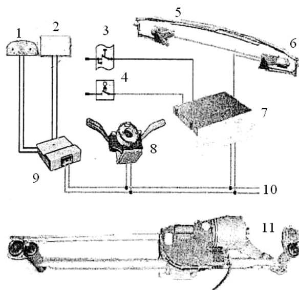
Рис. 8.17. Схема системи склоочисників на прикладі VW Touran/Golf V:
