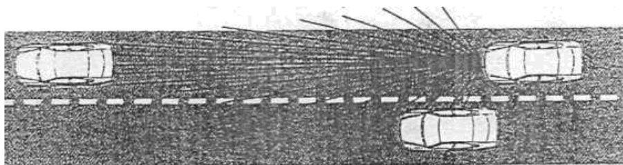
Рис. 8.4. Зони огляду сканера Alasca XT при його використанні в системі активного круїз контролю, здатного працювати в режимі «Старт-стоп»
