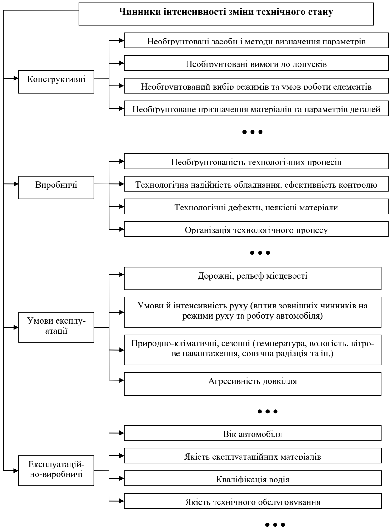
Рис. 2.8. Класифікація чинників впливу на інтенсивність зміни технічного стану автомобілів
