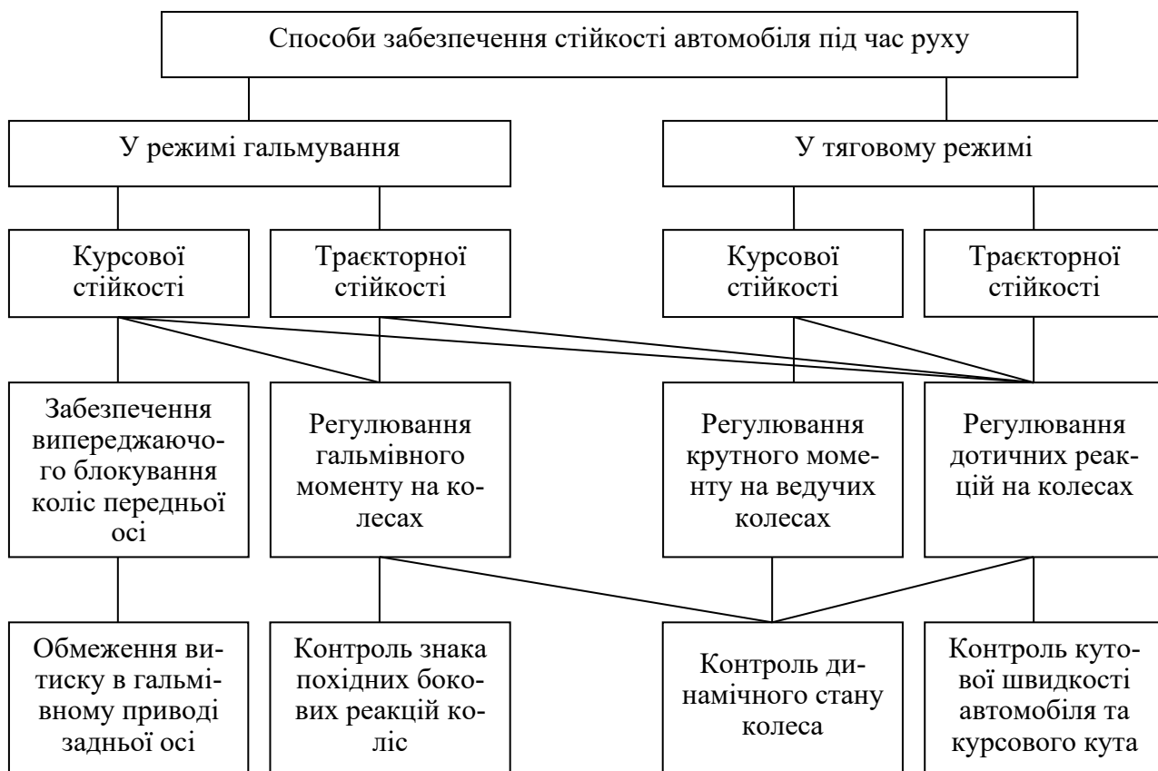
Рис. 9.2. Способи забезпечення стійкості автомобіля під час руху
