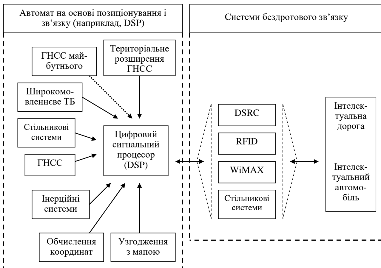
Рис. 4.3. Технології побудови навігаційних додатків ІТС:
