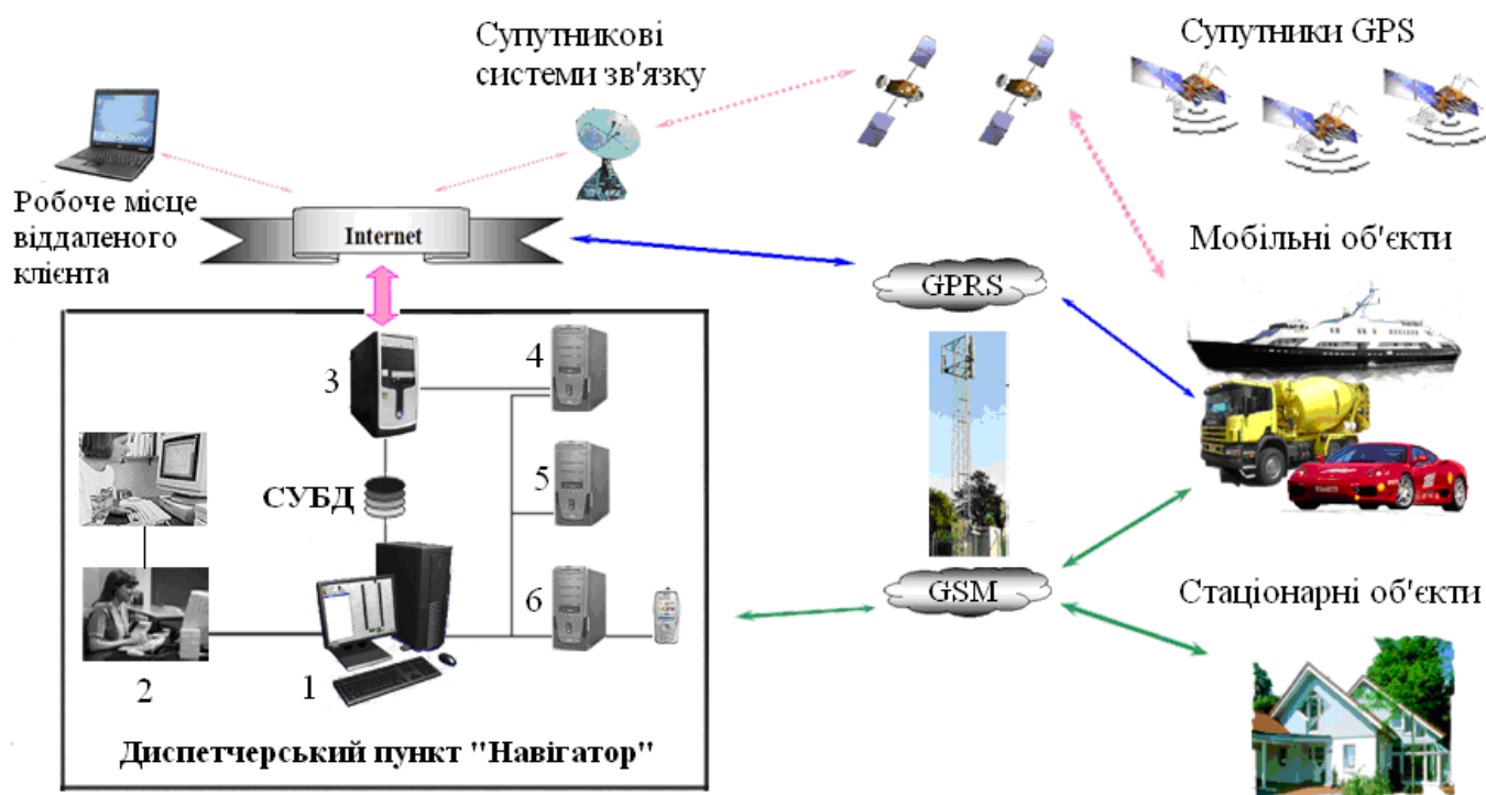
Рис. 6.24. Схема регіонального центра моніторингу мобільних об'єктів:
