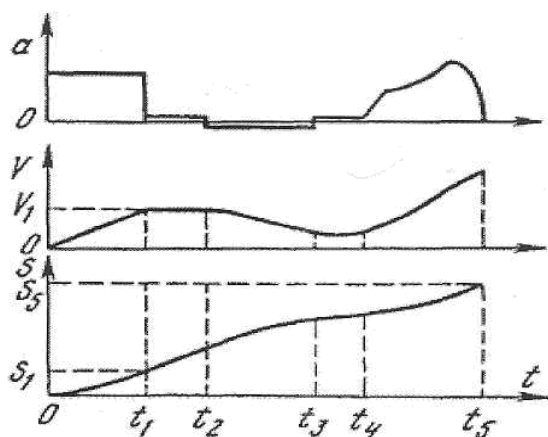
Рис. 5.14. Графіки зміни прискорення ( a ), швидкості ( V ), пройденого шляху ( S )
