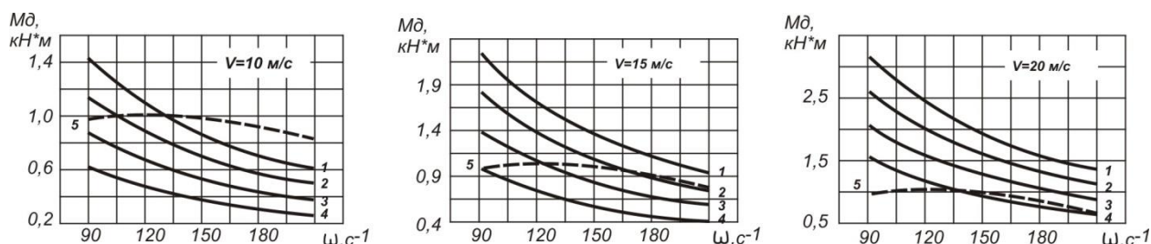
Рисунок 1 – Потужнісні параметри двигуна, які забезпечують рух автомобіля типу КрАЗ у різних дорожніх умовах
