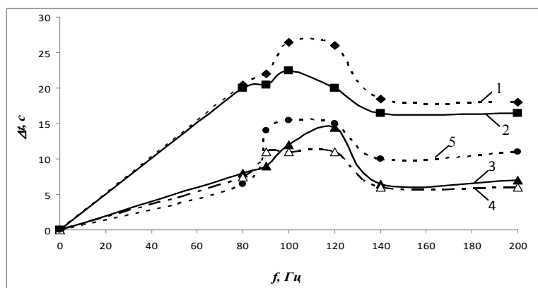
Рисунок 2 - Залежність зменшення часу нагрівання води від частоти імпульсів для різних варіантів електроактивації пропану і повітря (експеримент 2): 1,2,3,4,5 – номери варіантів дослідів
