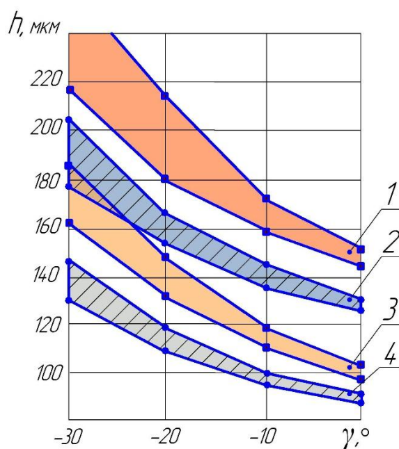
Рис. 1 – Вплив переднього кута \gamma під час чистового точіння:
