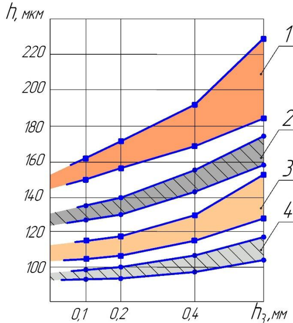
Рис. 2 – Вплив зносу різця h_3 під час чистового точіння:
