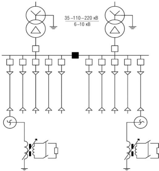
Рисунок 3.2 – Знижувальна під- станція із зазем- леною через дуго- гасний реактор ней- траллю на стороні 6- 10 кВ
