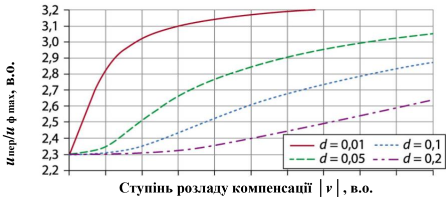
Рисунок 3.5 – Залежність перенапруг при дугових замиканнях на землю від ступеня розладу компенсації \nu за різних значень коефіцієнта демпфування d
