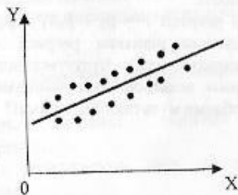
Рис 7.1. Гомоскедастичність
