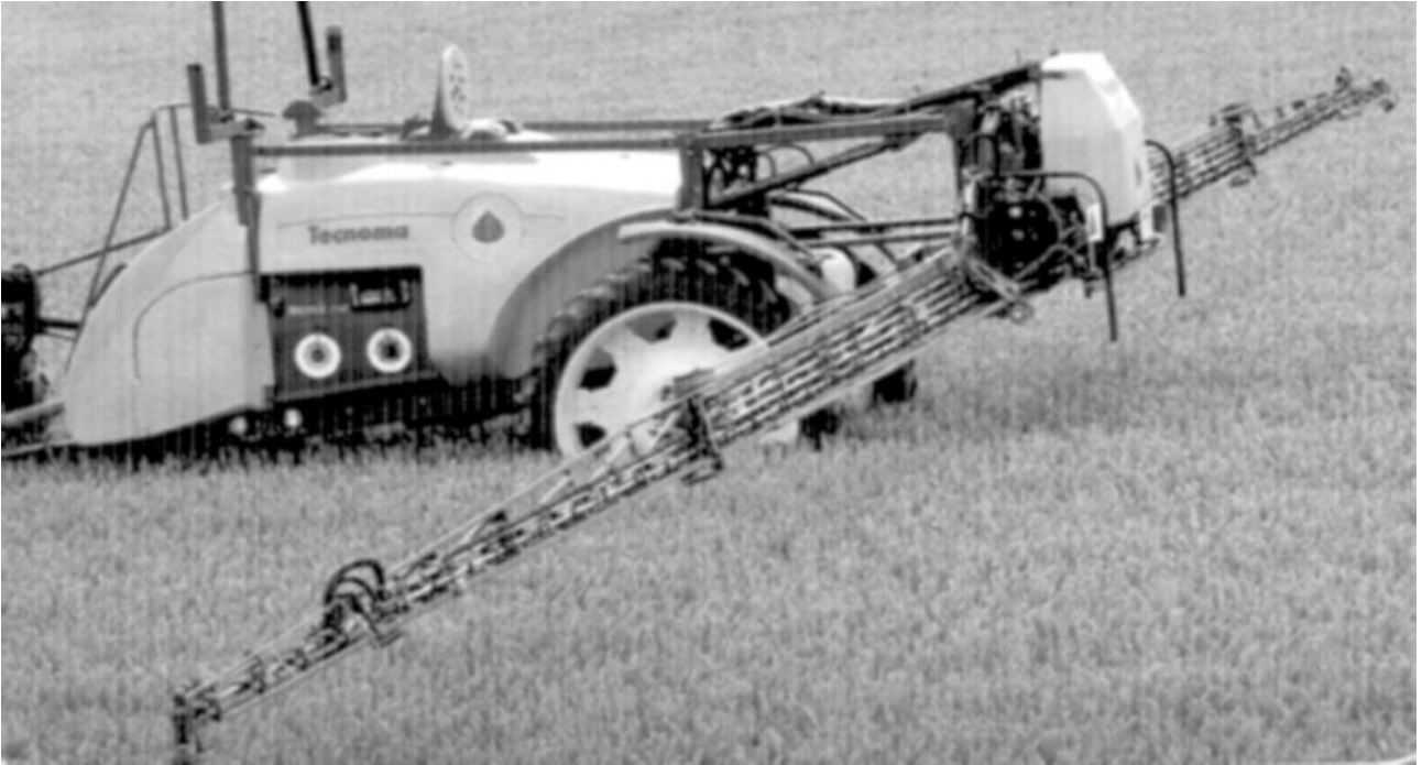
Рис. 96. Причіпний обприскувач TECNIS Об'єм бака робочої рідини 3100 л.+5 % Ширина захвату штанг 24, 28 м Необхідна потужність трактора 80–100 к. с.
