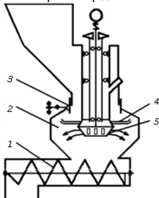
Рис. 70. Камера протруювання з дозатором насіння:
