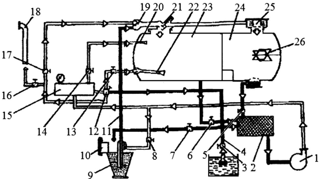
Рис. 112. Технологічна схема агрегату АПЖ-12:
