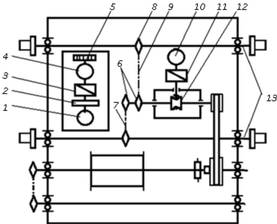
Рис. 84. Кінематична схема обприскувача ТОМ-1:
