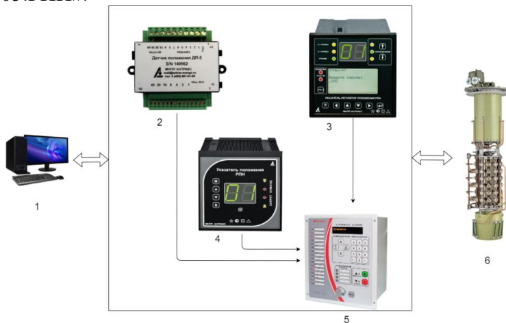
Рис. 1 – Структура випробувальної системи «Релсіс РЗЛ-05.РПН»: 1 – ПК; 2 – датчик положення привода ДП 5; 3 – показчик регулятор положення РПН; 4 – показчик положення РПН; 5 – пристрій мікропроцесорний для автоматичного управління РПН трансформатора «Релсіс РЗЛ-05»; 6 – РПН трансформатор
