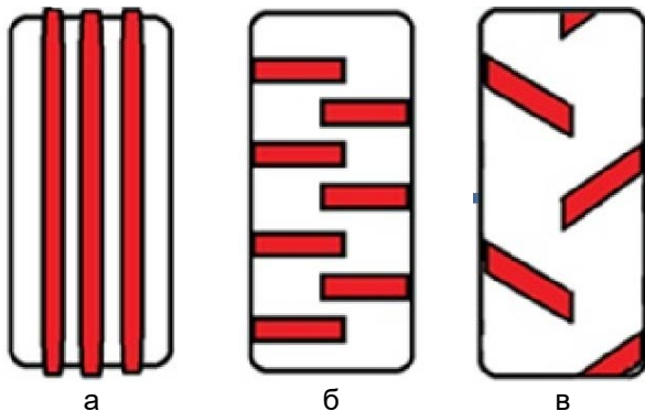
Рис. 3. Ґрунтозачепи нульовий кут (а), 90^\circ (б), комбінований (в)
