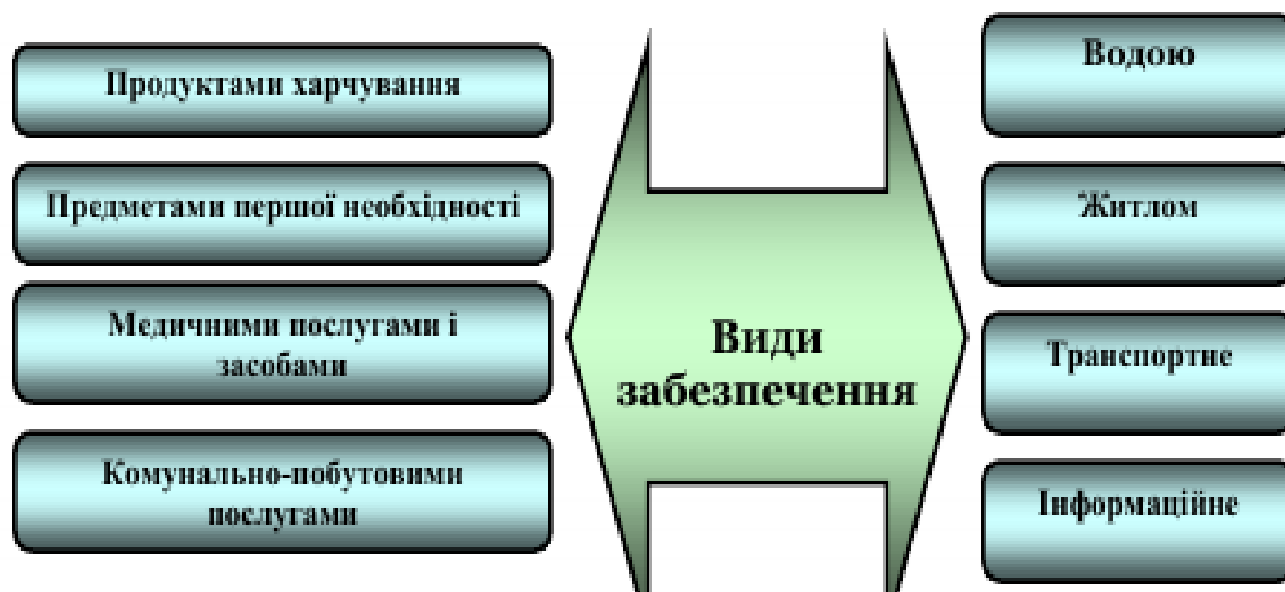
Рисунок 6.17 – Види забезпечення
