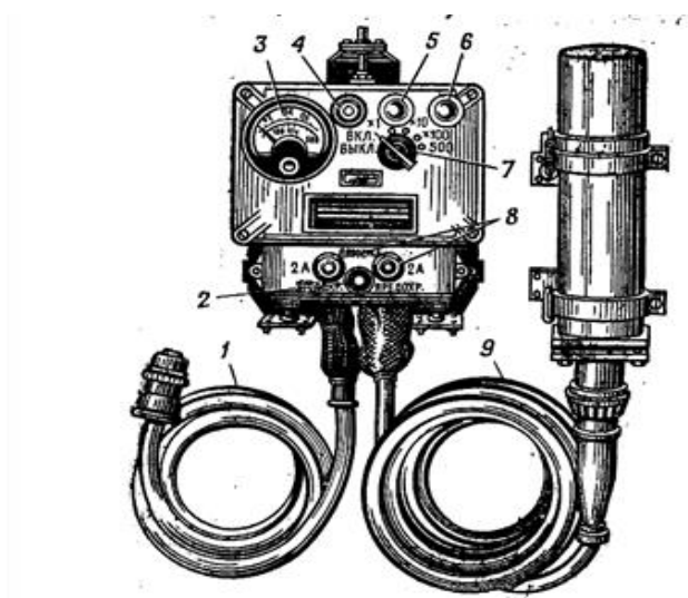
Рисунок 7.17 – Вимірювач потужності дози ДП-3Б:
