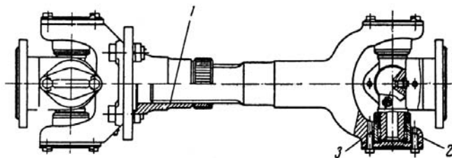
Рис. 3. Монтажные сопряжения деталей переднего карданного вала 125.36.011-2
