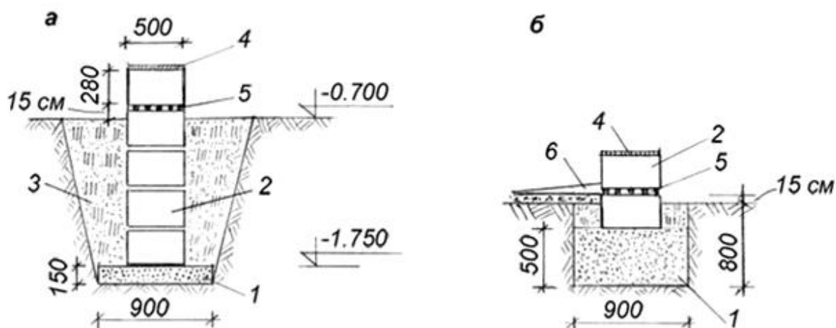
Рисунок 1 – Схема устрою збірного стовпчастого фундаменту:
