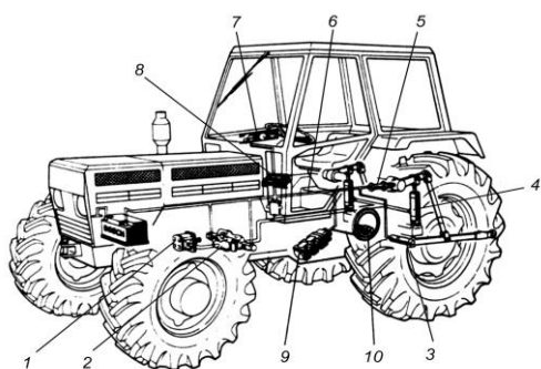
Рис. 1 – Розташування на тракторі компонентів ЕГСАР Hitch-Tronic: 1 – насос; 2 – регулятор системи; 3 – силовий датчик (другий не показаний); 4 – гідроциліндр начіпного пристрою; 5 – позиційний датчик; 6 – система кабелів для з'єднання компонентів ЕГСАР; 7 – панель керування системою; 8 – електронний блок керування ЕГСАР; 9 – радарний датчик; 10 – датчик швидкості обертання ведучих коліс
