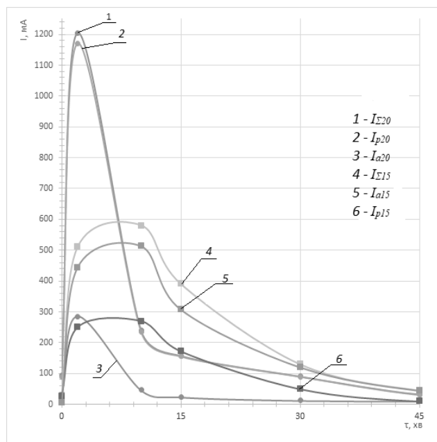
Рисунок 3 – Залежності струмів від зміни вологості в процесі сушіння абрикосу сорту "Любава" при: U_{EH} = 15 В, U_{EH} = 20 В, t_{н.с.} = 40 °C
