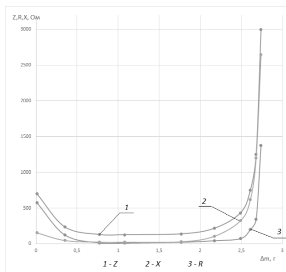
Рисунок 4 – Залежності опорів від зміни вологості в процесі сушіння абрикосу сорту "Любава" при: U_{EH} = 15 В, U_{EH} = 20 В, t_{н.с.} = 40 °C
