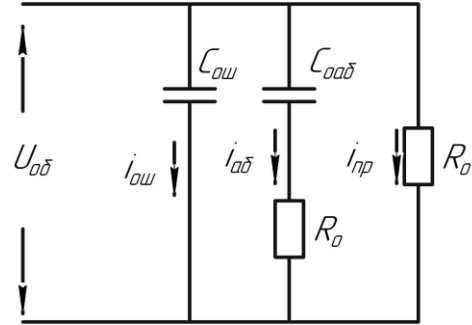
Рисунок 2 – Схема заміщення діелектрику (досліджуваного біоматеріалу)
